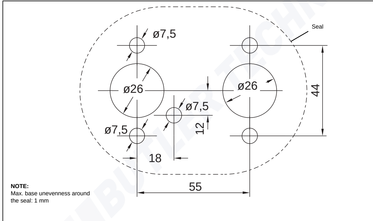
Fig. 37: Drilling template
