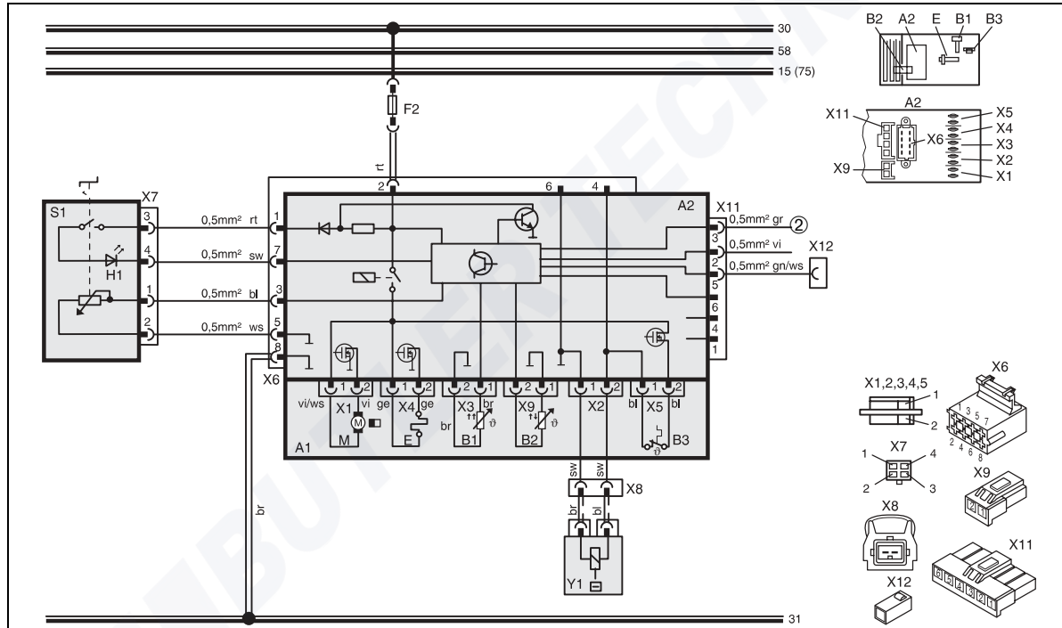
Bild 30: Automatikschaltplan Air Top 2000, 12V/24V mit Bedienelement, Legende siehe Seite 32 und 33
