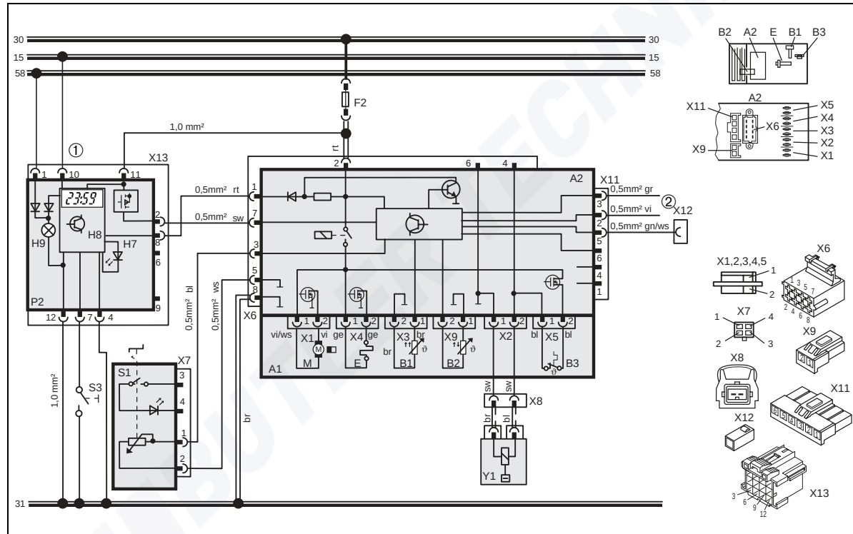
Bild 32: Automatikschaltplan Air Top 2000, 12V/24V mit Bedienelement und Kombiuhr, Legende siehe Seite 32 und 33
