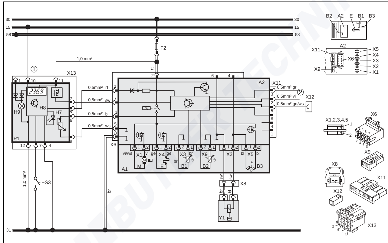
Fig. 31 Schéma électrique d'ensemble Air Top 2000, 12 V/24 V avec horloge polyvalente ; légende : voir pages 108 et 109
