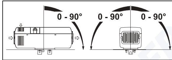
Bild 2: Empfohlene Einbaulagen Diesel Heizgeräte
