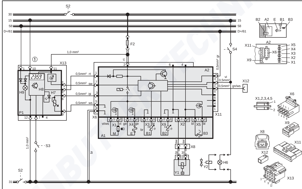
Bild 34: Automatikschaltplan Air Top 2000, 24V ADR-Betrieb mit Kombiuhr, Legende siehe Seite 32 und 33
