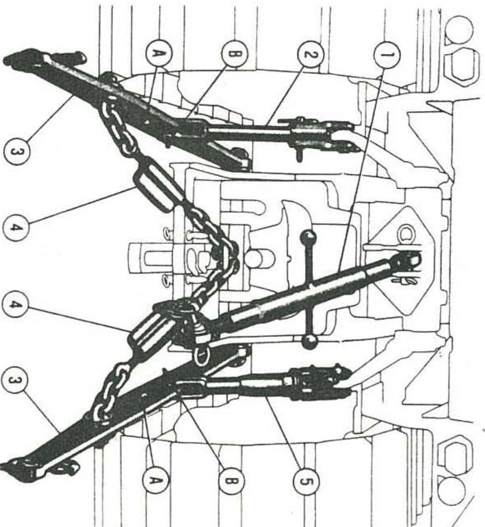
Fig. 10 - Dispositivo de levantamento hidráulico em 3 pontos.
