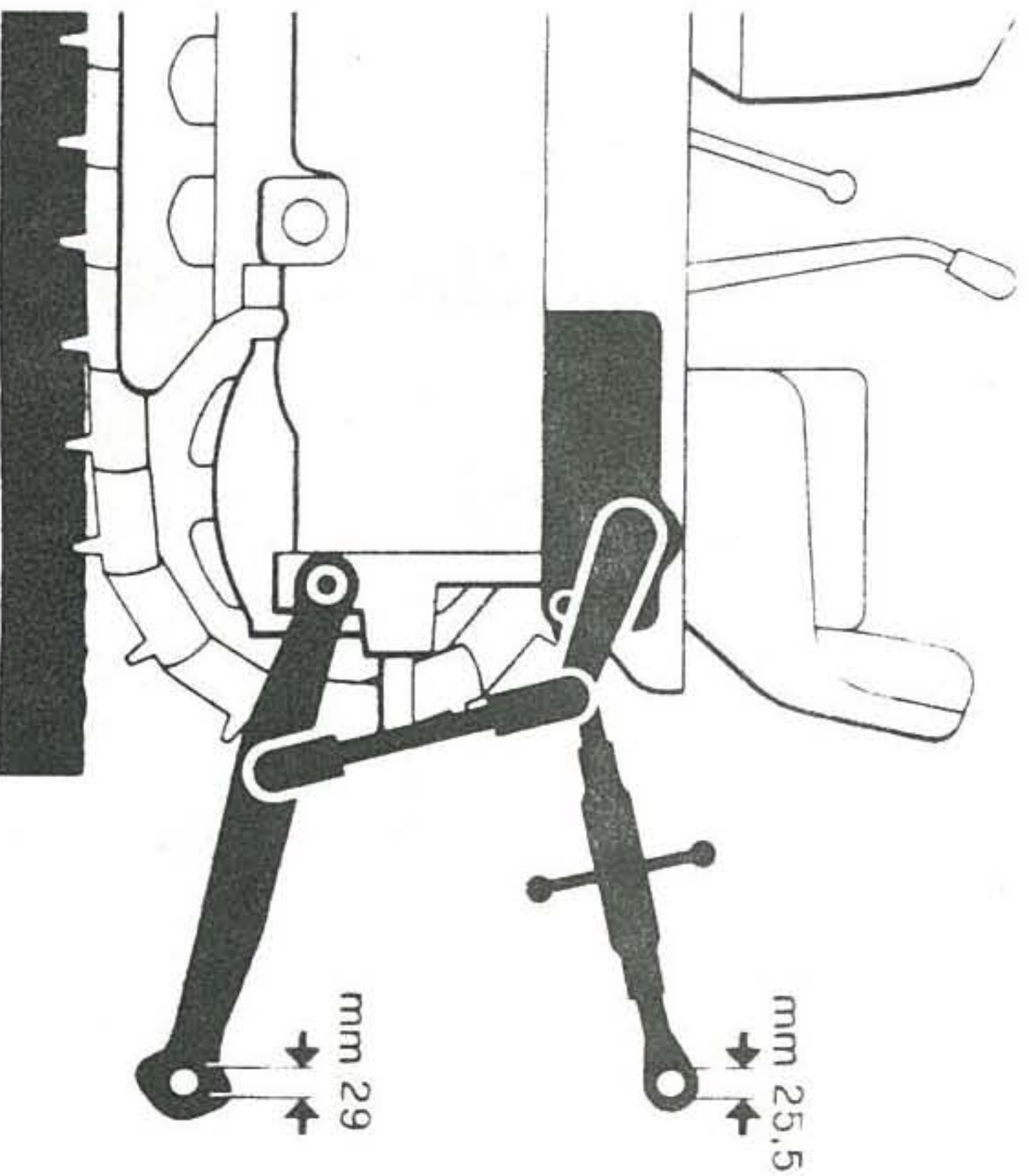
Fig. 11 - Engate de alfaías cat. II
