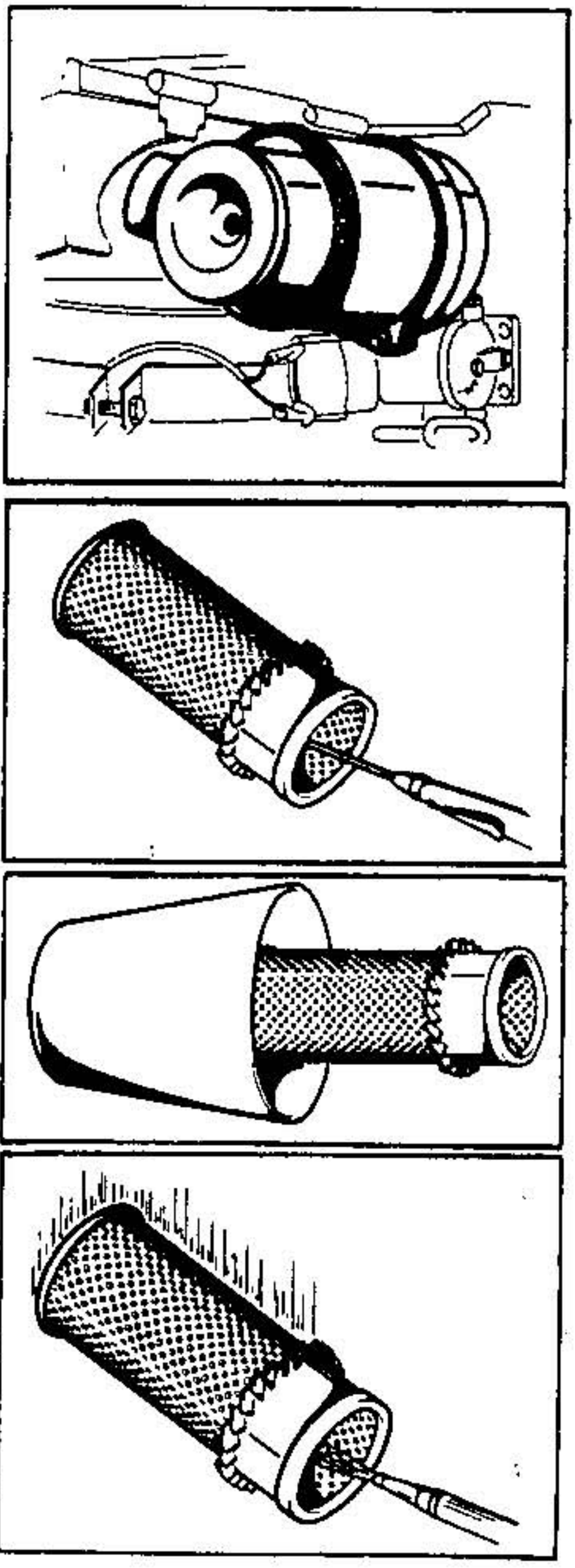
FIG. 13 - Filtro de ar a seco
