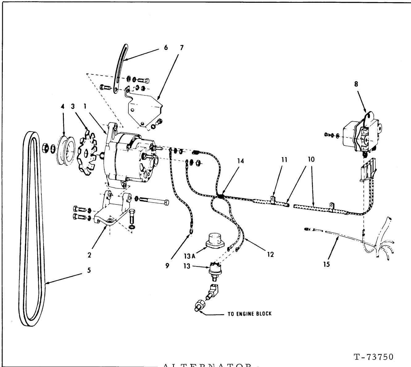
ALTERNATOR (Medium Output)
