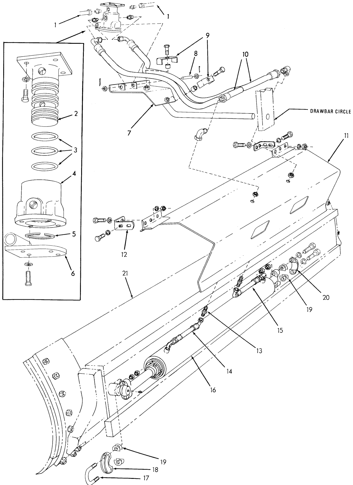
MOLDBOARD LATERAL SHIFT HYDRAULICS
