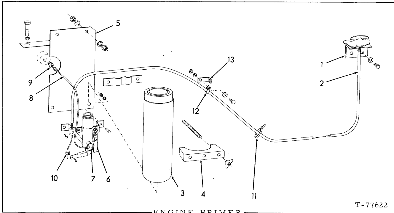
ENGINE PRIMER
