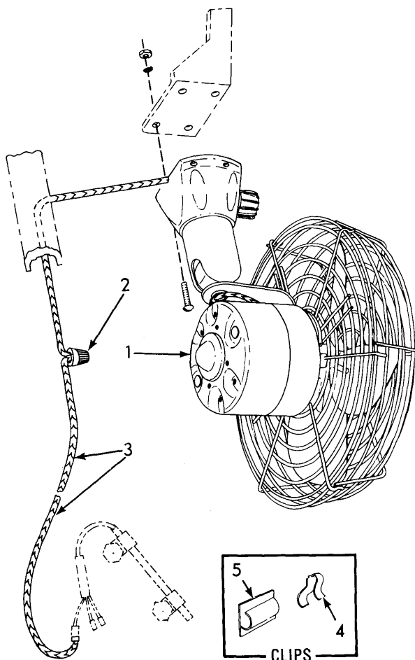
DEFROSTER FAN
