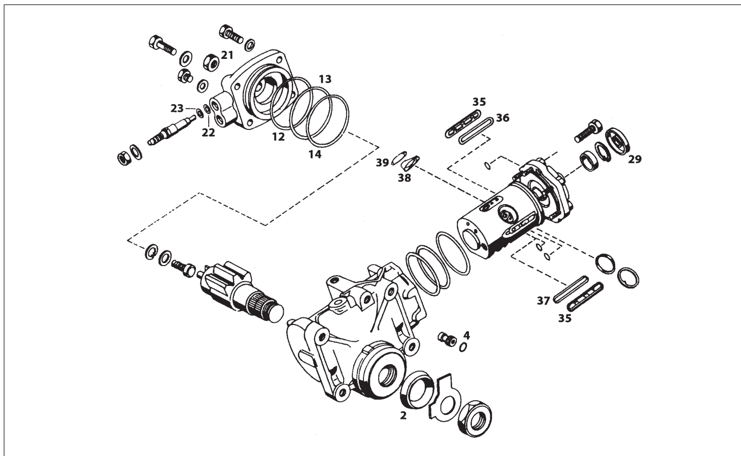
STEERING GEAR BOX (ZF)
