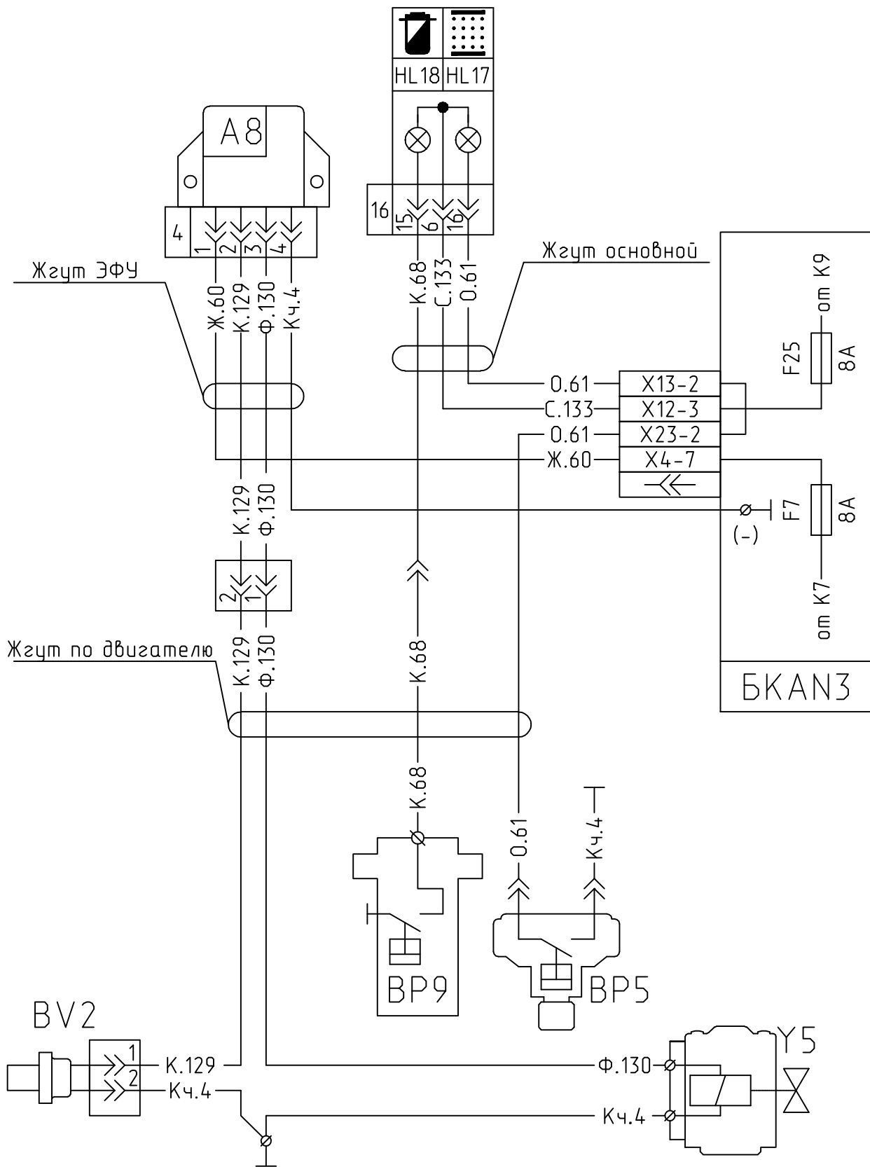
Блокировка демультимплекатора и датчики засоренности фильтров.
