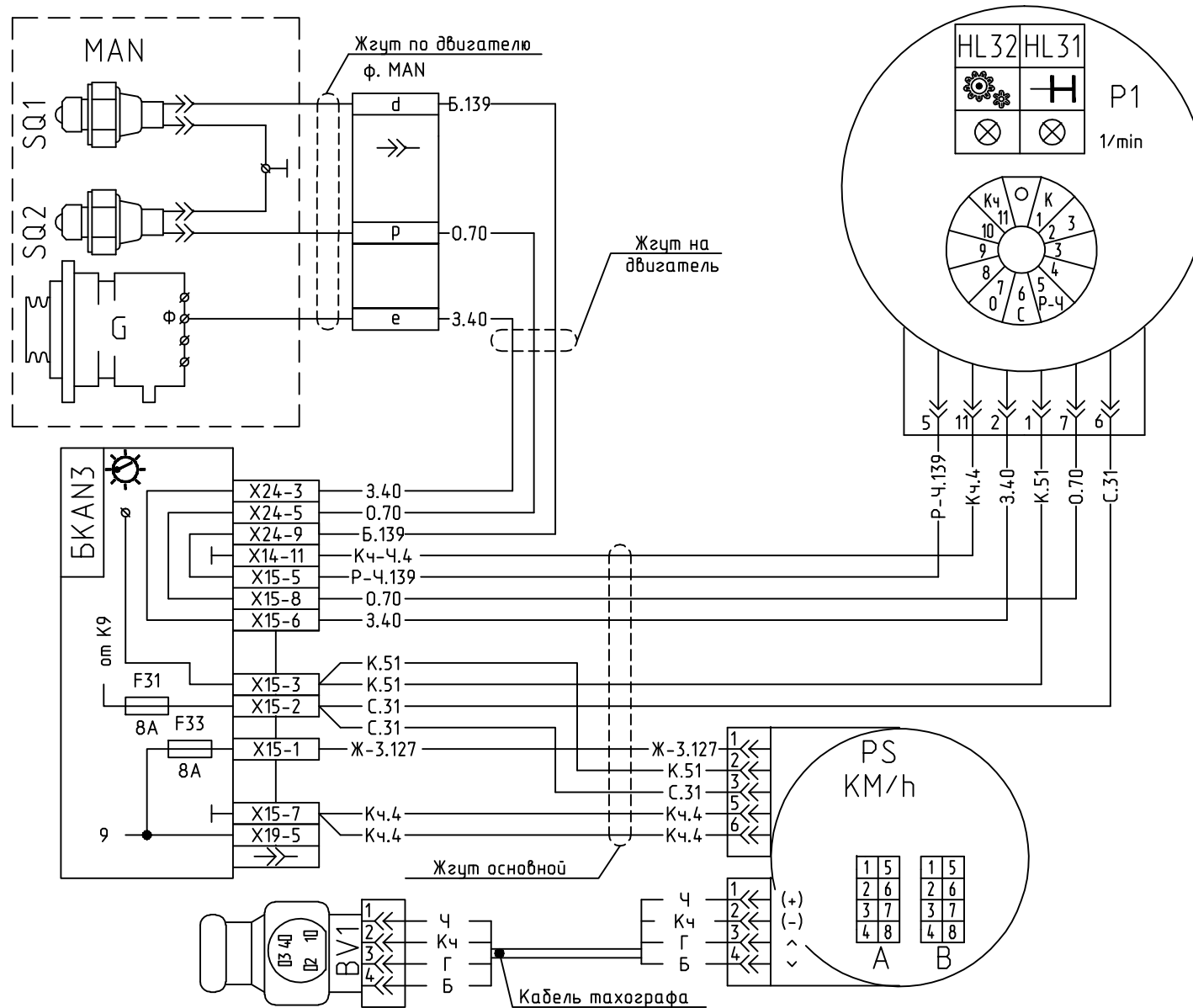
Система тахографа и тахометра для автомобилей с двигателем MAN.
