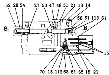
SECTION I - I
