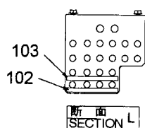
パイロット配管ブラケット PILOT PIPING BRACKET
