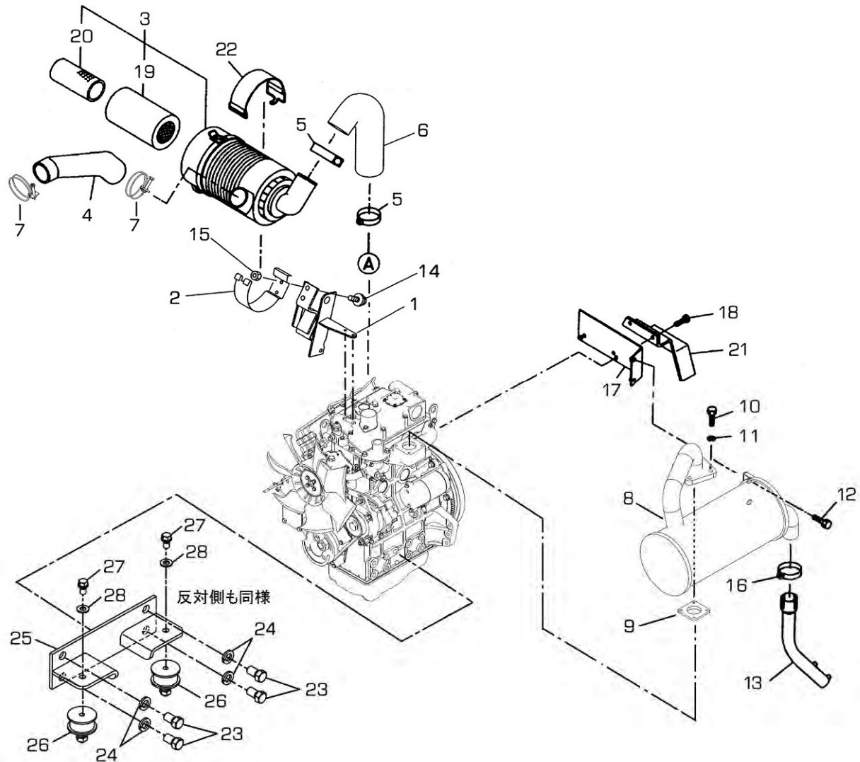
FIG.203-A AIR CLEANER, MUFFLER エアクリーナ、マフラー
