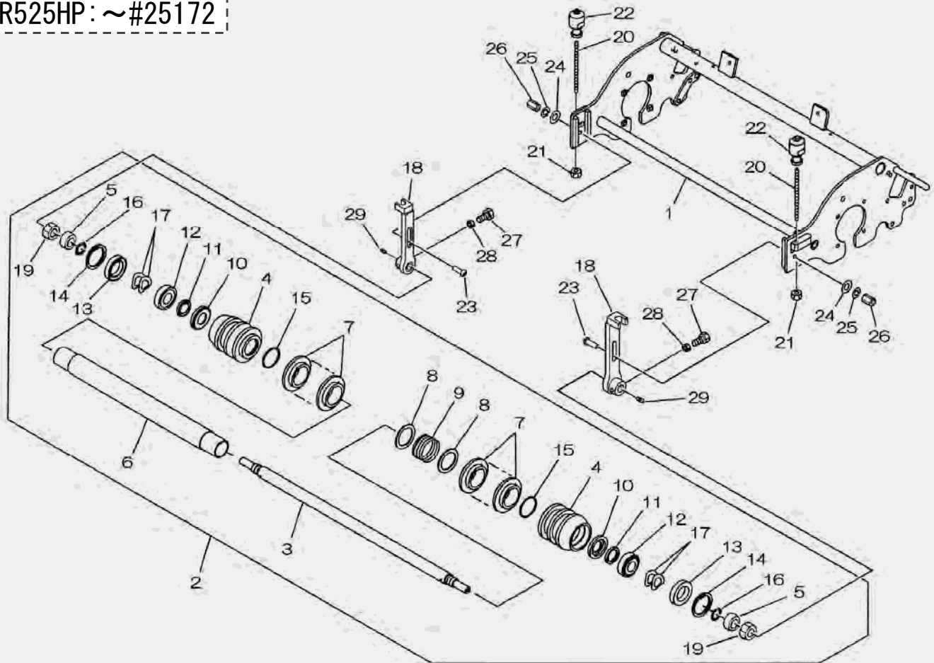
FIG.309-A FRONT ROLLER (W5/W7/W9) フロントローラー (W5/W7/W9)
