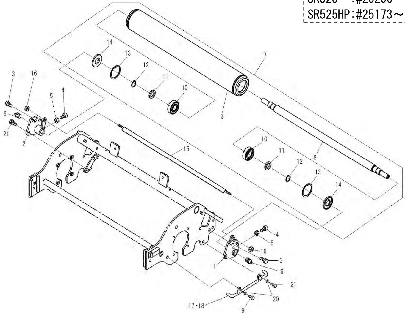
FIG.304-B REAR ROLLER (S7/S9/S11) リヤローラー (S7/S9/S11)
