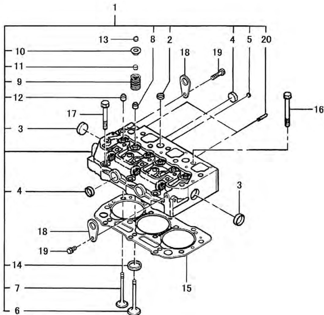
FIG.109 CYLINDER HEAD シリンダヘッド
