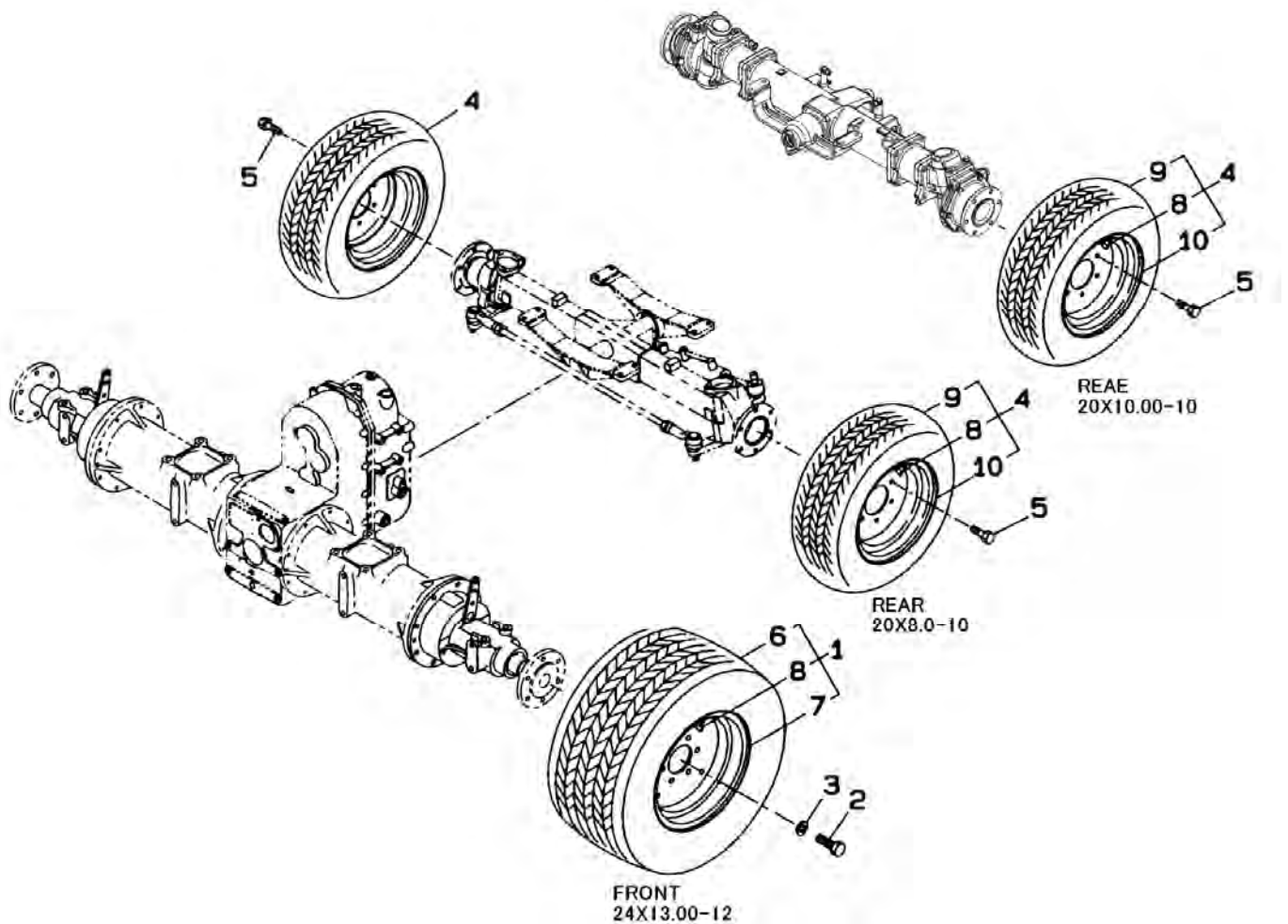
FIG.231 FRONT WHEELS, REAR WHEELS フロントホイール, リヤホイール
