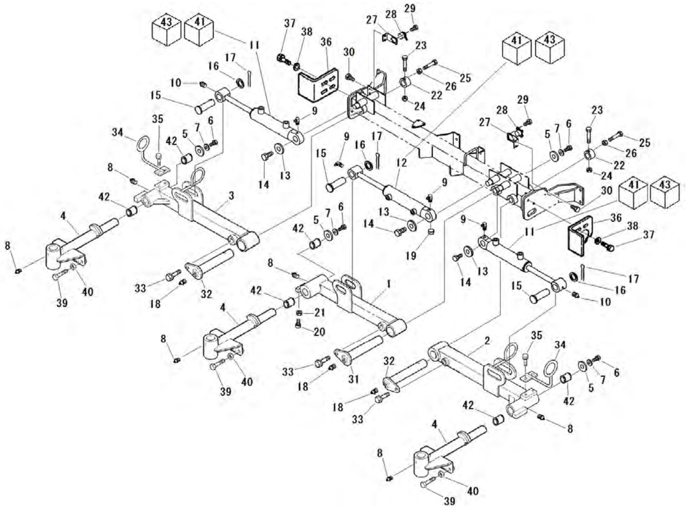
FIG.217-B CUTTER ARM (FRONT) 26INCH カッターアーム(フロント)
