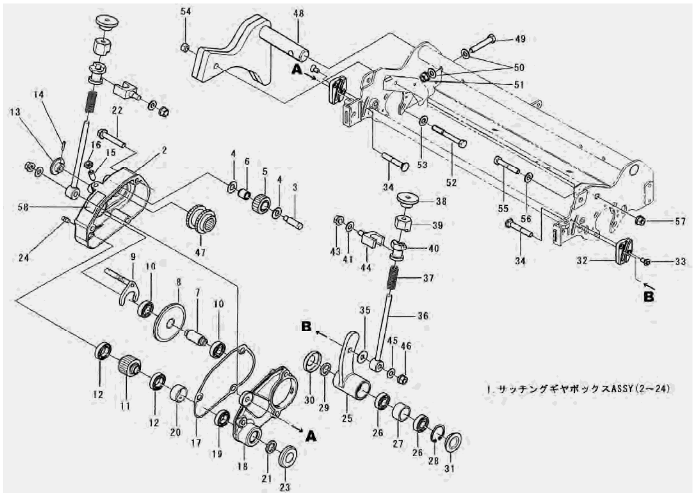
FIG.321 GEAR CASE (PD7) サッチングギヤケース (PD7)
