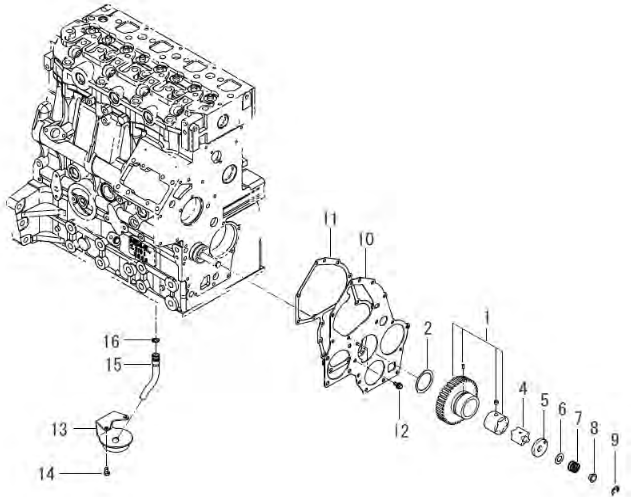
FIG.410 OIL PUMP,OIL FILTER オイルポンプ, オイルフィルター
