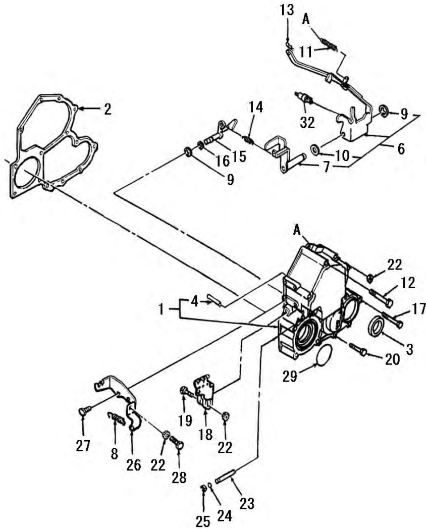
FIG.11 TIMING GEAR CASE タイミンギヤケース
