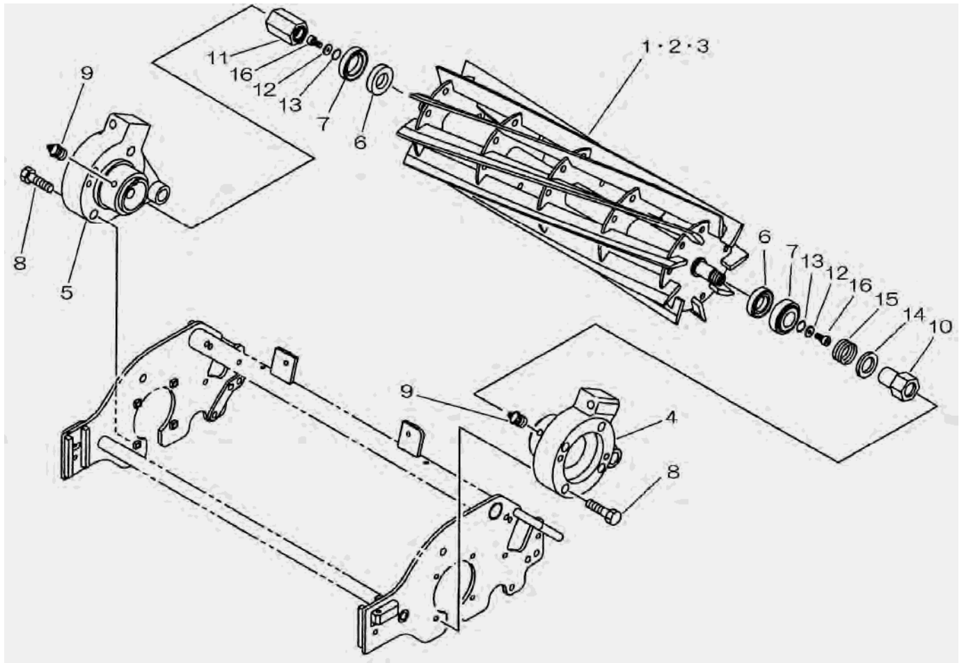
FIG.302 REEL BLADE (S7/S9/S11) カイテンバ (S7/S9/S11)
