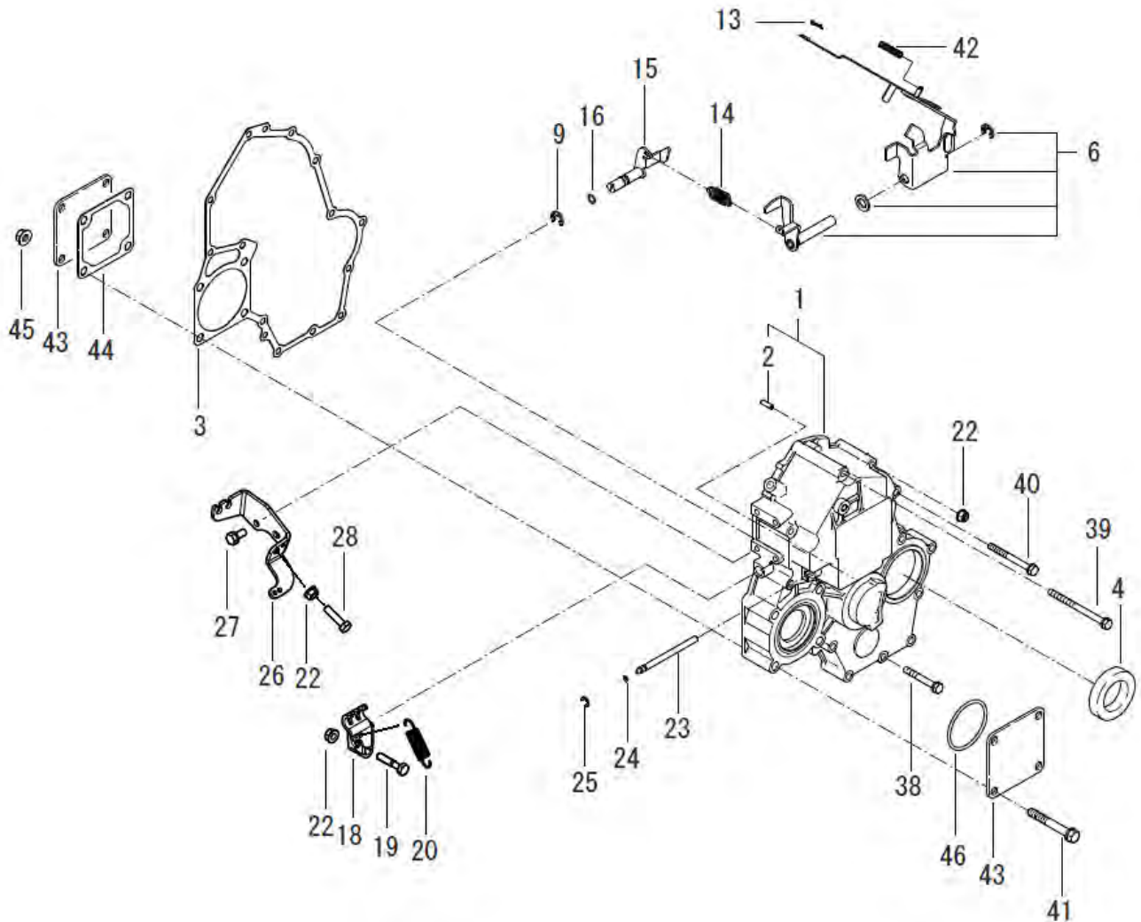
FIG.406 TIMING GEAR CASE タイミンギヤケース
