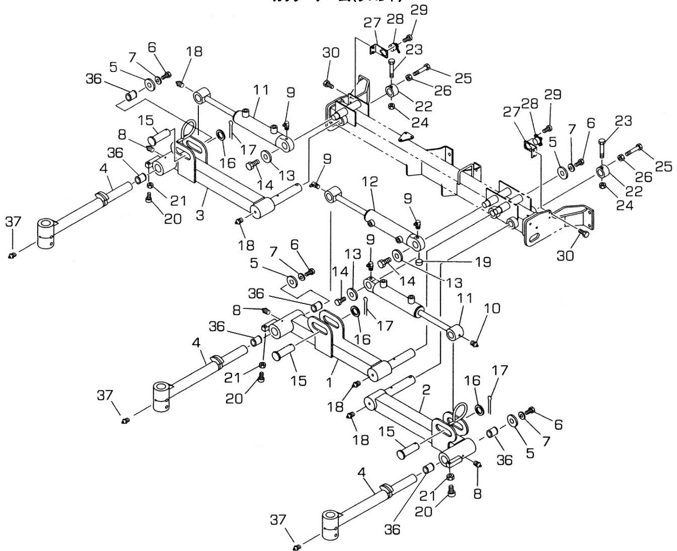
FIG.217-A CUTTER ARM (FRONT) 22INCH カッターアーム(フロント)
