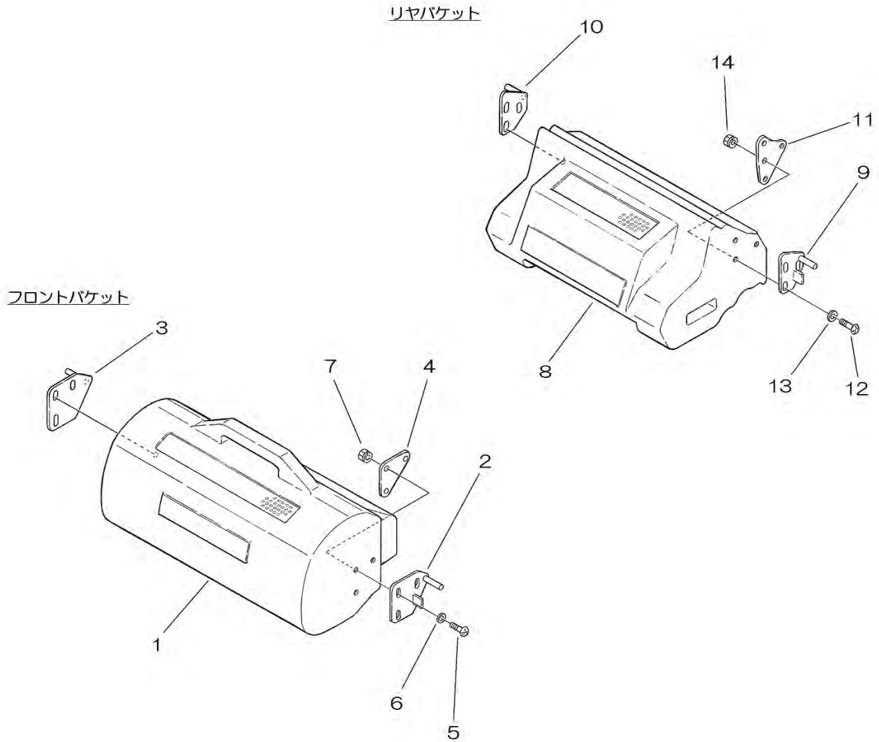
FIG.307 BUCKET (S7/S9/S11) バケット (S7/S9/S11)
