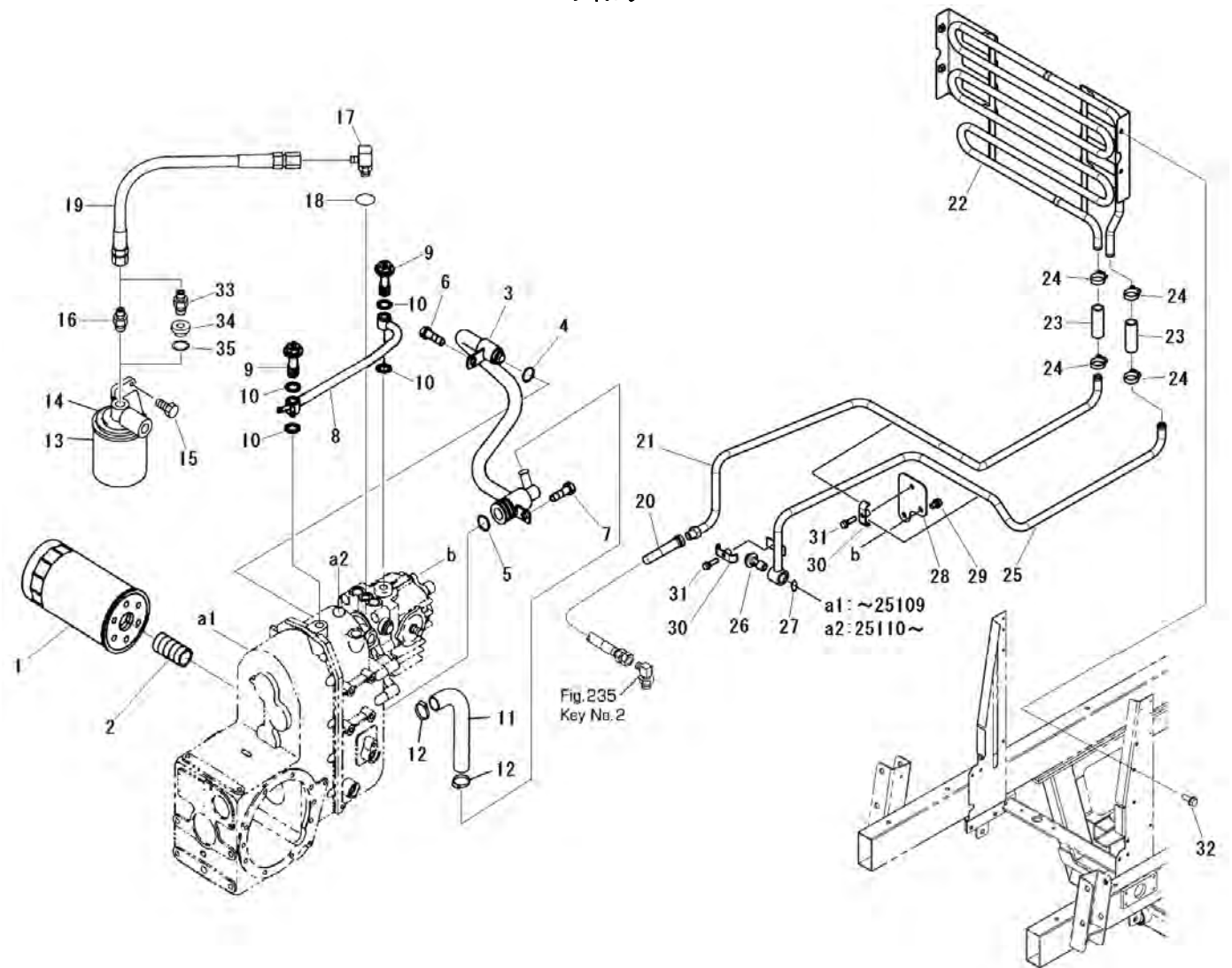
FIG.222-B FILTER, HYDRAULICS フィルター
