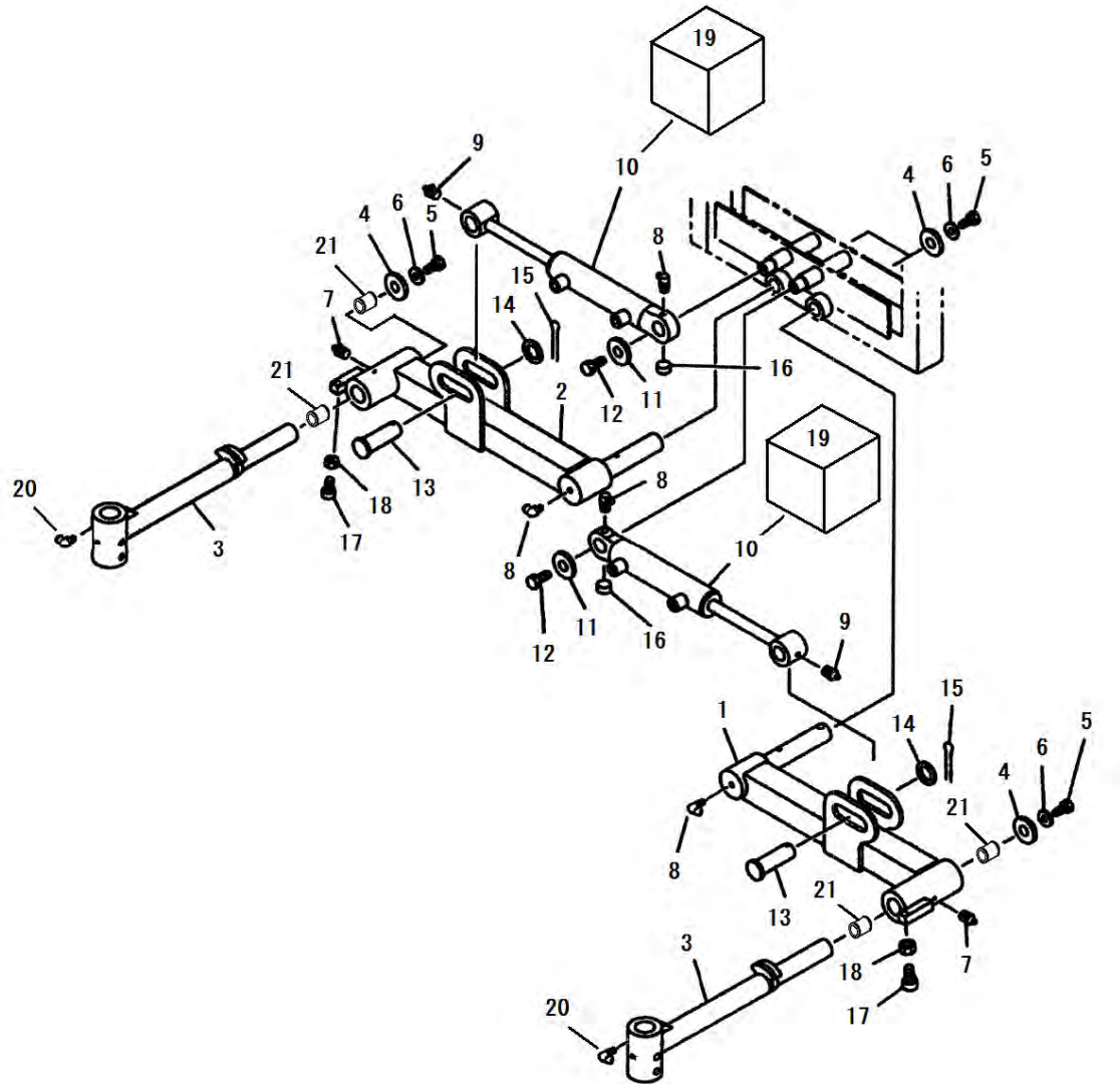
FIG.218-A CUTTER ARM(REAR) 22INCH カッターアーム(リヤ)
