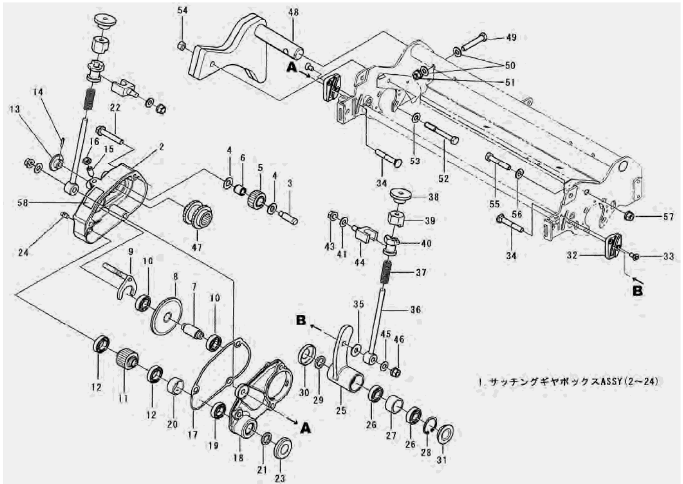
FIG.321 GEAR CASE (PD7) サッチングギヤケース (FD7)
