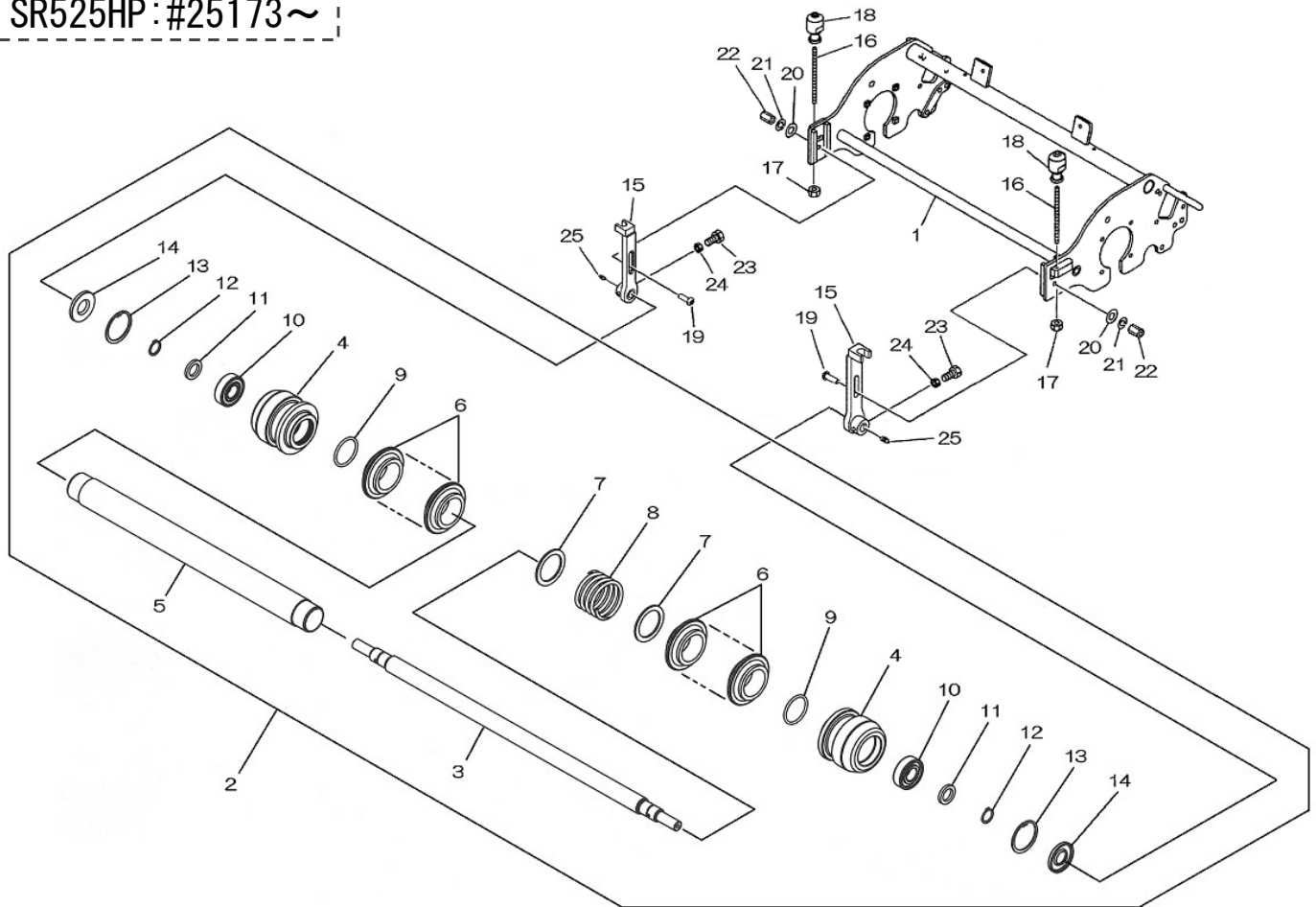
FIG.309-B FRONT ROLLER (W5/W7/W9) フロントローラー (W5/W7/W9)
