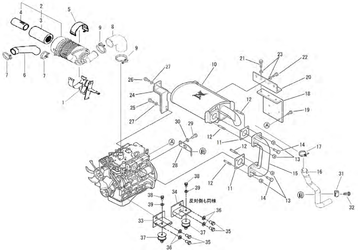
FIG.203-B AIR CLEANER, MUFFLER エアクリーナ、マフラー
