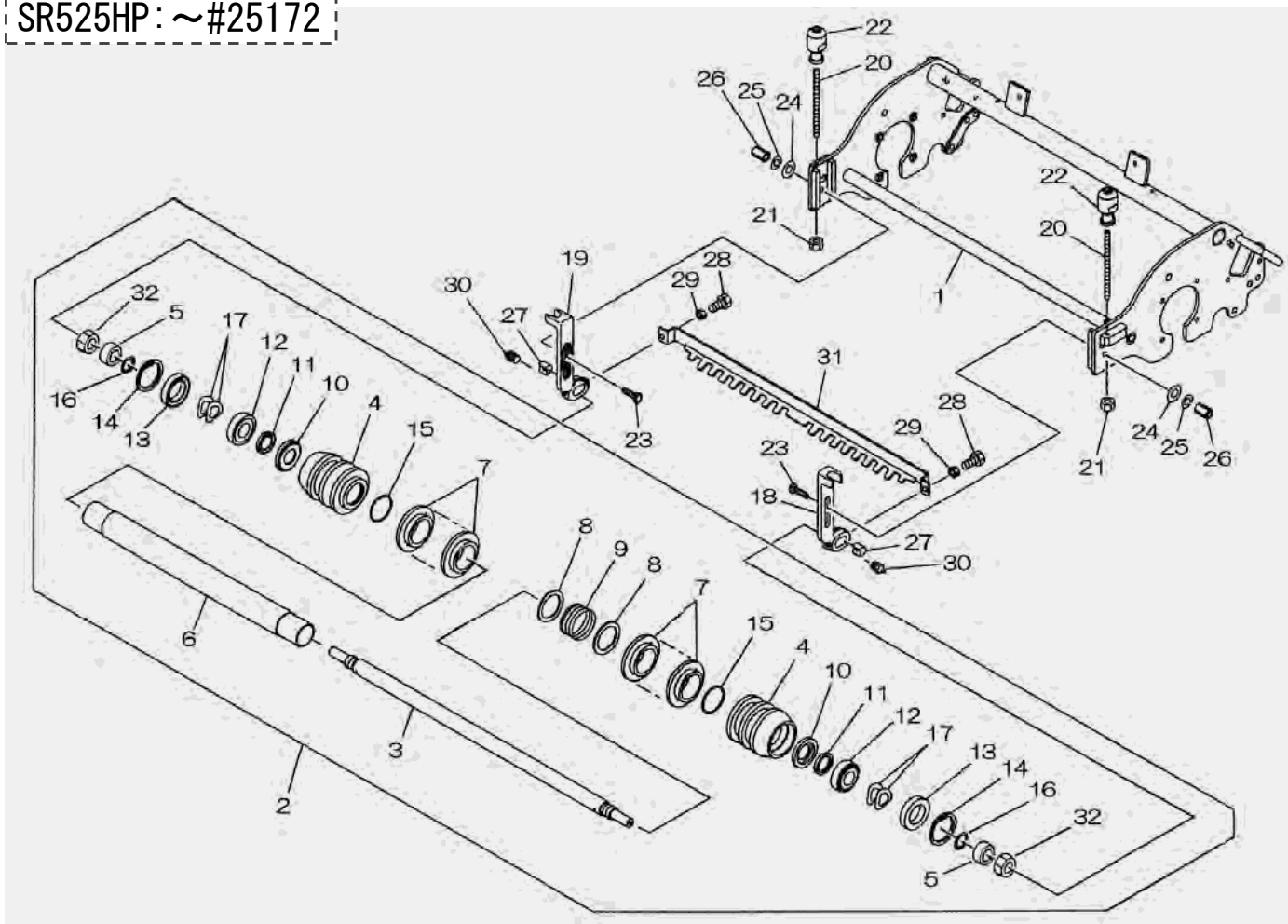
FIG.301-A FRONT ROLLER (S7/S9/S11) フロントローラー (S7/S9/S11)
