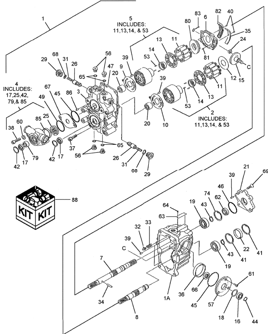
FIG.224 HYDRA-STATIC TRANSMISSION ユアツトランスミッション
