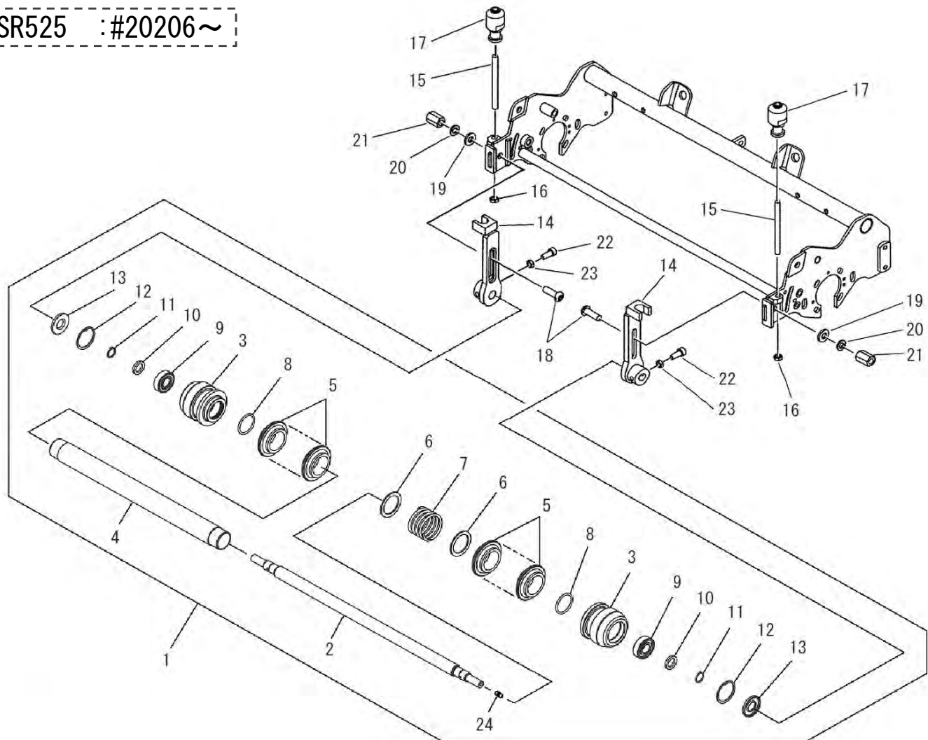
FIG.316-B FRONT ROLLER (F7) フロントローラー (F7)
