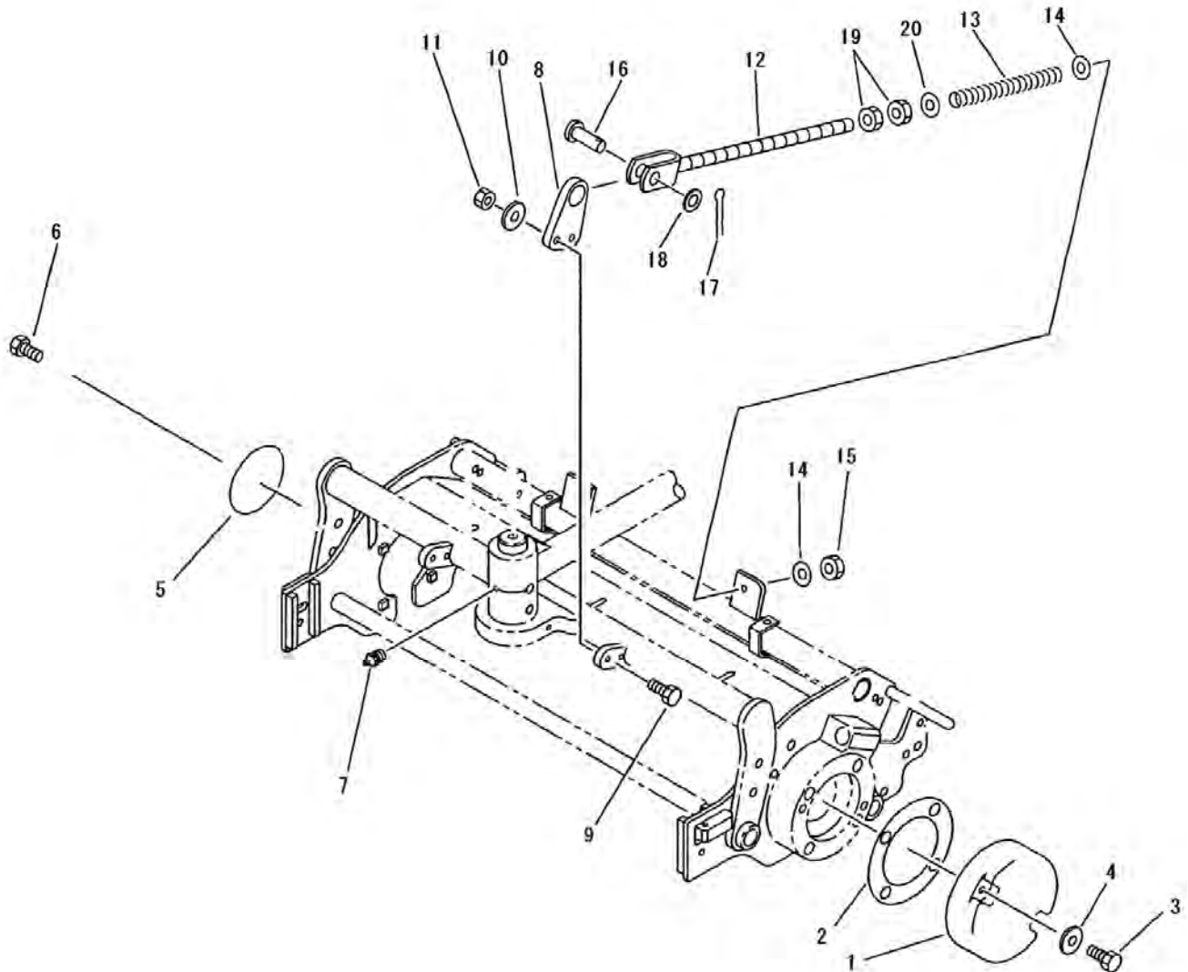
FIG.314 ACCESSORY (W5/W7/W9) フックピン (W5/W7/W9)
