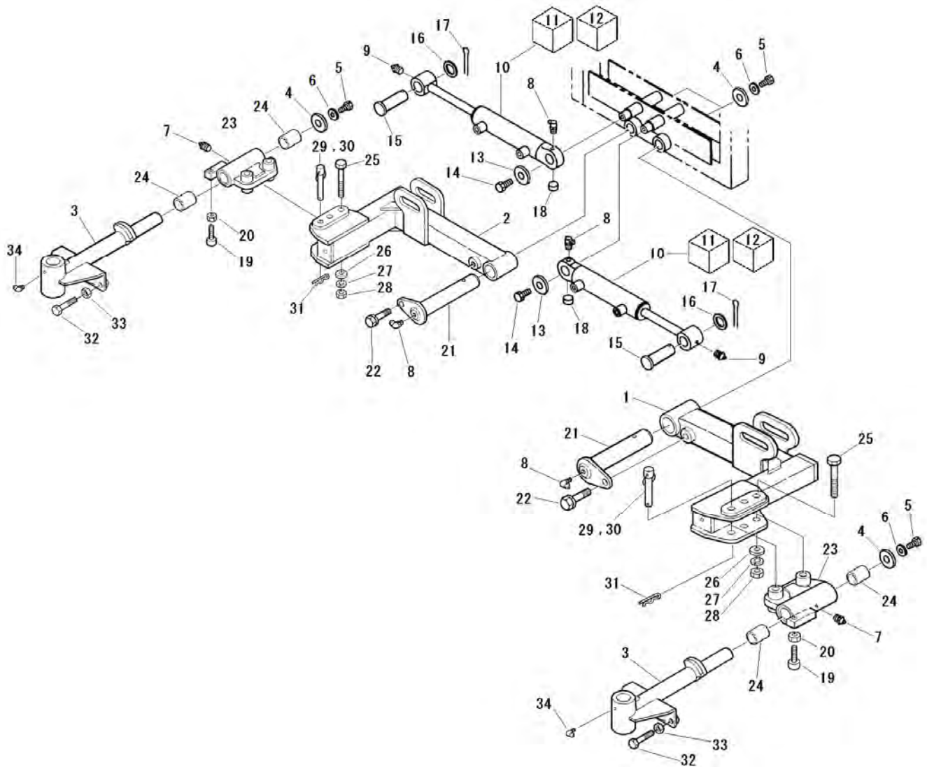
FIG.218-B CUTTER ARM(REAR) 26INCH カッターアーム(リヤ)
