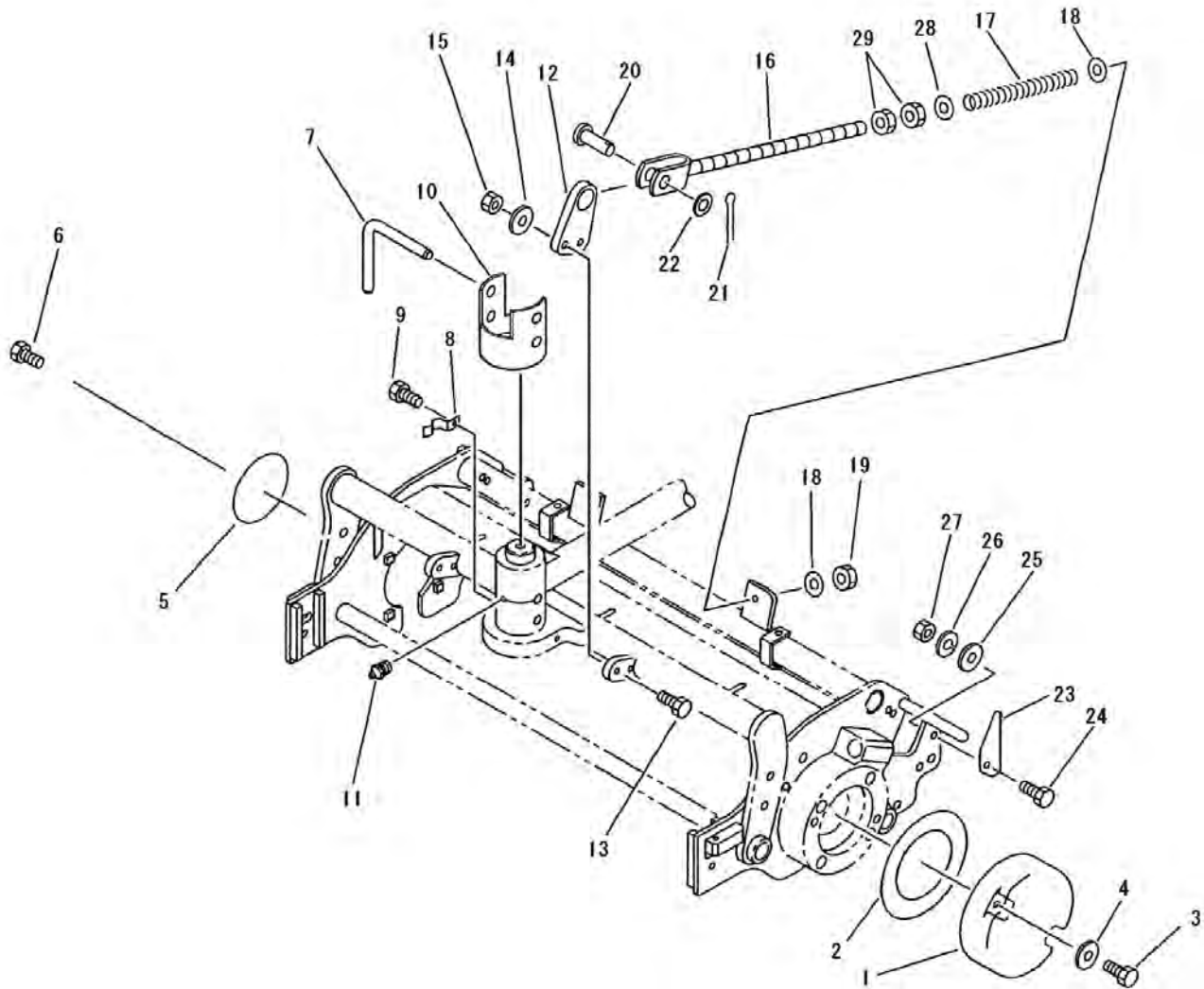
FIG.308 ACCESSORY (S7/S9/S11) フックピン (S7/S9/S11)
