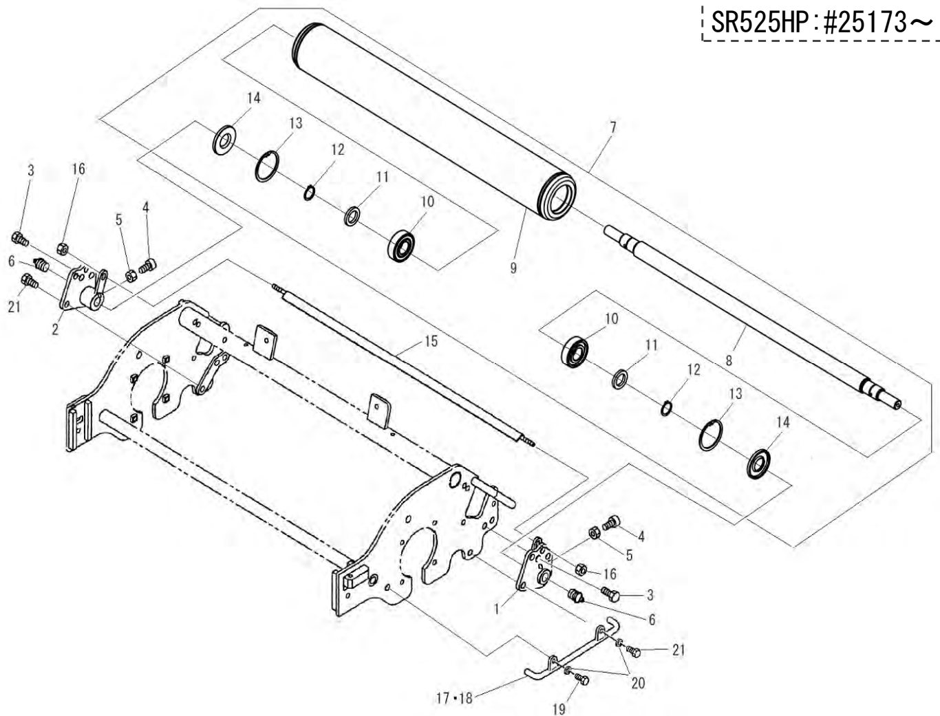
FIG.312-B REAR ROLLER (W5/W7/W9) リヤローラー (W5/W7/W9)
