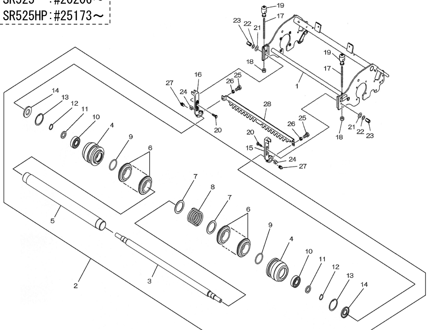
FIG.301-B FRONT ROLLER (S7/S9/S11) フロントローラー (S7/S9/S11)
