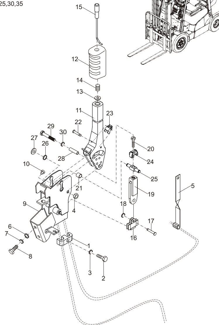
停车制动装置/BRAKE LEVER
