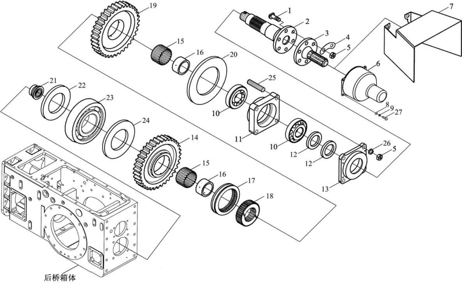
动力输出轴总成(二) PTO Shaft Assembly( II )
