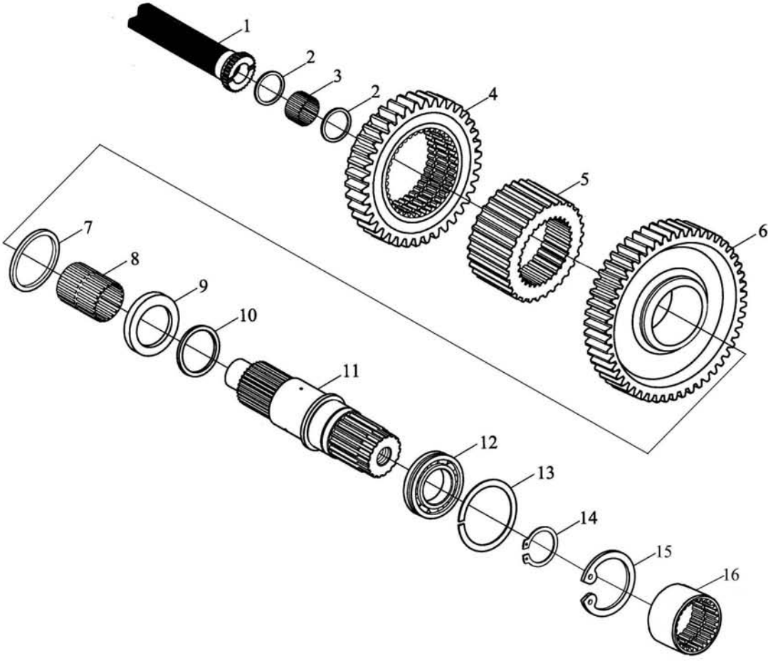
变速箱总成（四） Gearbox Assembly( IV ) 62
