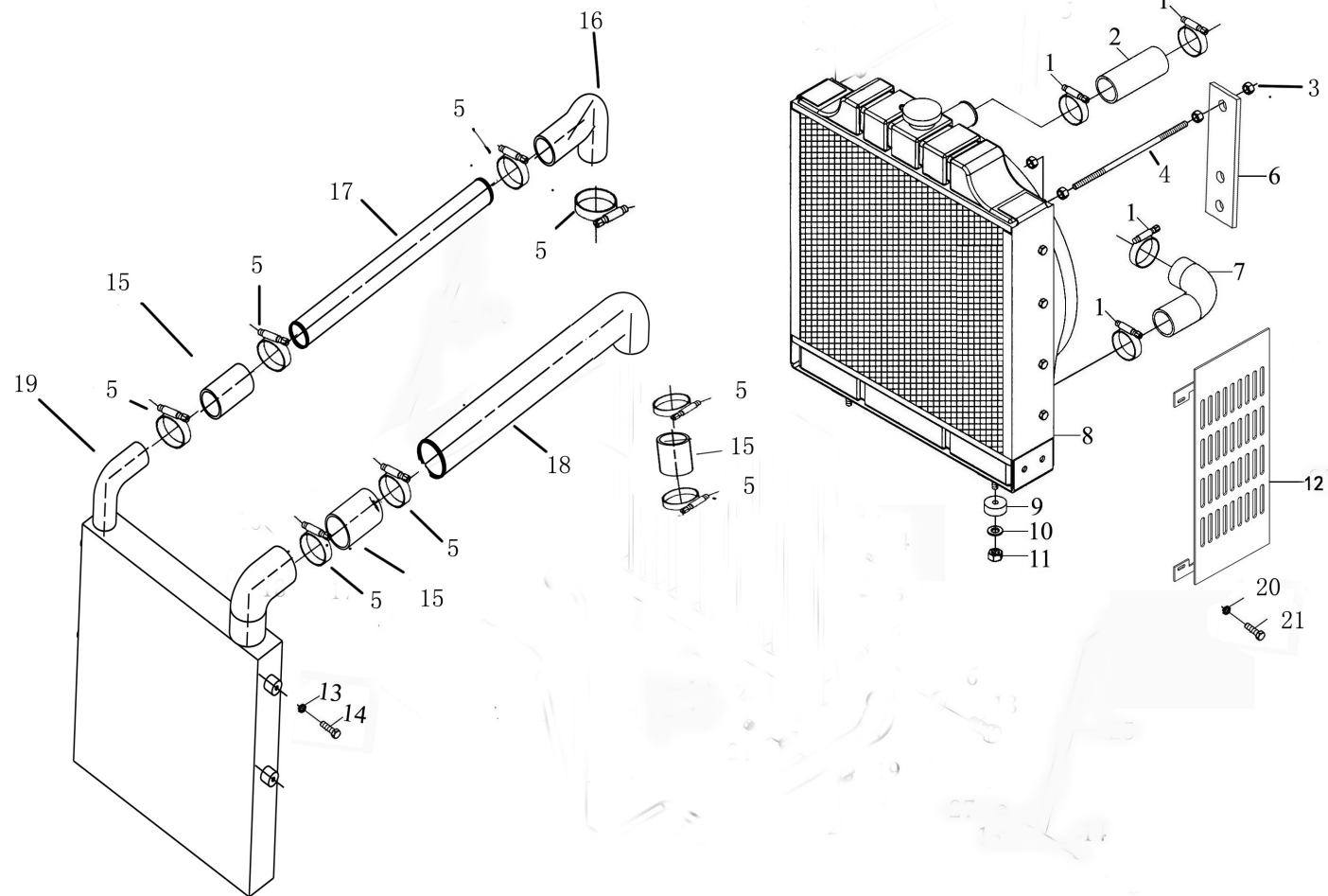
水箱散热器及管路总成 Radiator and pipes Assembly
