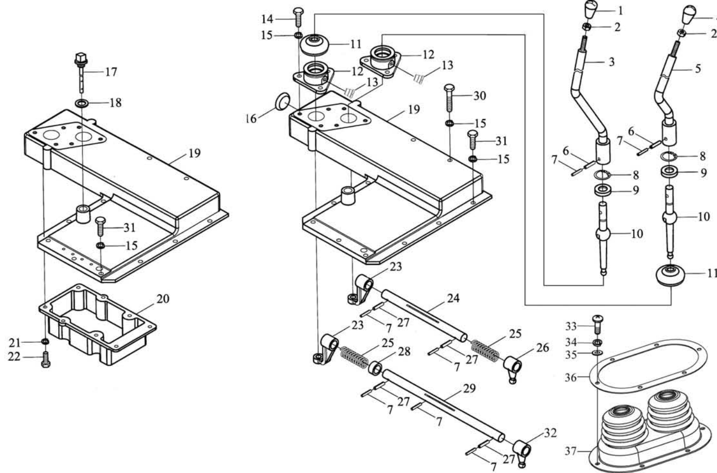
变速箱总成 (六) Gearbox Assembly (VI)
