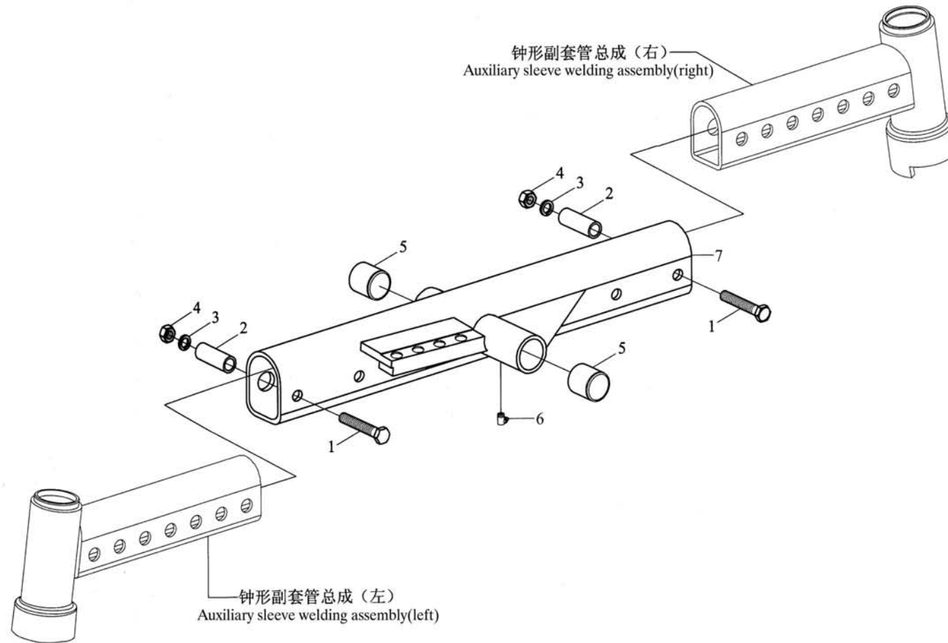
前轴总成 (四) Front Axle Assembly (IV)
