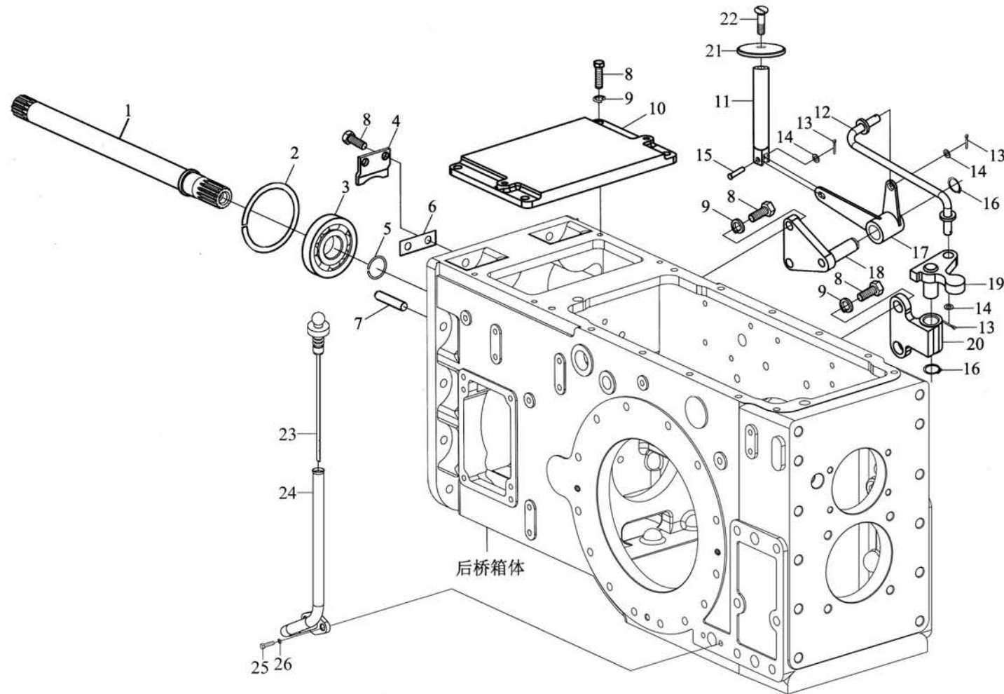
后桥总成 (三) Rear Axle Assembly (III)
