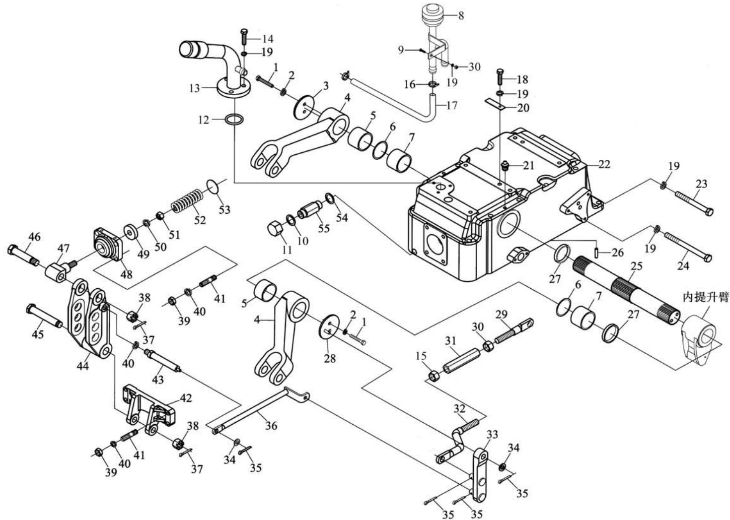
提升器总成 (一) Power Lifter Assembly(I)
