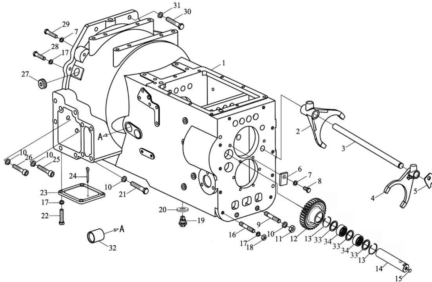
变速箱总成 (八) Gearbox Assembly (VIII)
