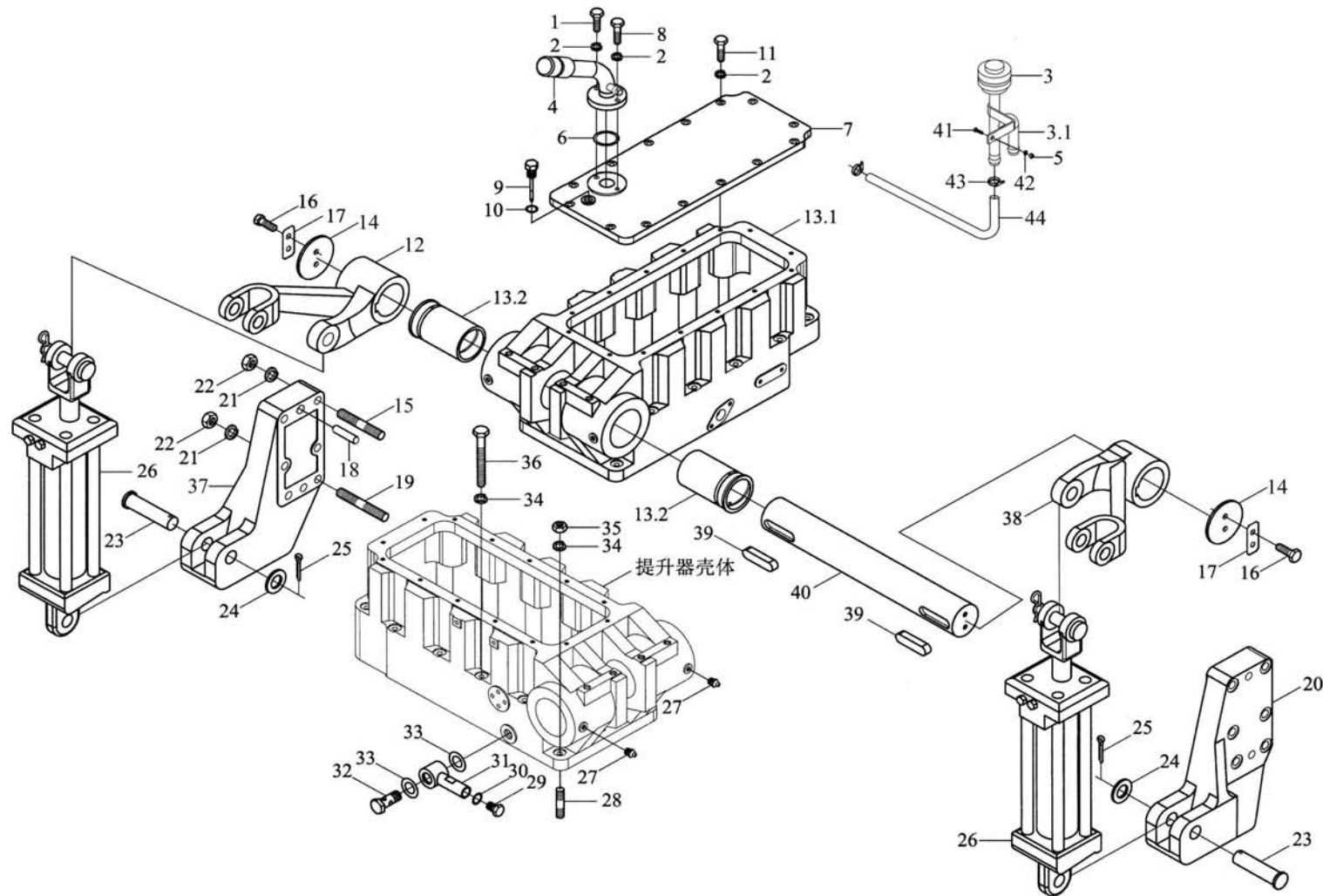
提升器总成 (三) Power Lifter Assembly (III)
