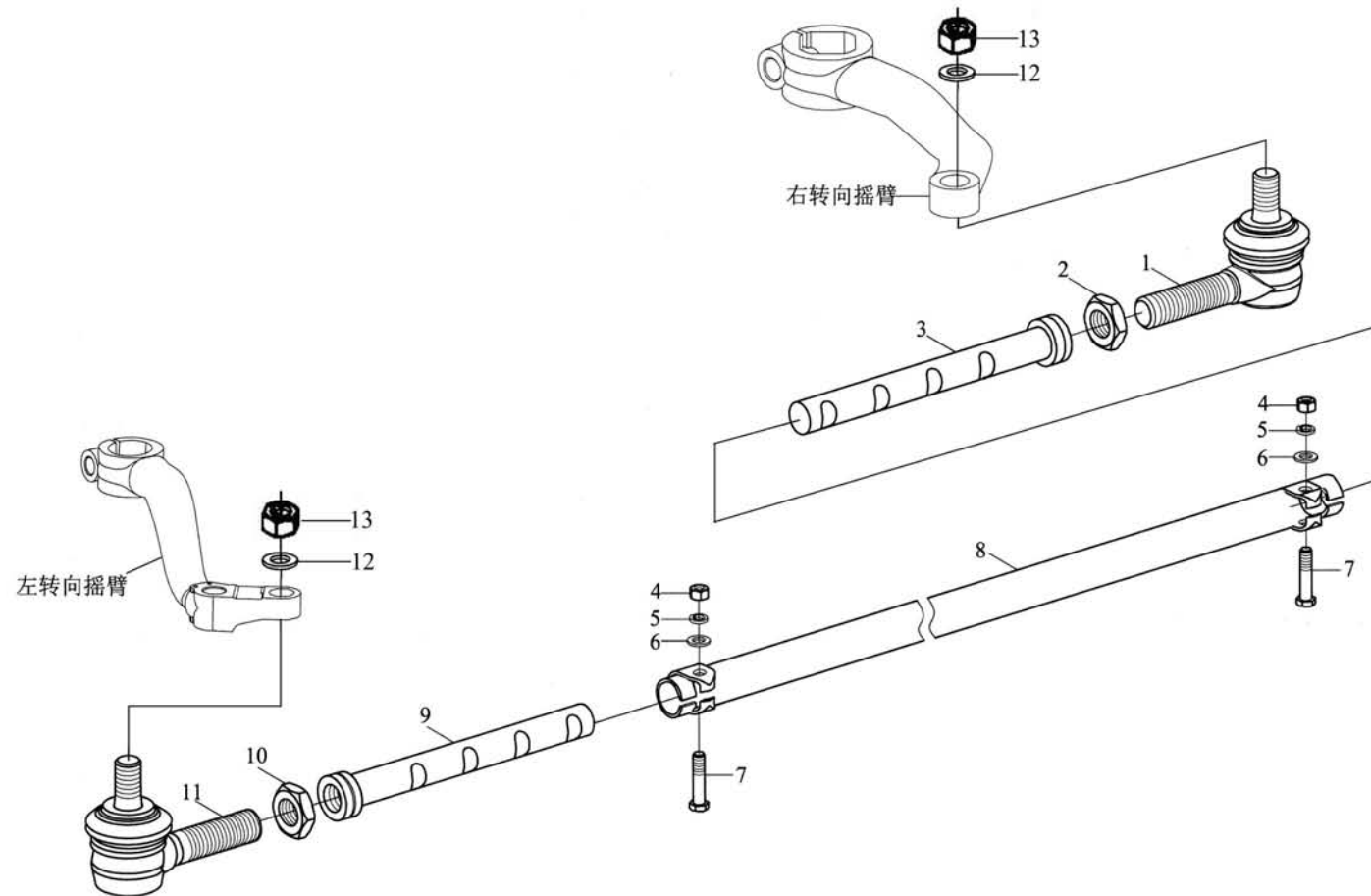
前轴总成 (一) Front Axle Assembly ( I )
