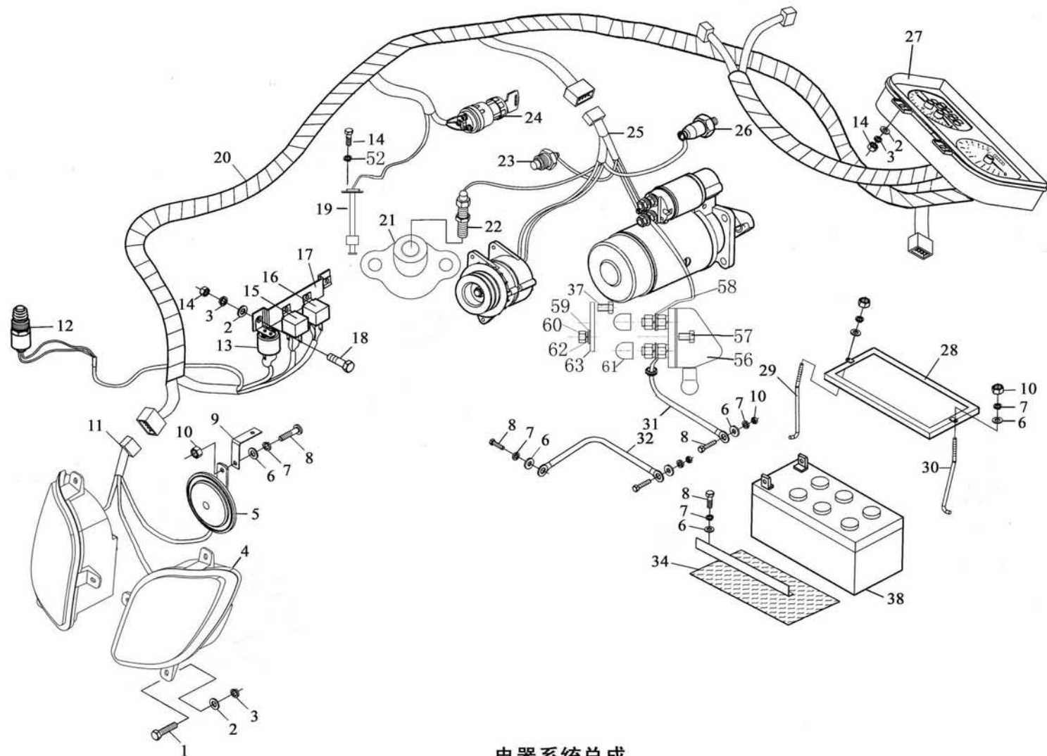
电器系统总成 Electrical System Assembly
