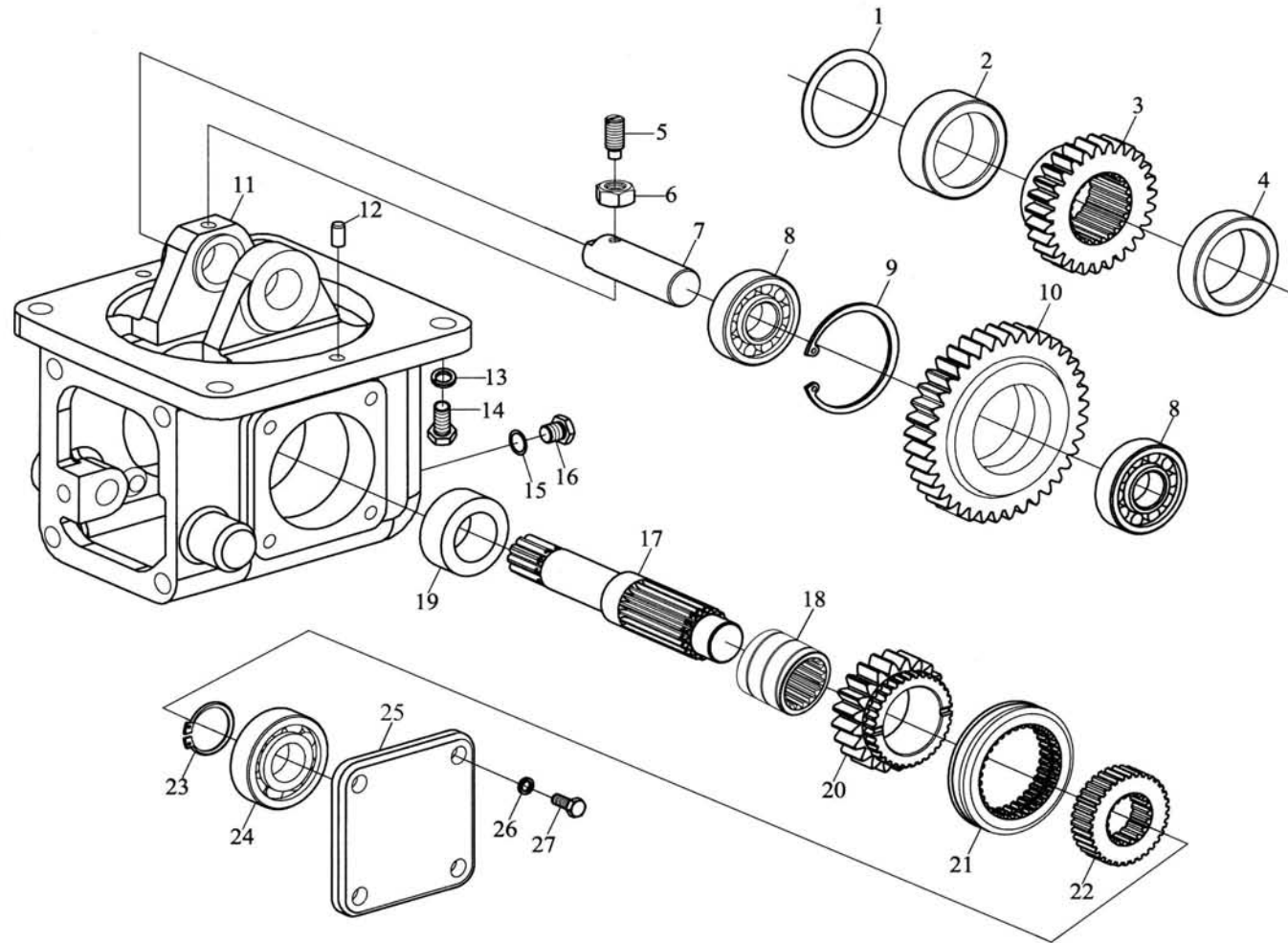
分动箱总成 (三) Transfer Case Assembly (III)
