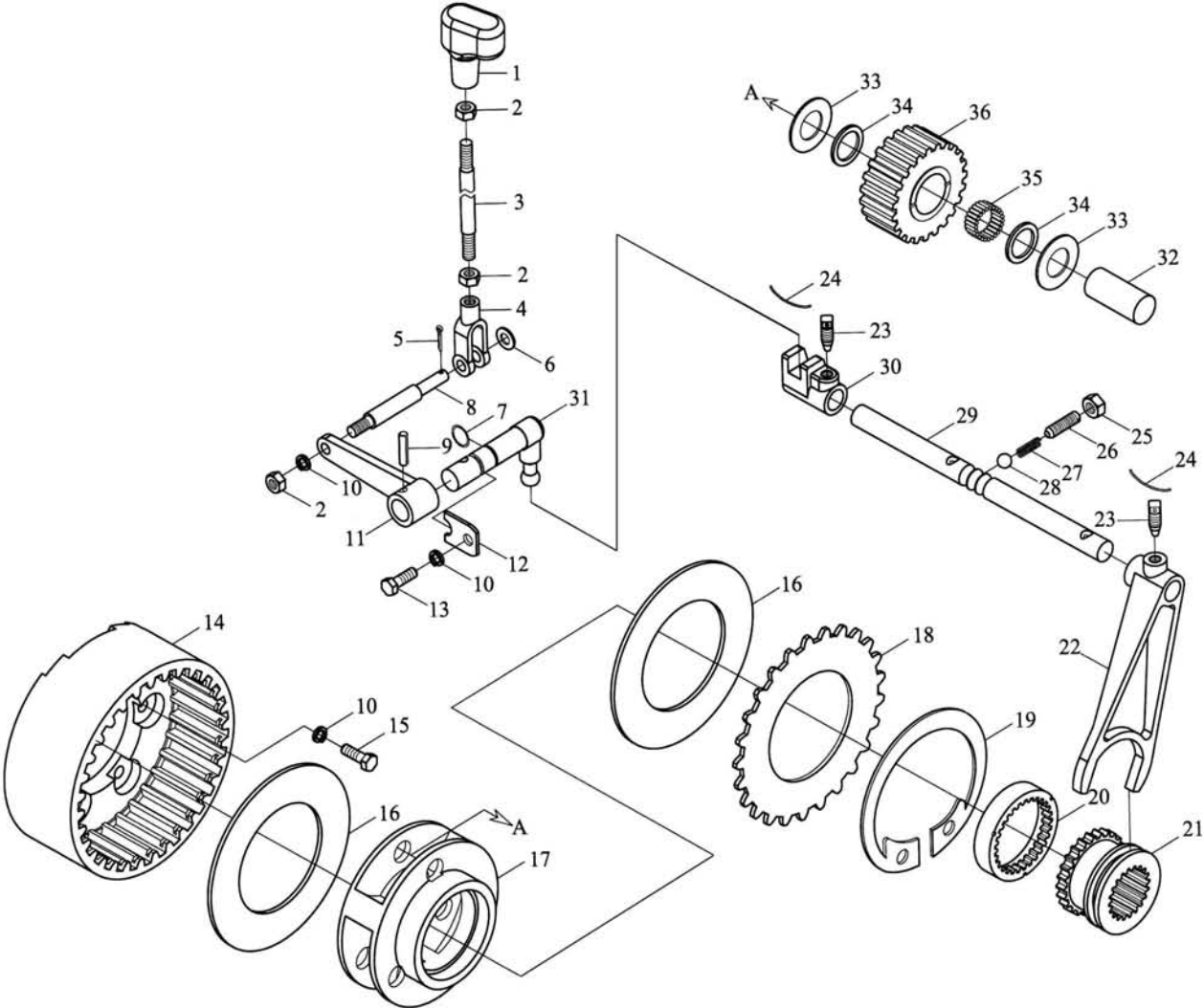
变速箱总成 (七) Gearbox Assembly (VII) 69
