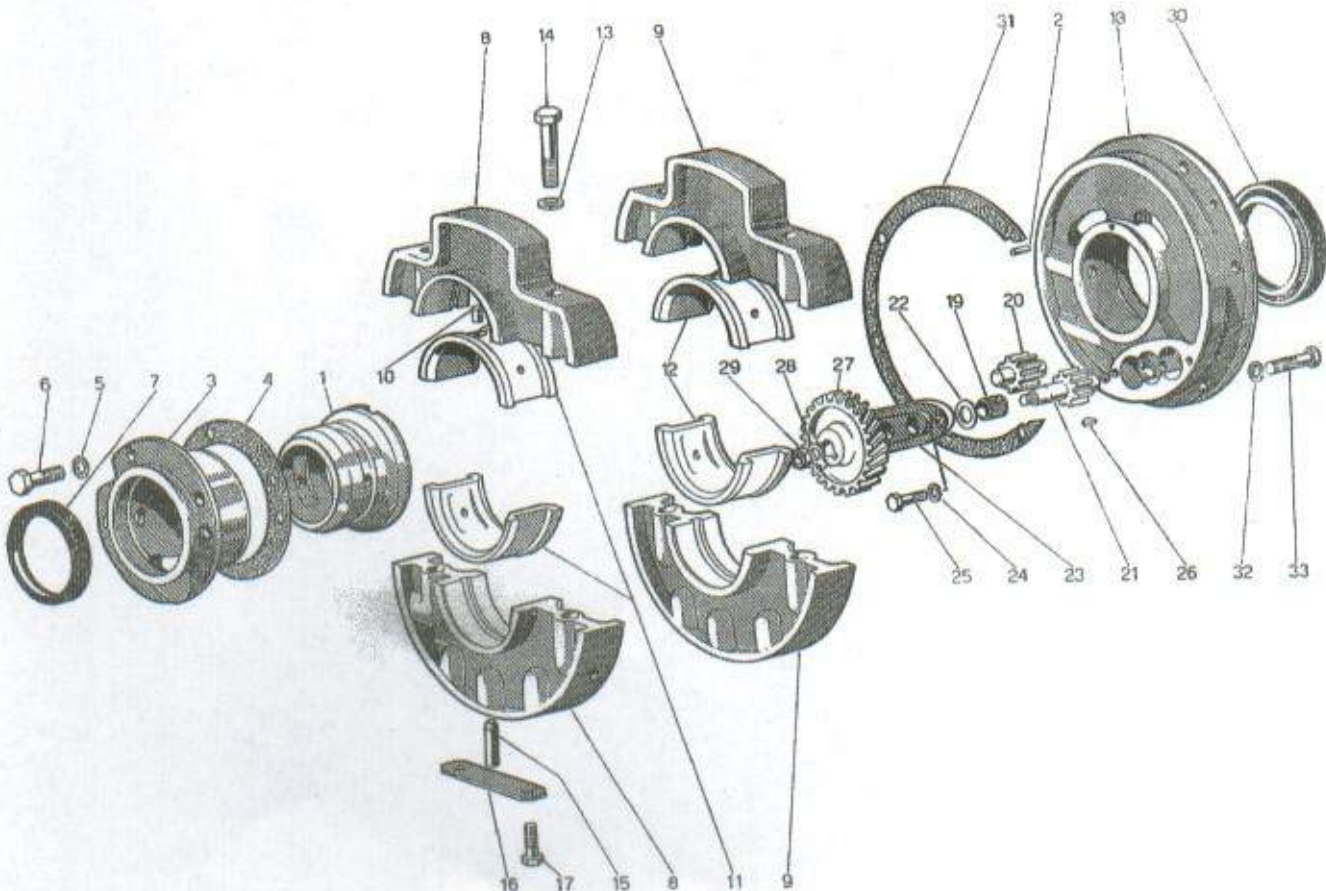
SUPPORTI CUSCINETTI DI BANCO
