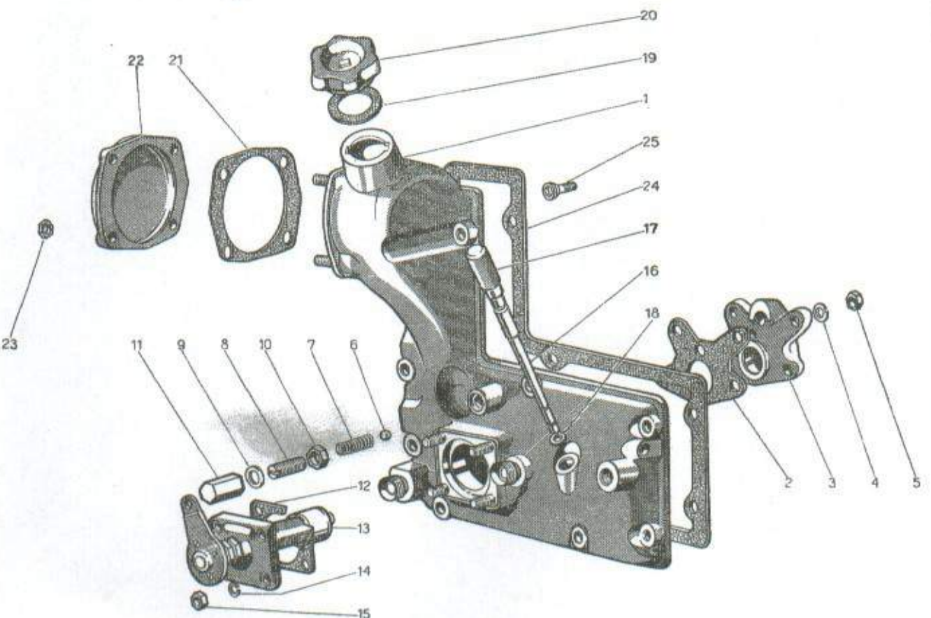
COPERCHIO FILTRO LIVELLO OLIO
