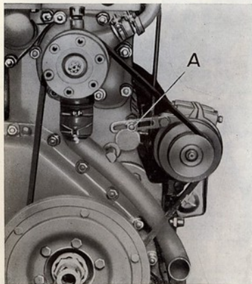
Fig. 24. - Tensado de las correas del mando-ventilador, bomba de agua y dinamo
