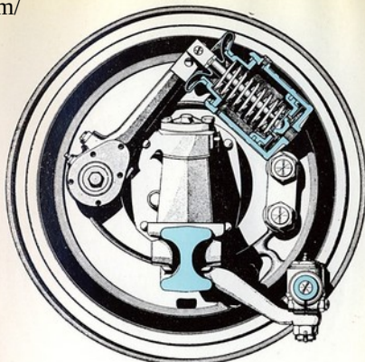
Fig. 46. - Frenos anteriores
