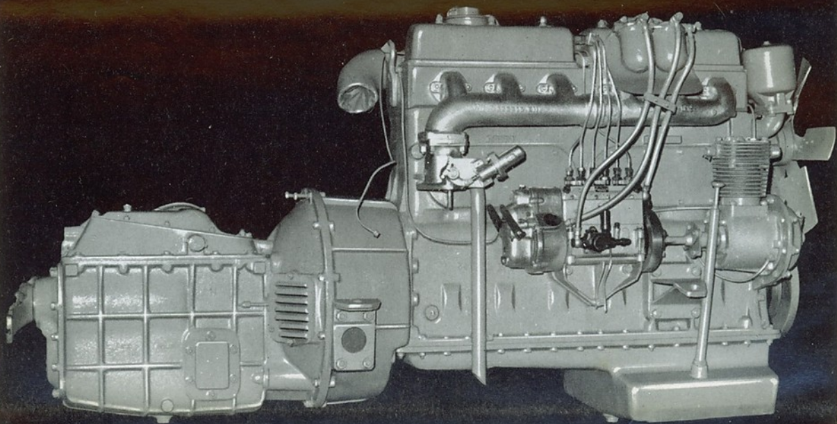
Fig. 11. - Motor, embrague y cambio (visto lado derecho)
