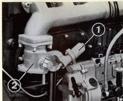
Fig. 49. - Freno-motor incorporado sobre el tubo de escape
