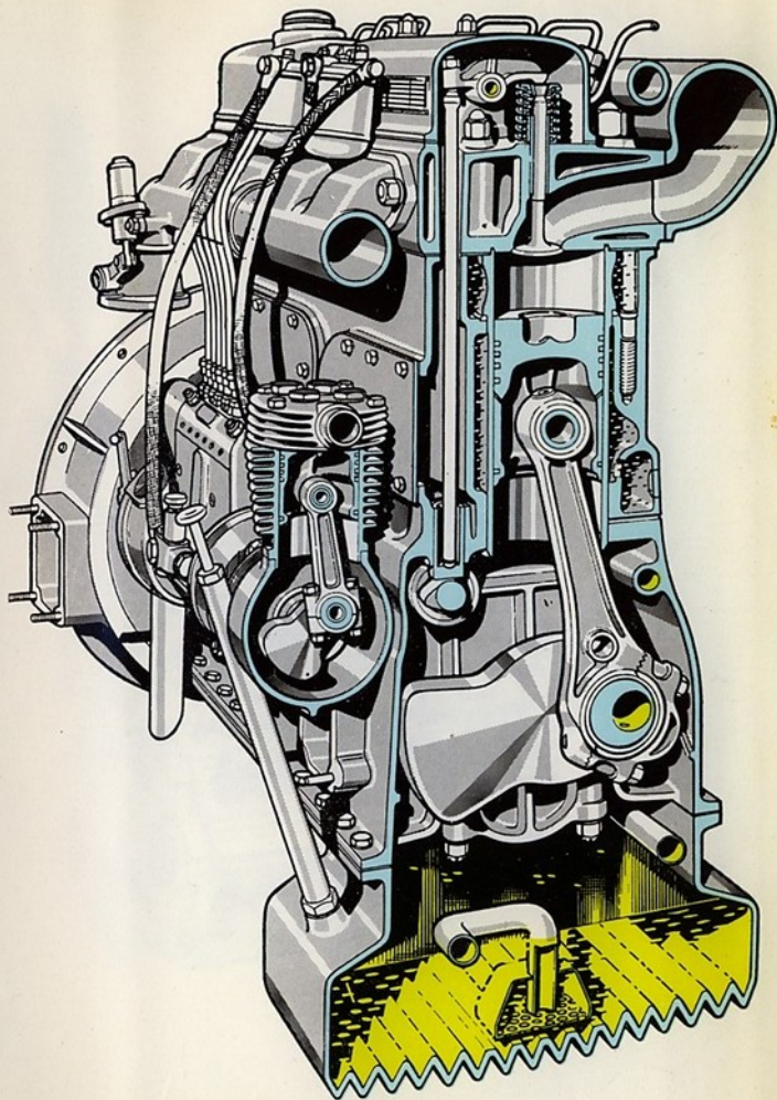
Fig. 13. - Motor (corte transversal)
