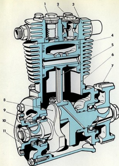
Fig. 42. - Compresor
