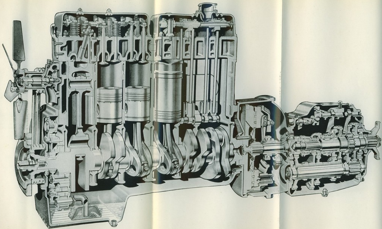
Fig. 13 bis. - Motor, embrague y cambio (sección longitudinal)
