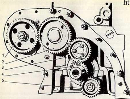
Fig. 21. - Engranajes de la distribución
