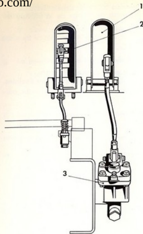
Fig. 50. - Pedal de freno y pedal acelerador
