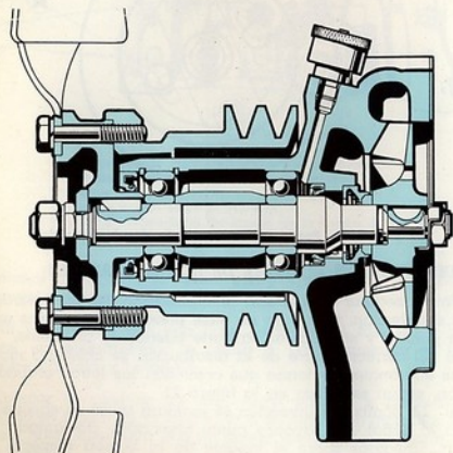
Fig. 22. - Bomba de agua
