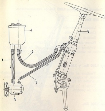
Fig. 36. - Esquema general de la Servodirección "Virex-Fulmina"
