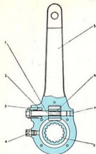
Fig. 45. - Palanca para ajuste de las mordazas
