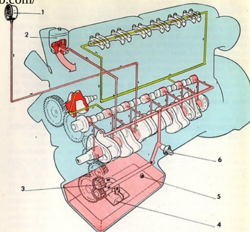
Fig. 15. - Esquema del circuito de lubricación
