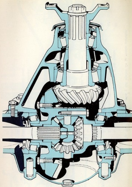
Fig. 30. - Diferencial
