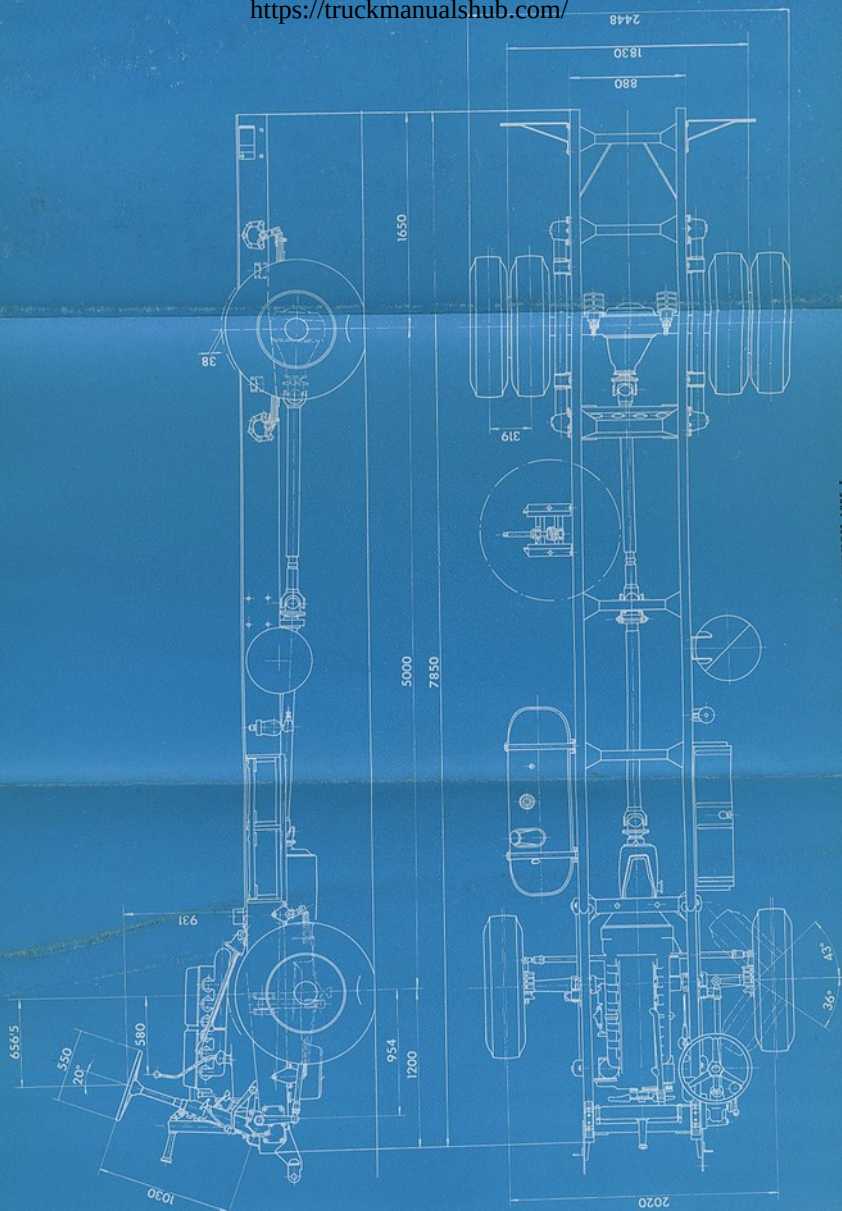
FIG. 5. - CAMION 1065 L DIMENSIONES GENERALES
