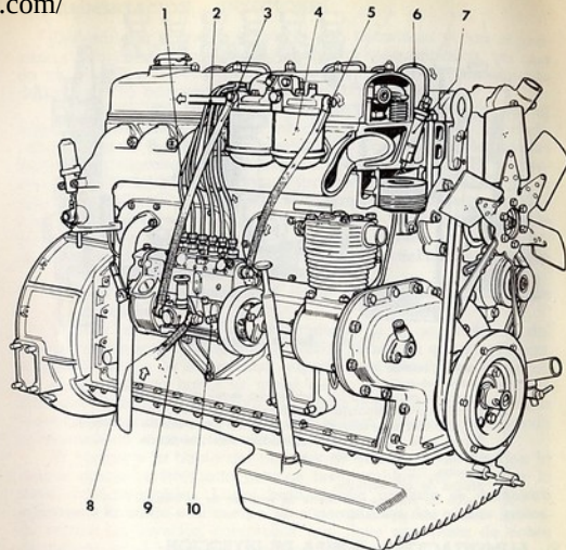
Fig. 18. - Esquema del circuito de alimentación y de inyección del combustible
