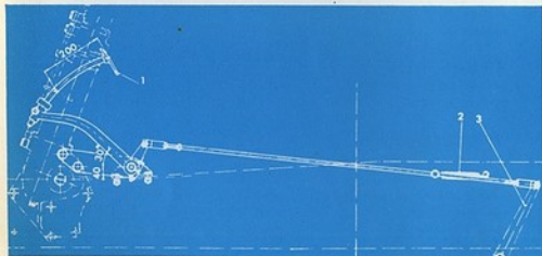
Fig. 25. - Pedal y mando exterior del embrague
