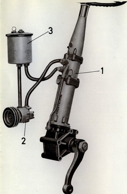
Fig. 34. - Dirección
