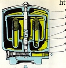
Fig. 14. - Depurador centrífugo de aceite
