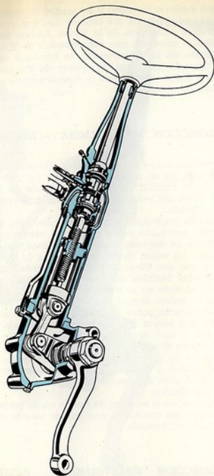
Fig. 35. - Dirección (corte longitudinal)
