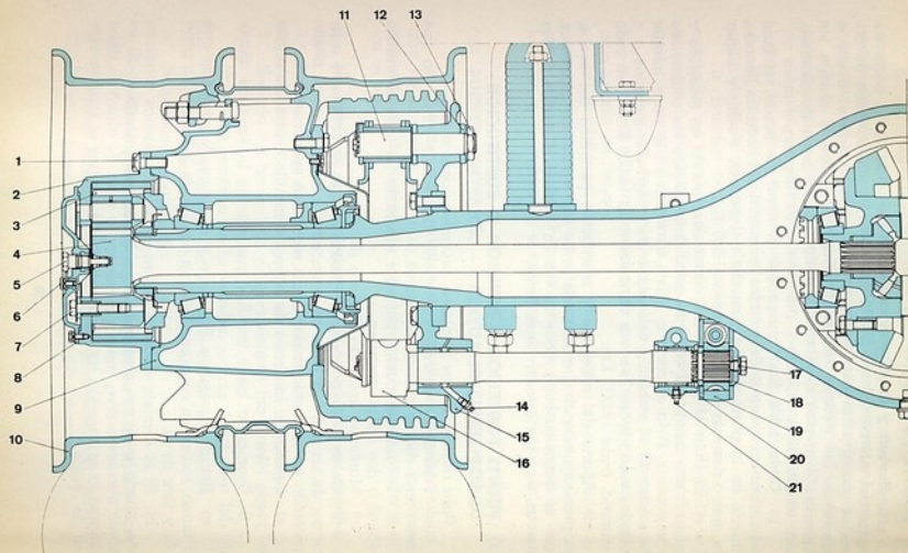
Fig. 31. - Sección del cubo y del tambor de la rueda posterior
