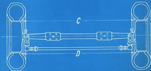
Fig. 33. - Alineación de las ruedas anteriores
