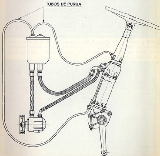
Fig. 37 bis. - Tubos de purga de la servo-dirección
