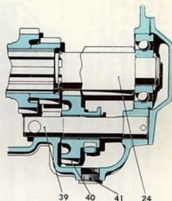
Detalle de la marcha atrás
