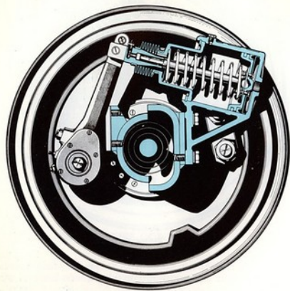
Fig. 47. - Frenos posteriores
