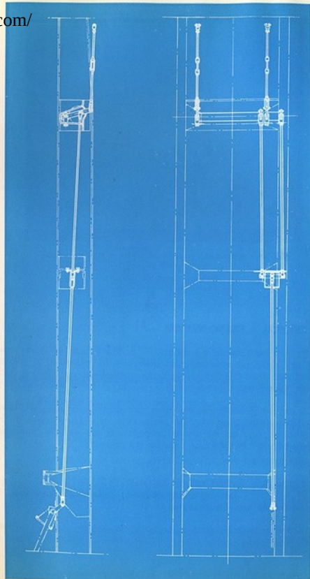
Fig. 48. - Esquema del mando mecánico del freno de mano
