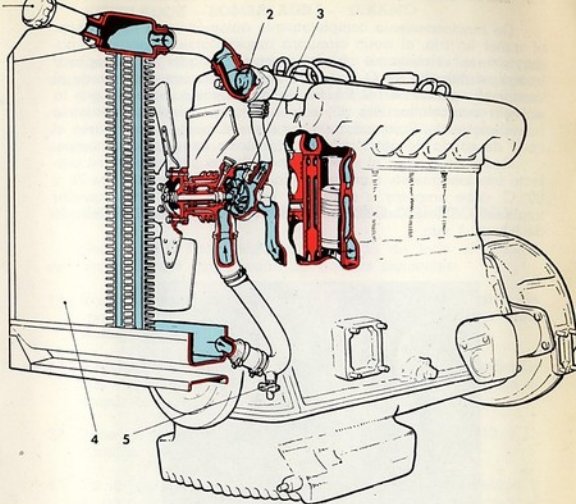
Fig. 23. - Circuito de refrigeración
