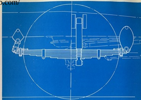
Fig. 38. - Suspensión anterior
