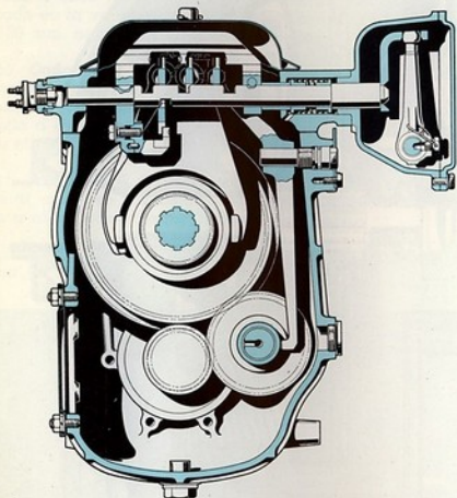
Fig. 27. - Mandos internos del cambio
