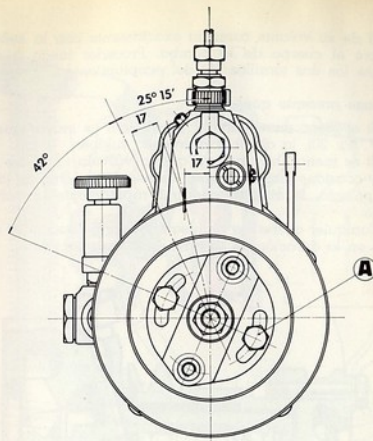
Fig. 21 bis. - Puesta en fase de la bomba de inyección
