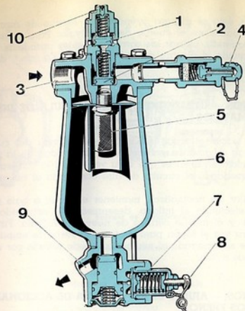
Fig. 43. - Depurador-regulador de aire
