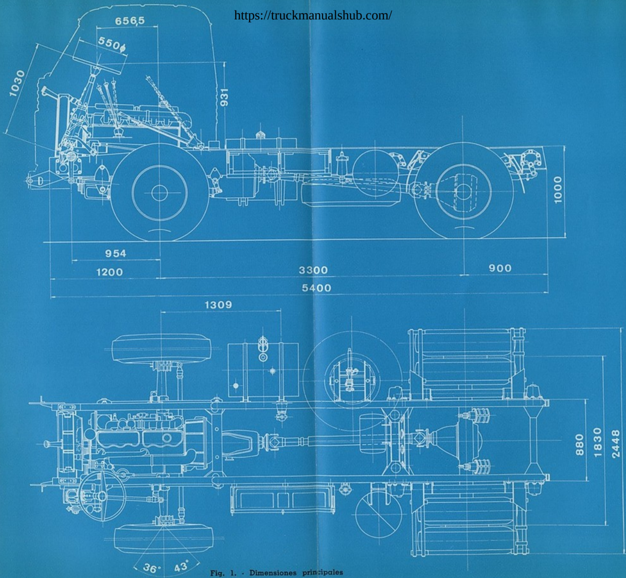
Fig. 1. - Dimensiones principales
