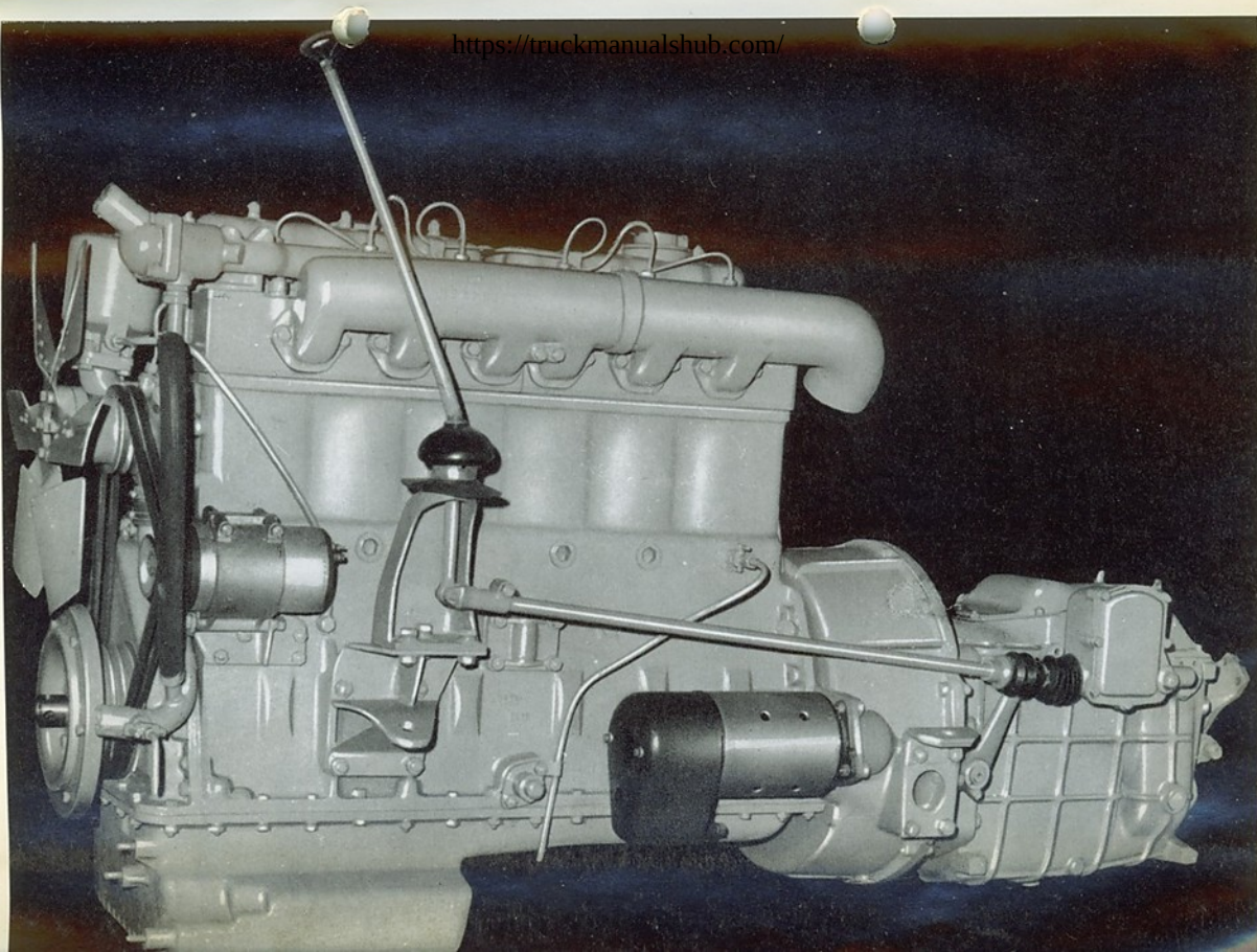
Fig. 12. - Motor, embrague y cambio (visto lado izquierdo)
