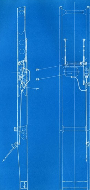
Fig. 2. - Mando servo-asistido del freno de mano
