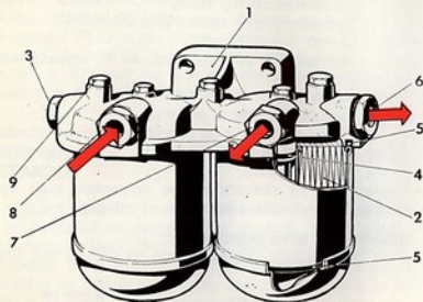
Fig. 17. - Filtro principal de combustible
