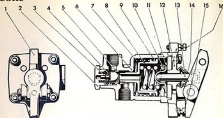
Fig. 44. - Válvula de accionamiento
