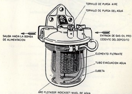
Fig. 16. - Filtro primario
