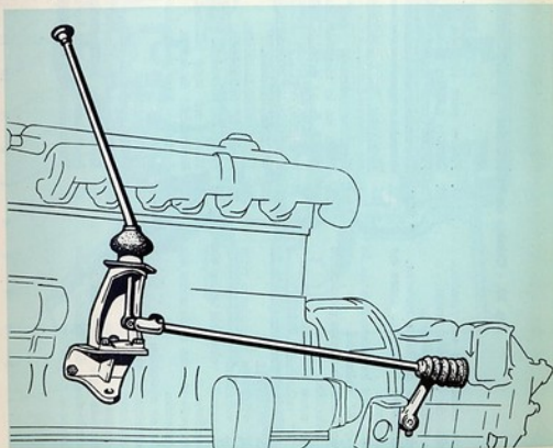
Fig. 28. - Palanca mando cambio
