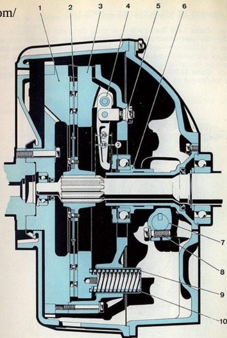
Fig. 26. - Embrague
