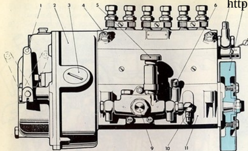
Fig. 18 bis. - Bomba de inyección
