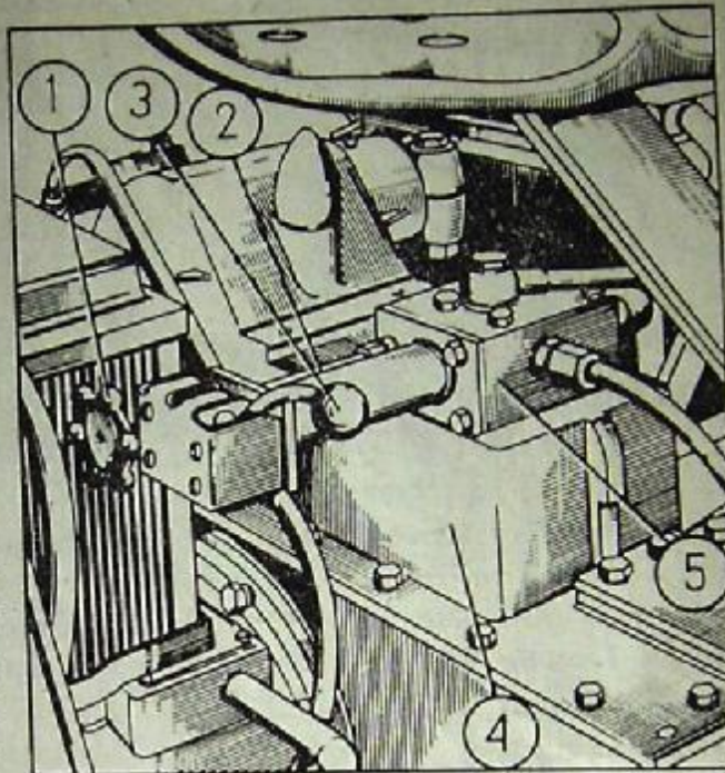
Rys. 33. Podnośnik hydrauliczny: 1 — pokrętło regulacji dociążania osi tylnej, 2 — tabliczka ze schematem położenia dźwigni (niewidoczne), 3 — dźwignia rozdzielacza podnośnika, 4 — korpus podnośnika hydraulicznego, 5 — rozdzielacz podnośnika.
