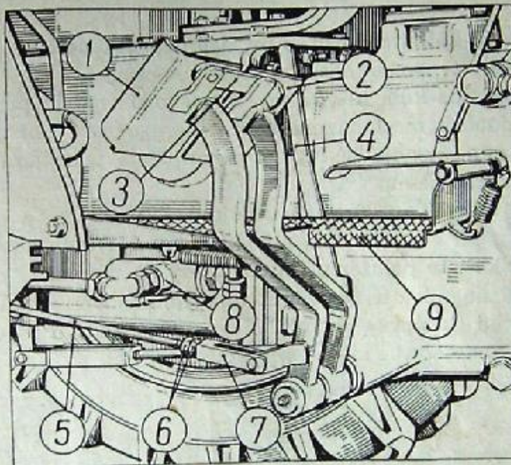
Rys. 27. Hamulce:
