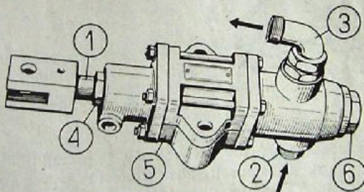
Rys. 44. Zawór hamulcowy:
