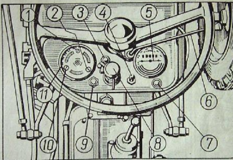
Rys. 3. Tablica rozdzielcza:
