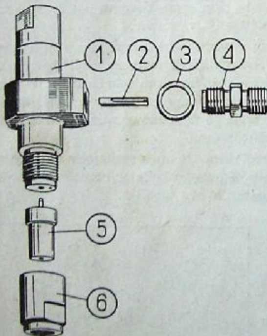
Rys. 18. Wtryskiwacz czopikowy: 1 — korpus, 2 — filtr szpilkowy, 3 — uszczelki, 4 — króciec, 5 — rozpylacz, 6 — nakrętka.
