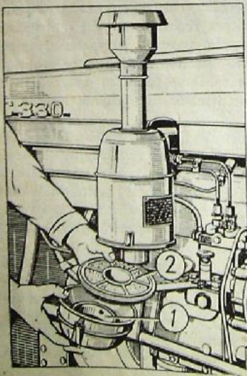
Rys. 19. Filtr powietrza: 1 — miska olejowa, 2 — sekcja wstępnego oczyszczania.
