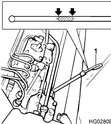
Щуп контроля уровня масла
