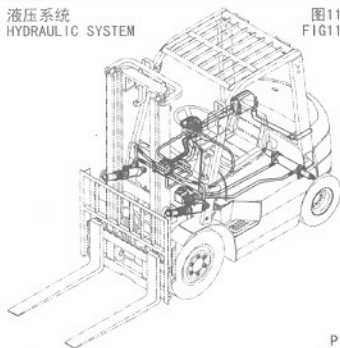
液压系统 HYDRAULIC SYSTEM
