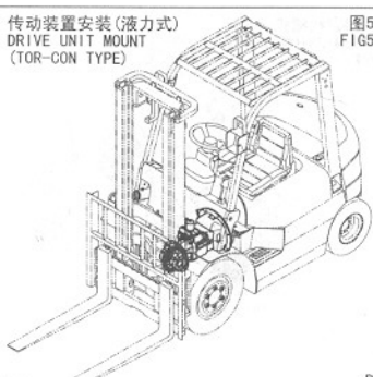
传动装置(液力式) DRIVE UNIT (TOR-CON TYPE)
