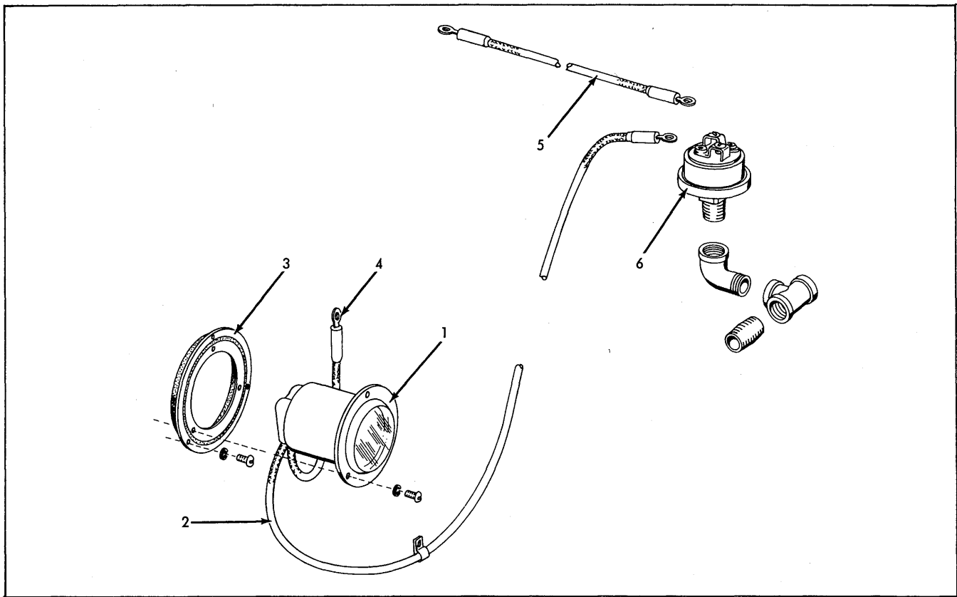
HOUR METER
