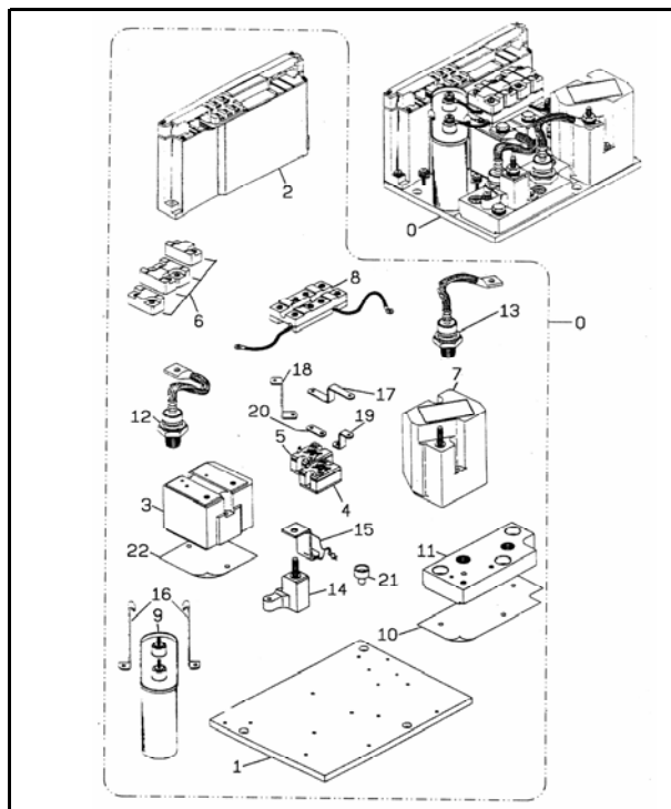
A355-1A ELECTRICAL MODULE -G.E. LTX TRACTION
