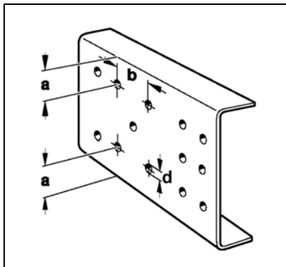
Furações na alma
