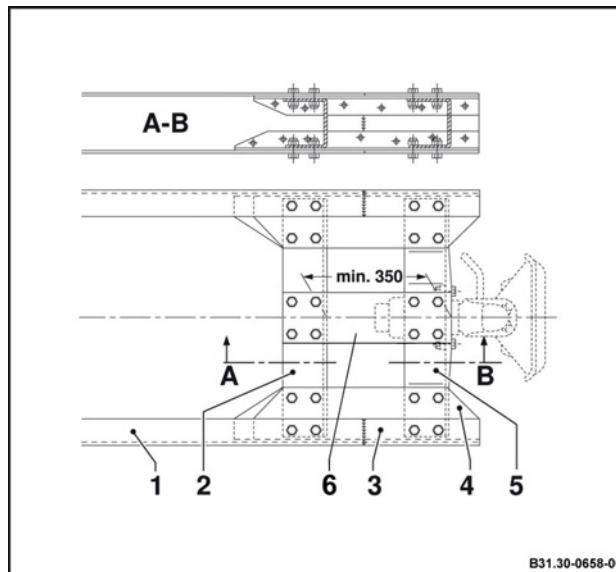
Travessa de fechamento do quadro.
