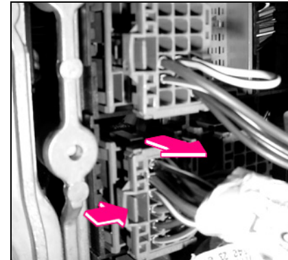
Remoção dos conectores
