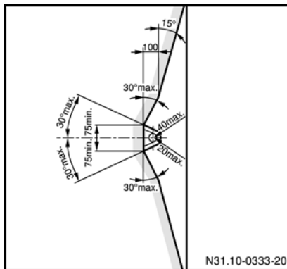
Medidas de espaço livre
