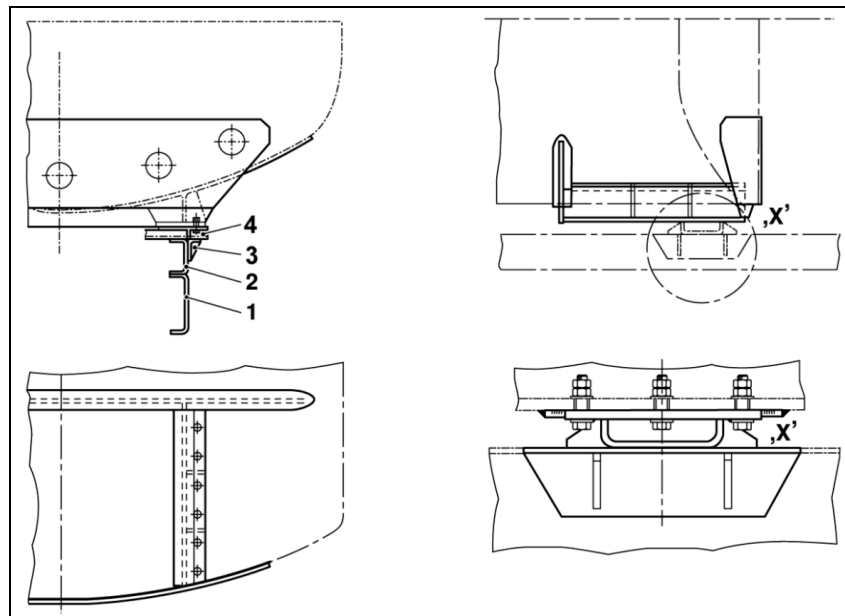
Suspensão rígida na fixação traseira
