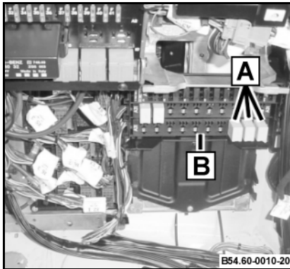
A Relés K8, K9 e K10 (A004 545 35 05)
