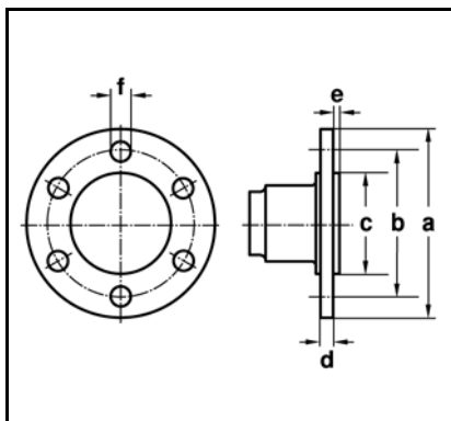
Flange de acoplamento
