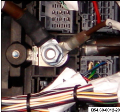
Ponto de massa na central elétrica
