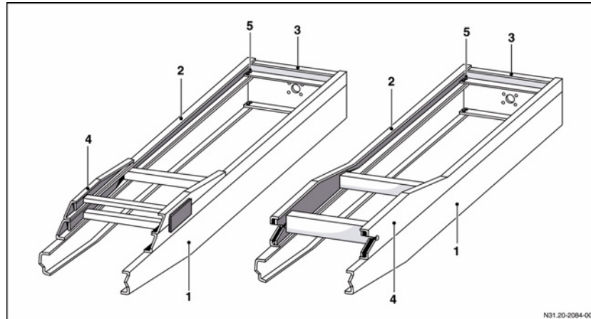
Fixação do quadro auxiliar no chassi - montagem de guindastes
