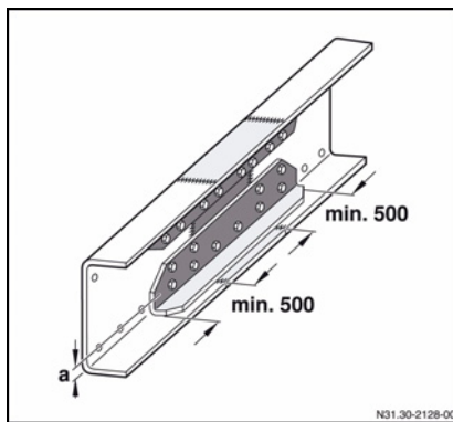
Aumento da distância entre eixos a ≥ 55mm
