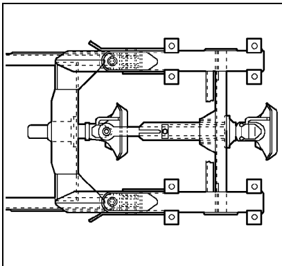
Guincho removível
