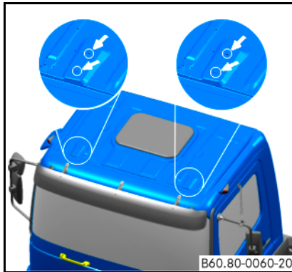
Região de fixação no teto
