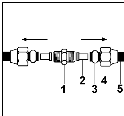
Unões de tubulações pneumáticas
