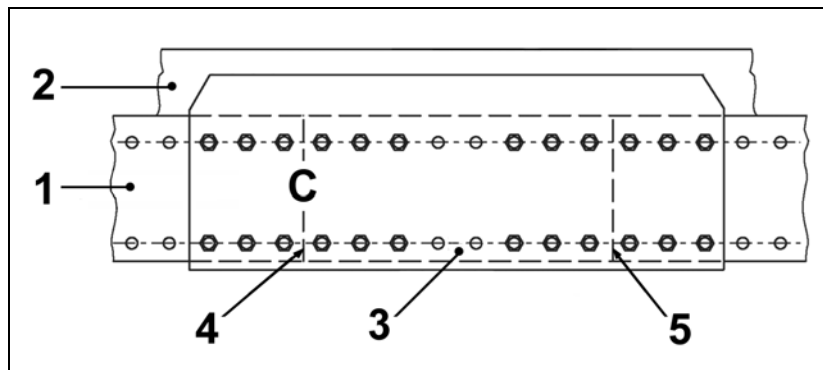
Pontos de corte na longarina do quadro
