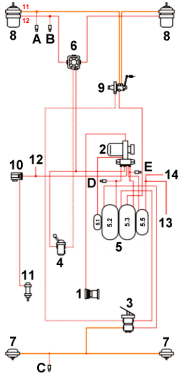
Esquema pneumático de freio (4X2)
