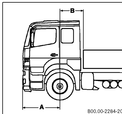
Balanço dianteiro
