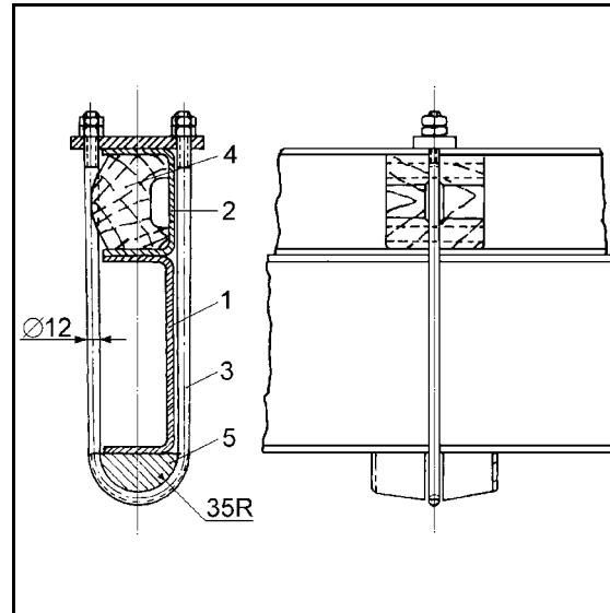
Fixação por grampos "U"
