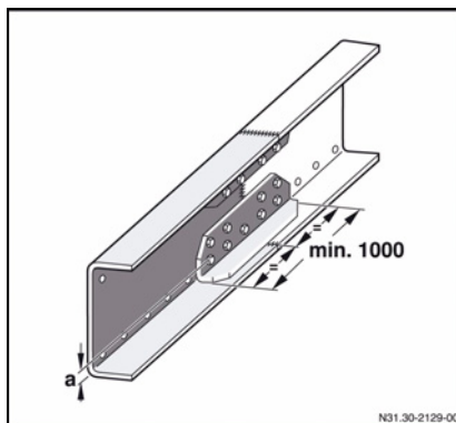
Diminuição da distância entre eixos a ≥ 55mm
