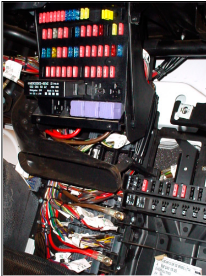
Central elétrica
