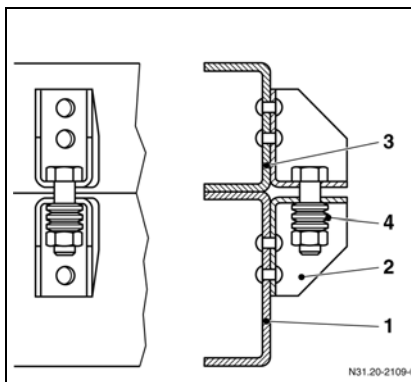
Console com elemento elástico
