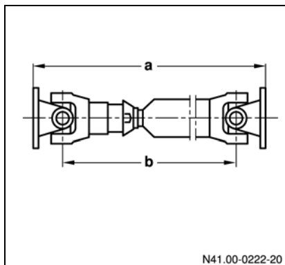
a - Comprimento da instalação b - Comprimento admissível do eixo
