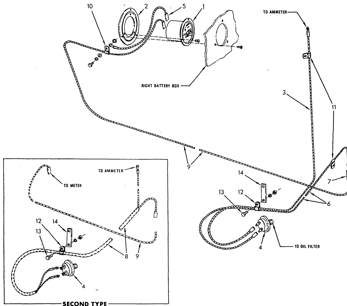
HOUR METER
