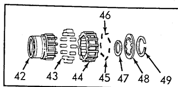
INPUT SHAFT
