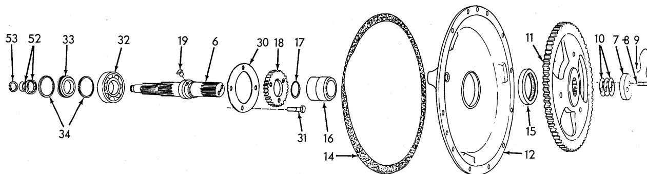
INPUT SHAFT
