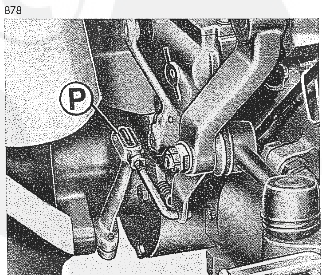
Fig. 29 - Registrazione frenatura di soccorso e stazionamento anteriore
