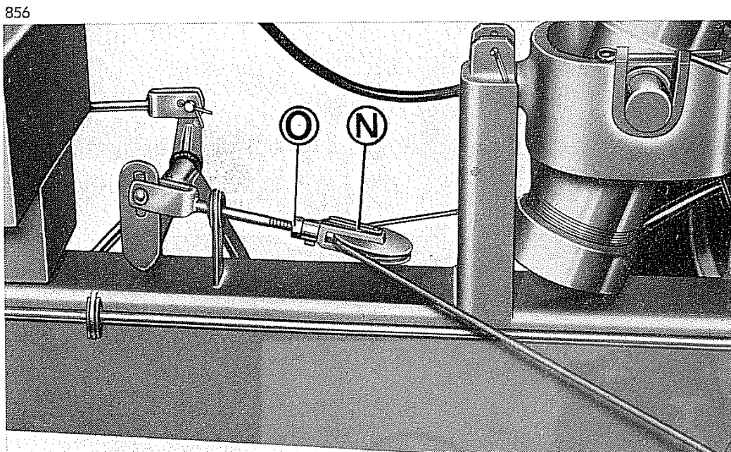
Fig. 28 - Registrazione frenatura di soccorso e stazionamento posteriore
