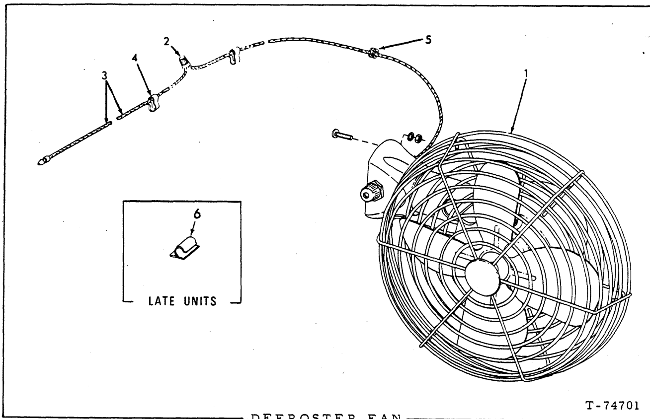
DEFROSTER FAN
