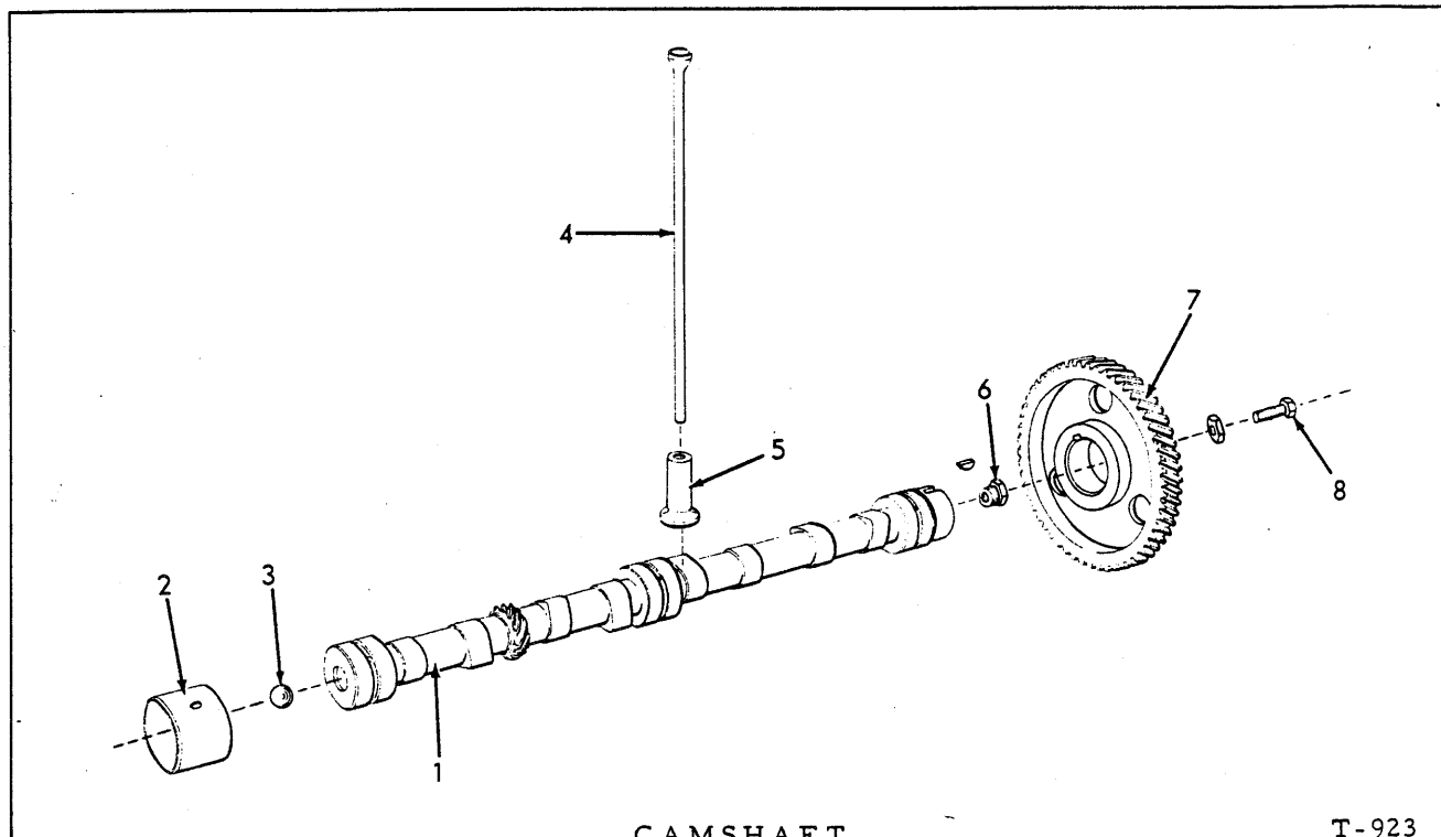
CAMSHAFT
