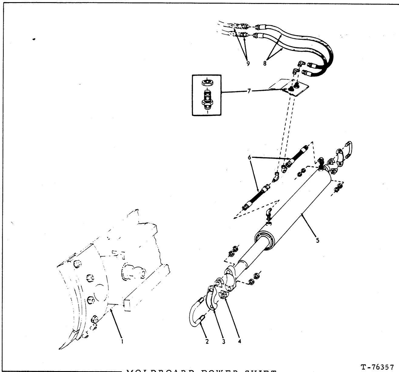
MOLDBOARD POWER SHIFT
