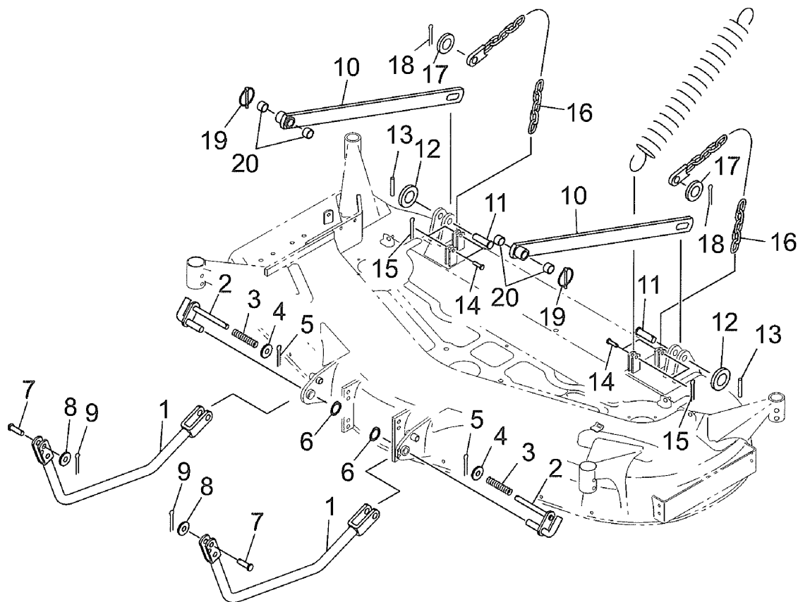
リンク FIG.302 LINK
