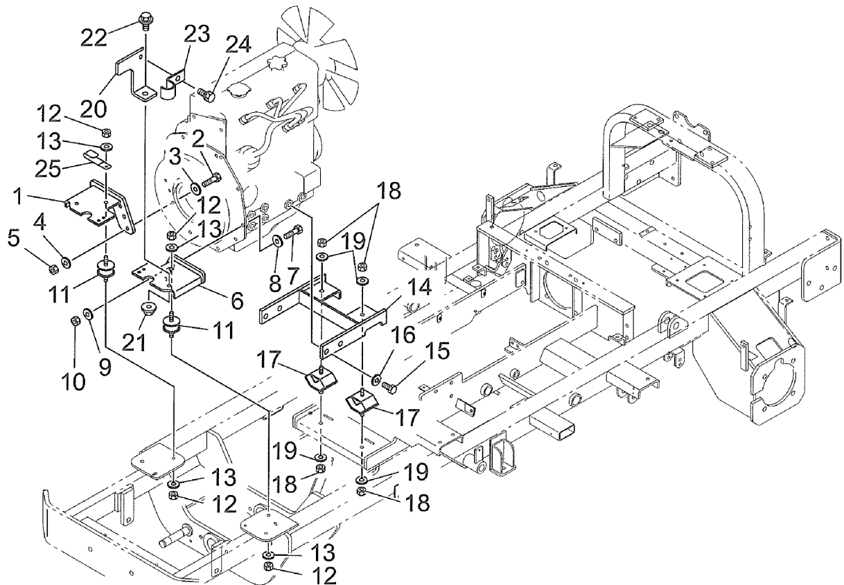
https://truckmanualshib.com/ エンジンマウント FIG.204 ENGINE MOUNT
