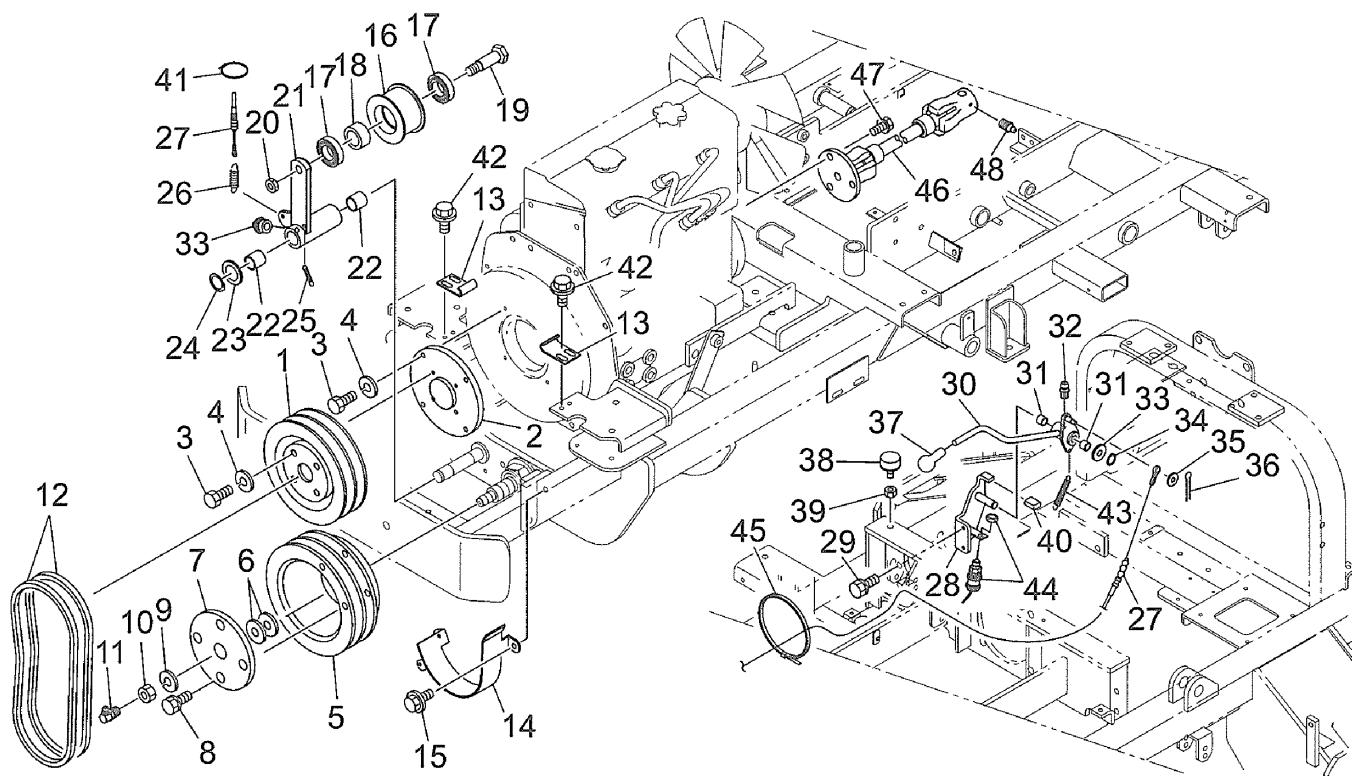
FRONT P.T.O
