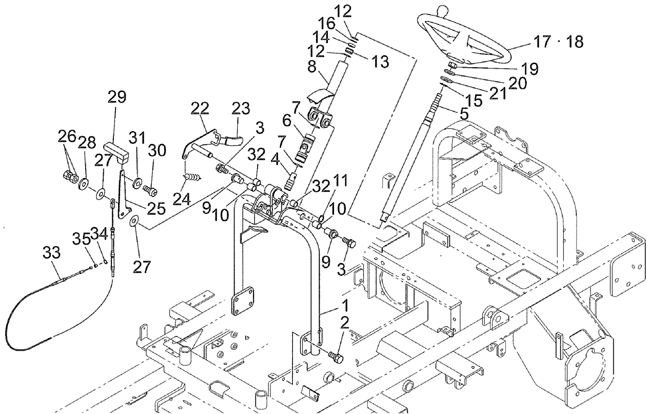
ステアリング FIG.207 STEERING
