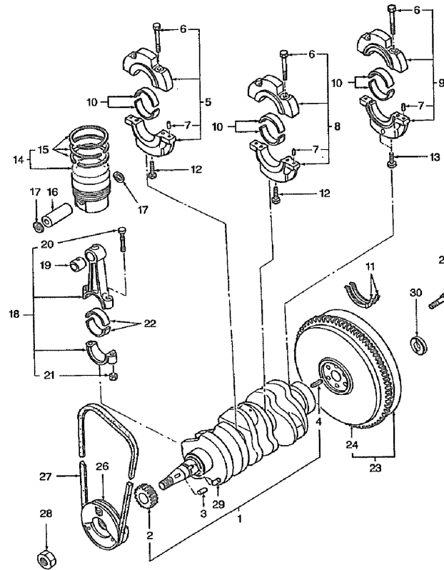
FIG.104 クランクシャフト、ピストン CRANKSHAFT,PISTON
