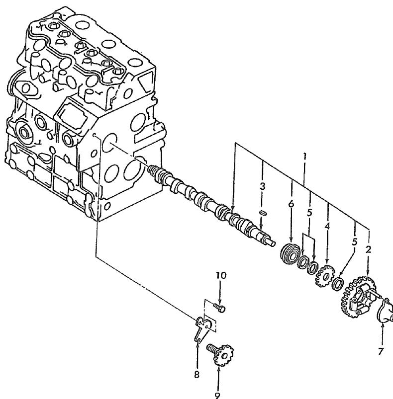
CAMSHAFT
