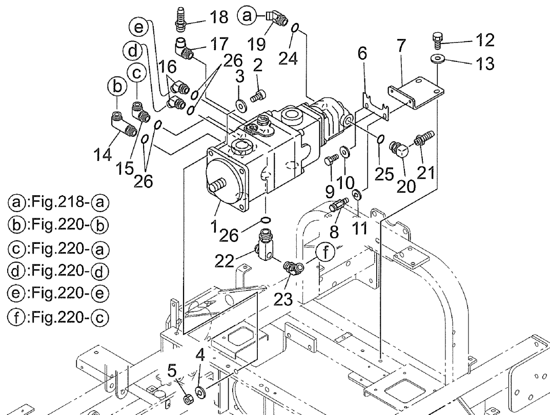
https://truckmanuals.com/ エフ/人(H.S.T) FIG.222 HYDRAULIC(H.S.T)
