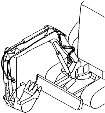
Fig.98 油圧配管 (テレスコピックアーム:ブーム) HYD. OIL PIPING (TELESCOPIC ARM:BOOM)
