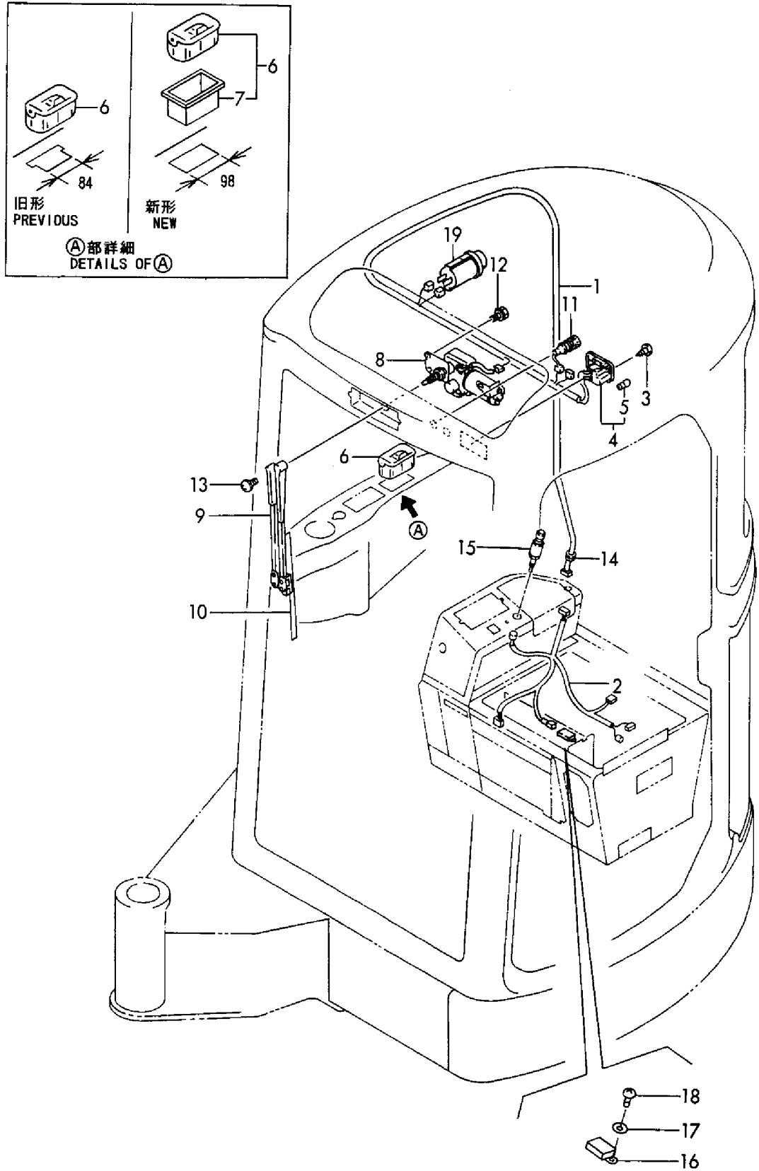
Fig. 27 電装品(キャビン専用) ELECTRIC PART(CABIN)
