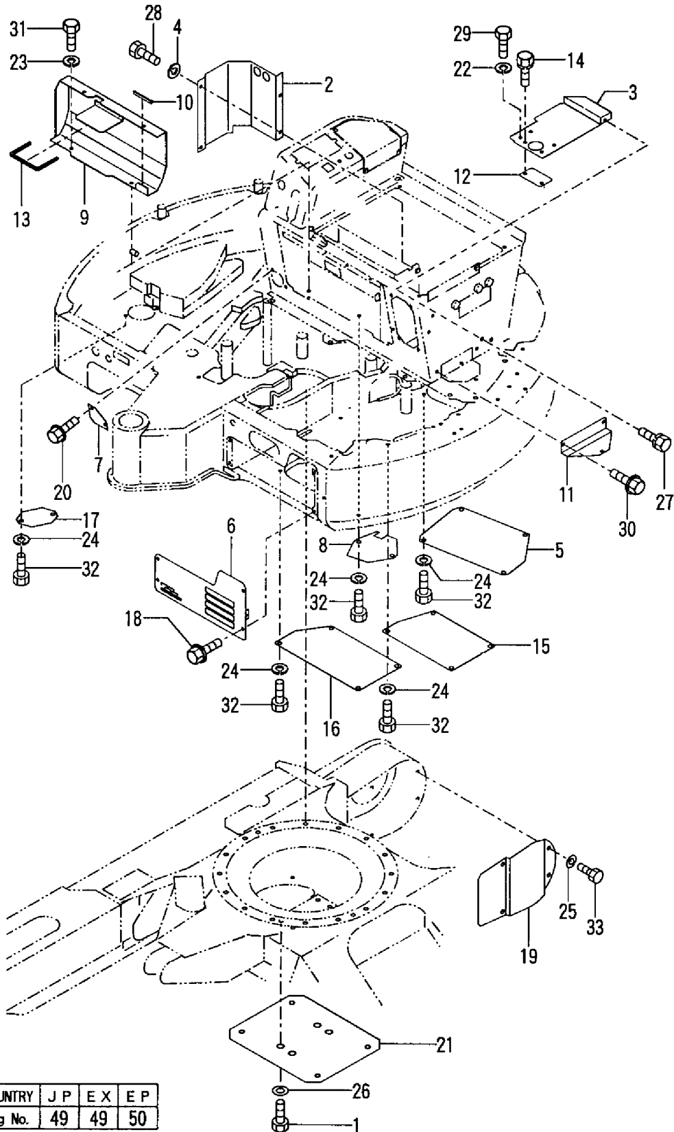
Fig. 50 フレームカバー(キャビン仕様)(EP) FRAME COVER(CABIN SPEC.)(EP)
