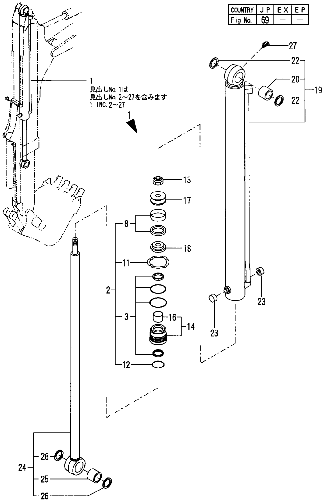
Fig. 69 スライドシリンダ(テレスコピックアーム仕様) SLIDE CYLINDER(TELESCOPIC ARM SPEC.)
