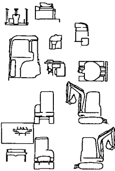
Fig.2 銘板(キャビン:JP)(新形:PL仕様) LABEL(CABIN:JP)(NEW :PL SPEC.)
