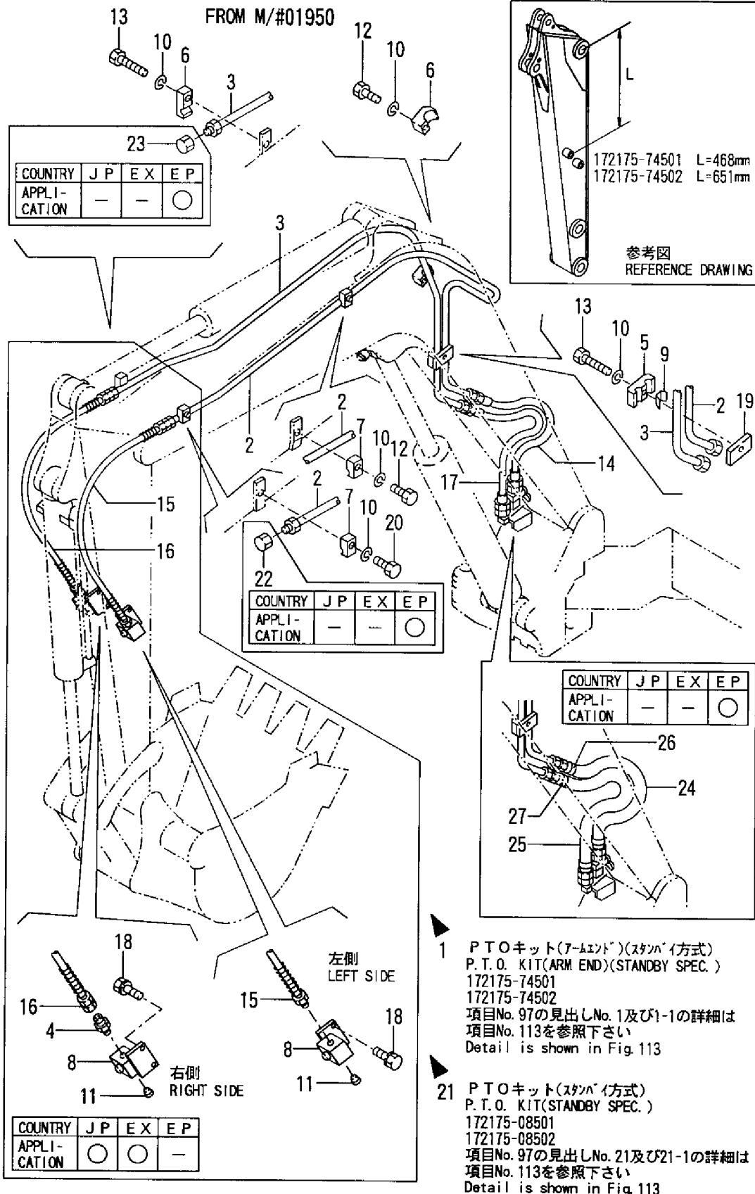
Fig. 97 油圧配管(PTO7-メント)(新形) HYD. OIL PIPING(P. T. O. ARM END)(NEW)
