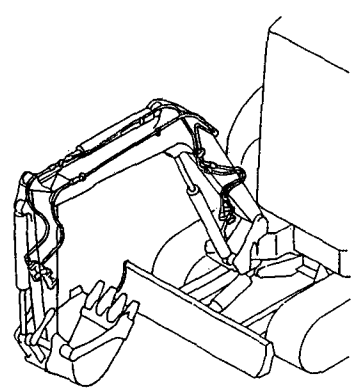
Fig. 96 油圧配管(PTOアームエンド)(旧形) HYD. OIL PIPING (P. T. O. ARM END)(PREVIOUS)
