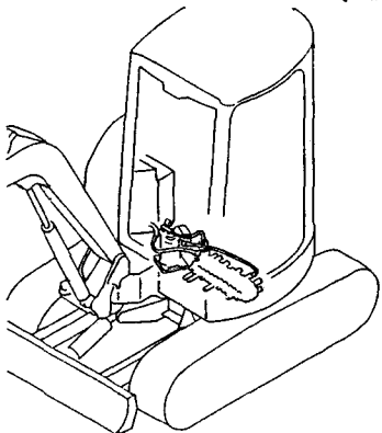
Fig. 92 油圧配管(リターン)(新形) HYD. OIL PIPING(RETURN) (NEW)
