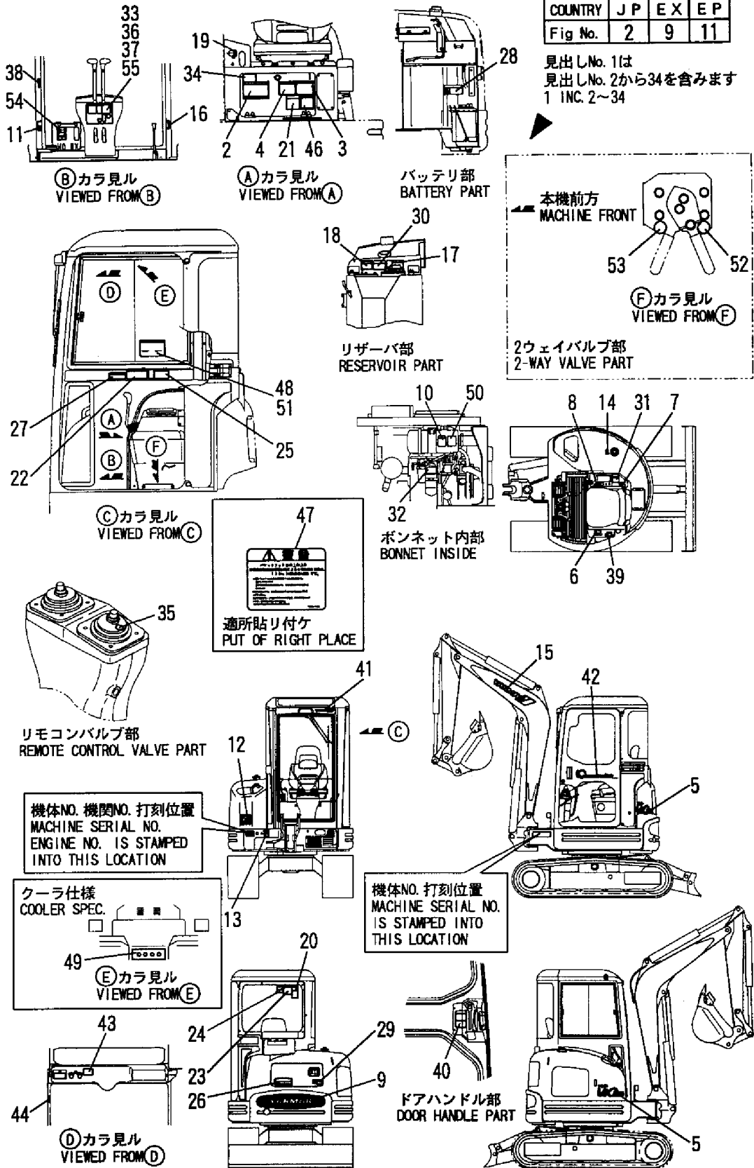
Fig. 2 銘板(キャビン:JP)(新形:PL仕様) LABEL(CABIN:JP)(NEW:PL SPEC.)
