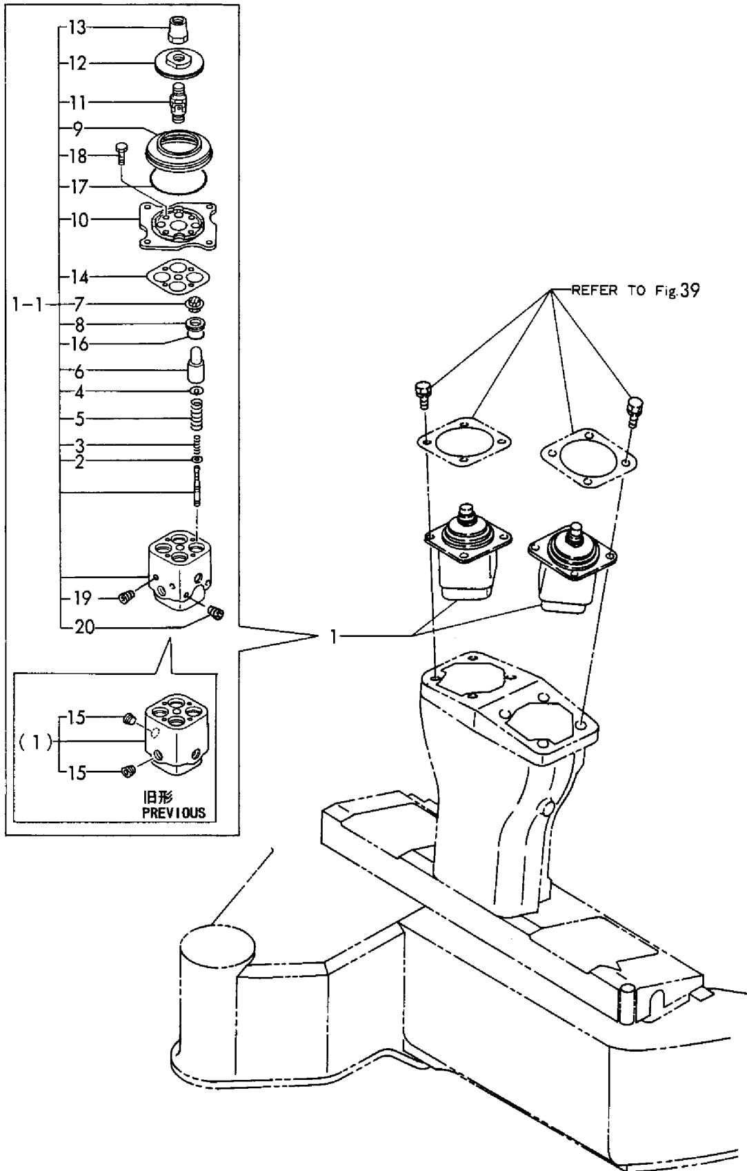
リモコンバルブ REMOTE CONTROL VALVE Fig. 80
