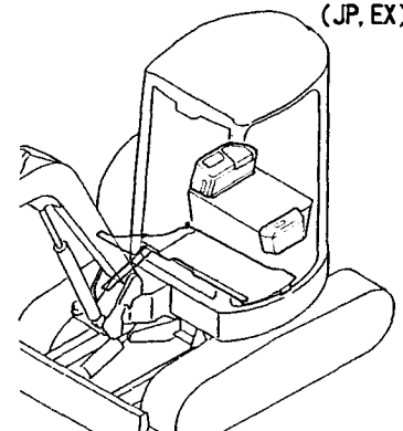
Fig.52 ステップ & インパネ (JP, EX) STEP & INSTRUMENT PANEL (JP, EX)
