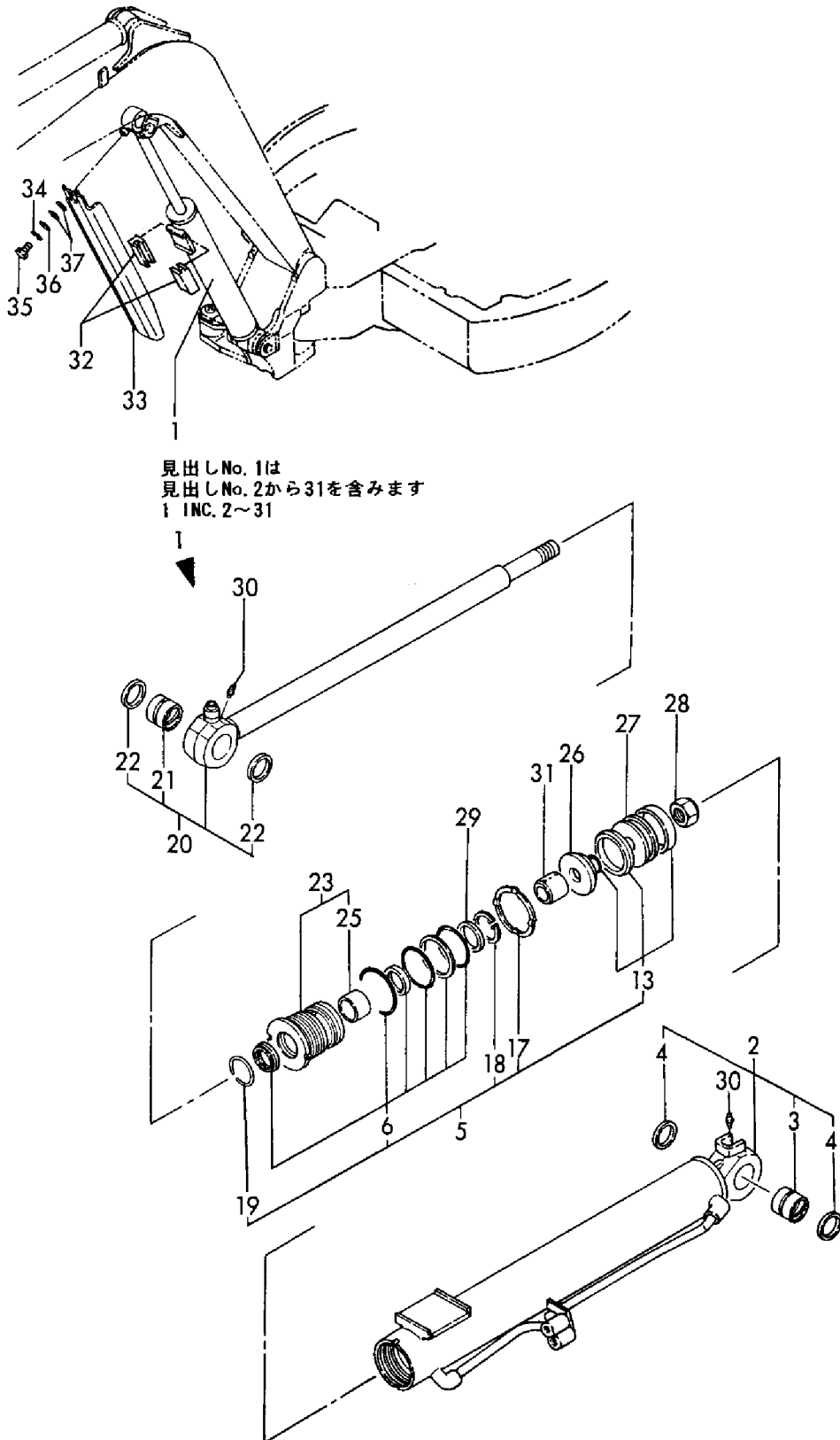
Fig. 66 ブームシリンダ(キャビン) BOOM CYLINDER(CABIN)
