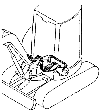
Fig. 88 油圧配管(ポンプ, バルブ ～モータ, ブーム) HYD. OIL PIPING(PUMP, VALVE ~MOTOR, BOOM)
