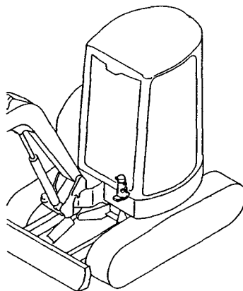
Fig. 78 コントロールバルブ(1/2) CONTROL VALVE(1/2)
