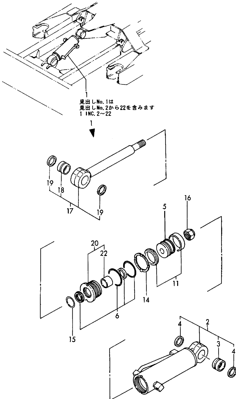
Fig. 73 ブレードシリンダ BLADE CYLINDER
