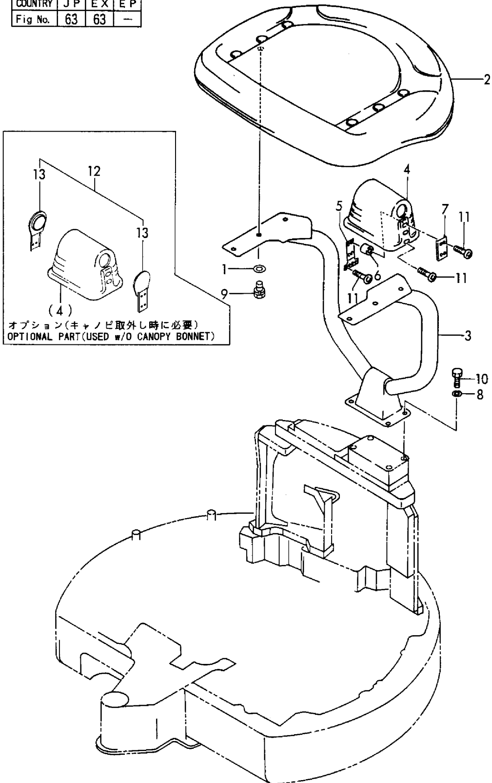
Fig. 63 キャノピ CANOPY
