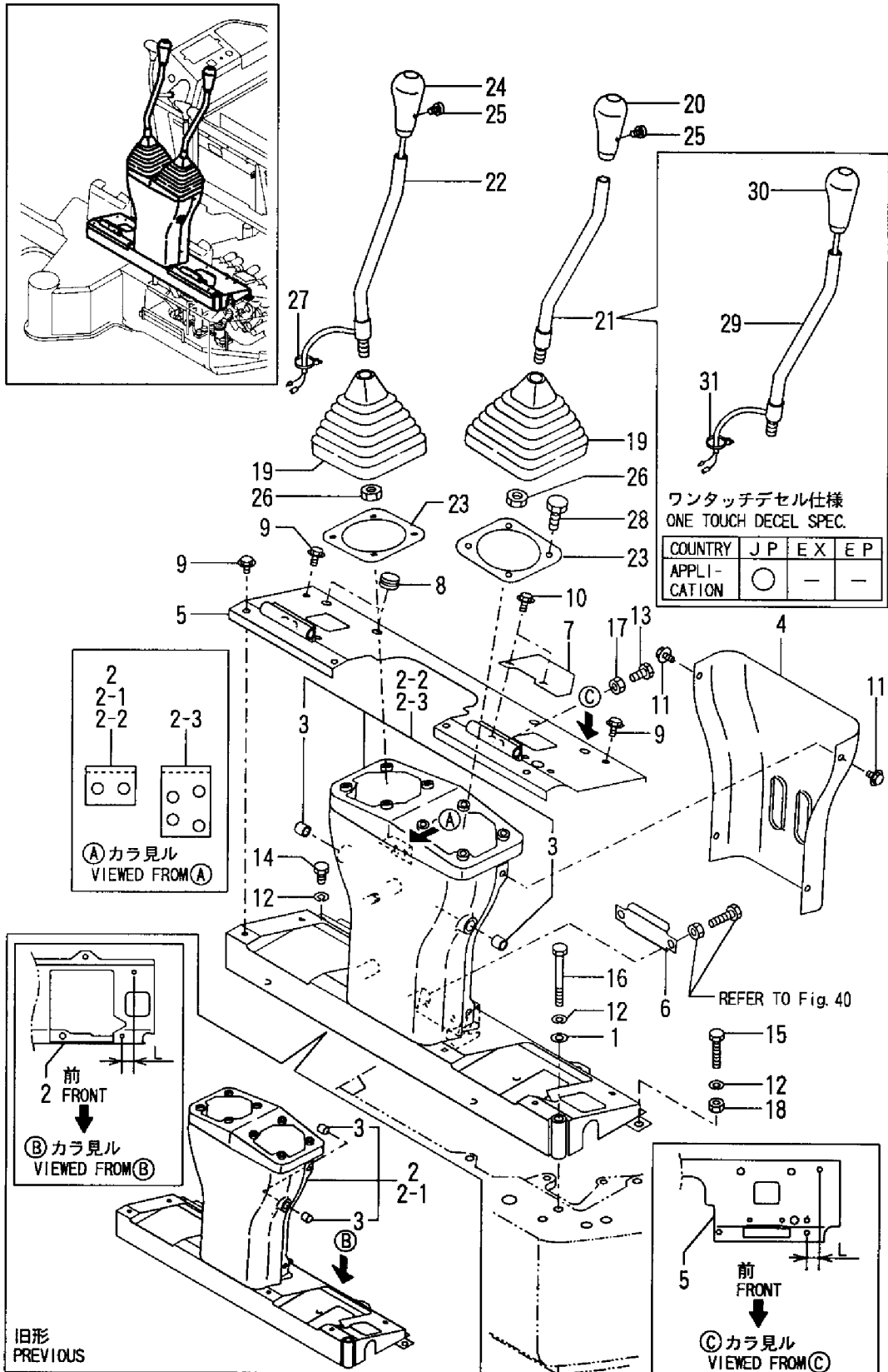
Fig. 39 39 操縦装置(作業レバー & スタンド) CONTROL EQUIPMENT(OPERATION LEVER & STAND)
