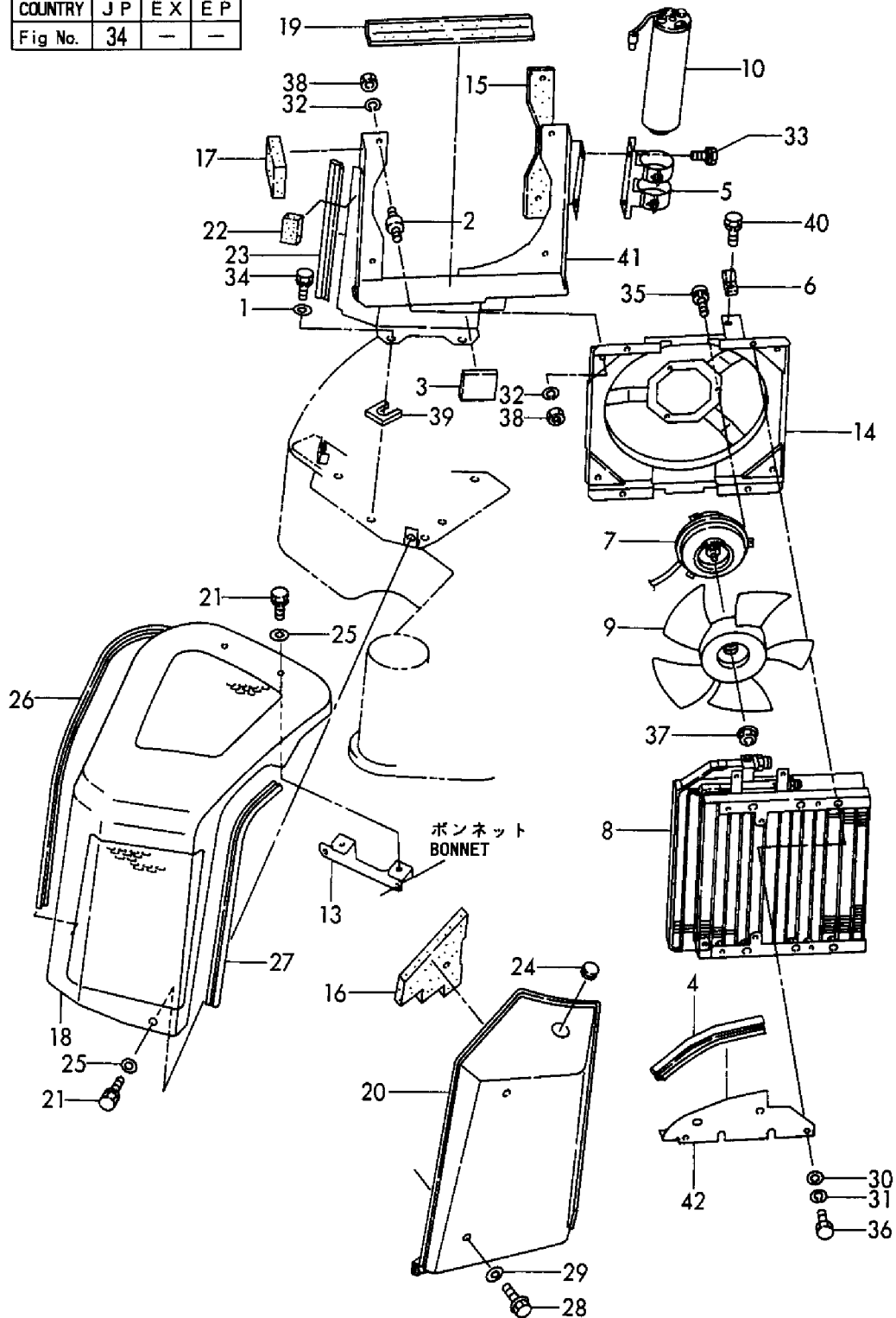
Fig. 34 クーラ(コンデナシ関連) COOLER(CONDENSER RELATED)
