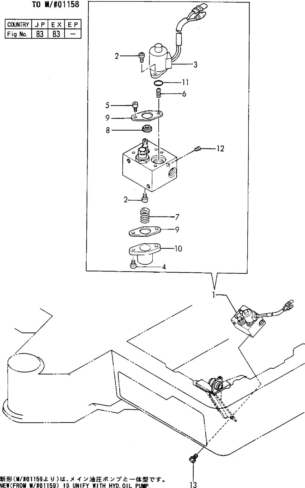
Fig. 83 ローハイバルブ(旧形) LOW-HIGH VALVE(PREVIOUS)
