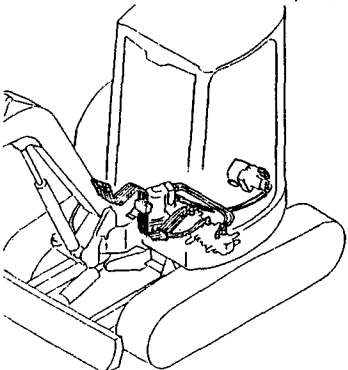
Fig. 88 油圧配管(ポンプ, バルブ ～モータ, ブーム) HYD. OIL PIPING(PUMP, VALVE ~MOTOR, BOOM)
