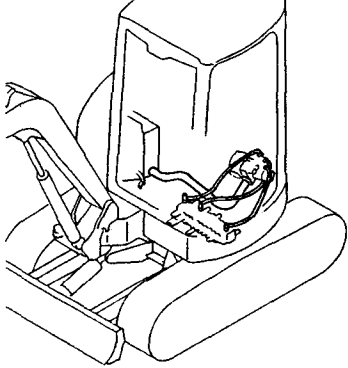
Fig. 87 油圧配管(バルブ～モータ, ～ブーム) HYD. OIL PIPING(VALVE ~MOTOR, BOOM)
