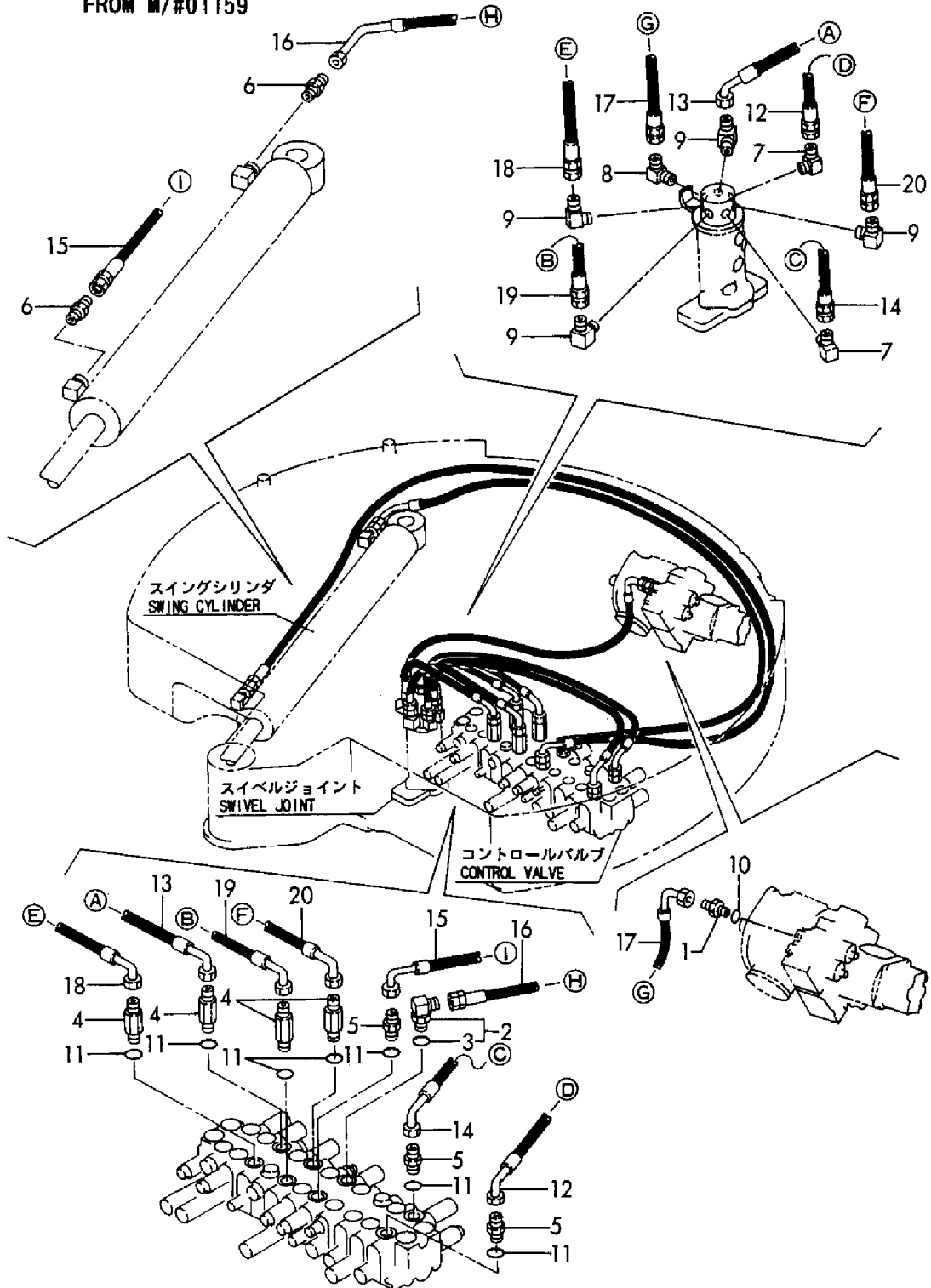
Fig. 90 油圧配管(バルブ～スィベル, スイング)(新形) HYD. OIL PIPING (VALVE ~ SWIVEL, SWING) (NEW)
