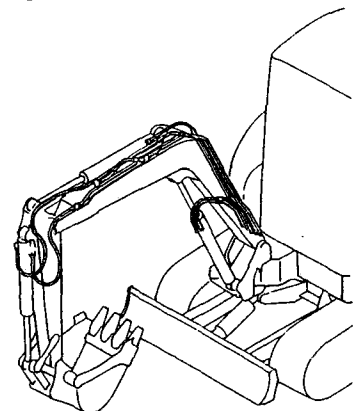
Fig. 96 油圧配管(PTOアームエンド)(旧形) HYD. OIL PIPING (P. T. O. ARM END)(PREVIOUS)
