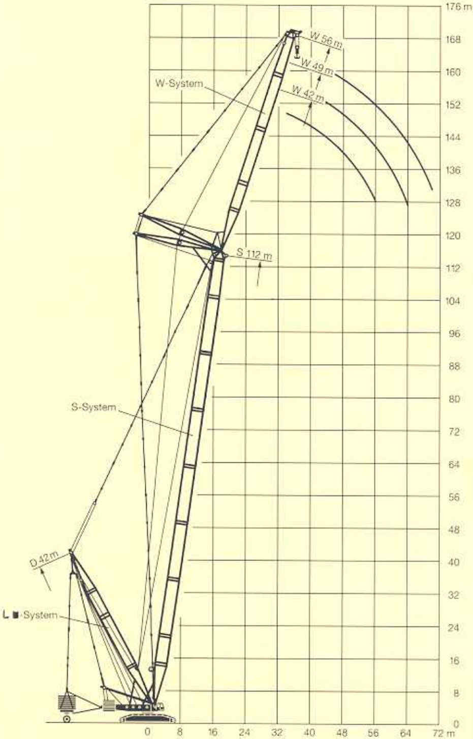
S-Ausleger / S boom / Flèche principale S: 82°
