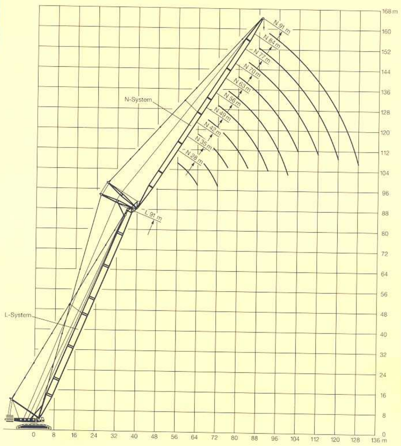
L-Ausleger / L boom / Flèche principale L: 67°
