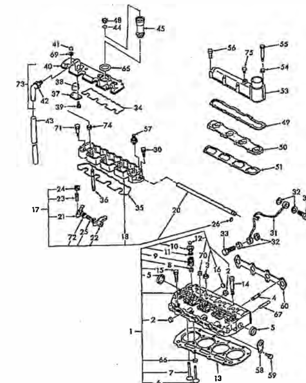
FIG.103 シリンダヘッド、ロッカアーム/CYLINDER HEAD, ROCKER ARM
