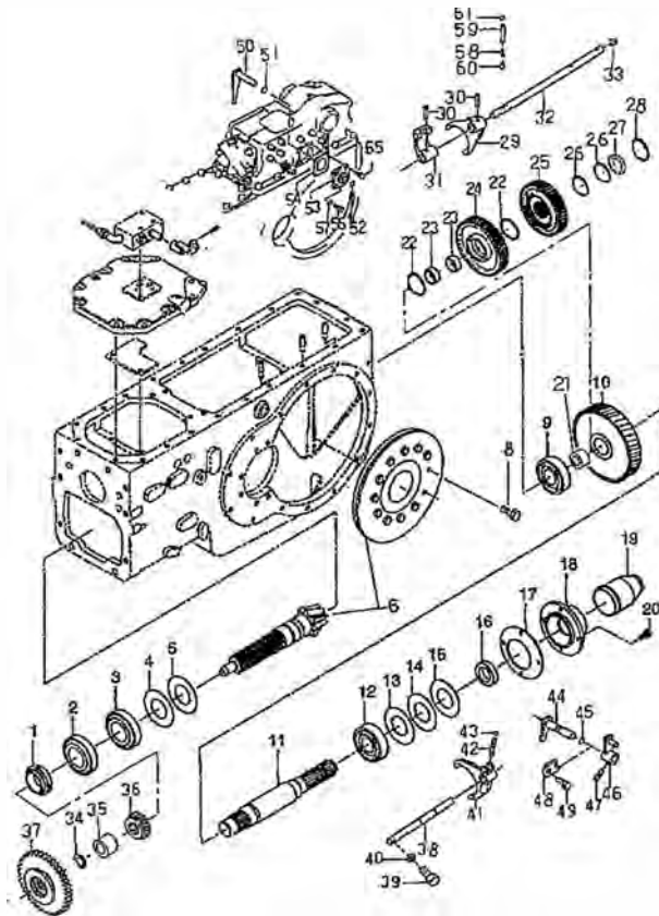
FIG.212 リヤトランスミッション ; PTO/REAR TRANS MISSION ; PTO
