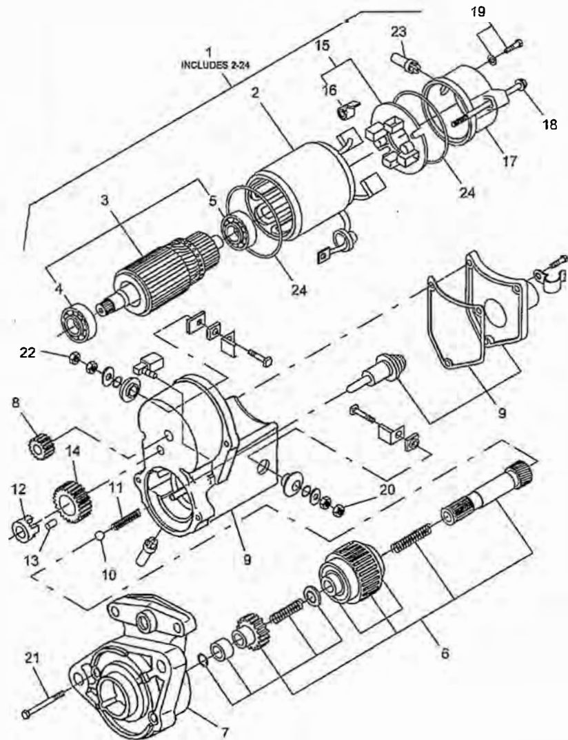
FIG.111 スターティングモーター/STARTING MOTOR
