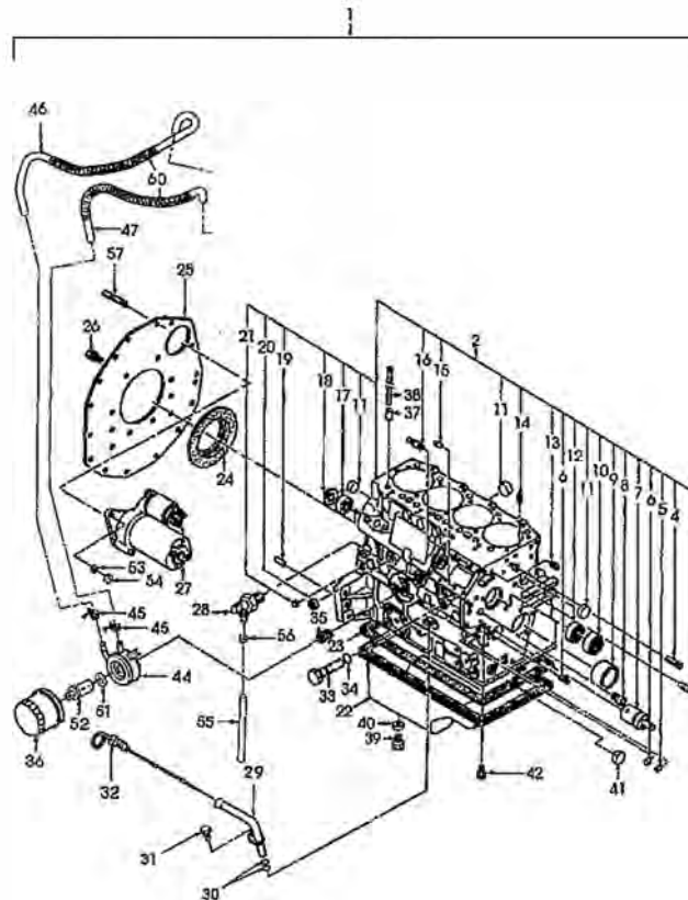
FIG.102 シリンダブロック/CYLINDER BLOCK
