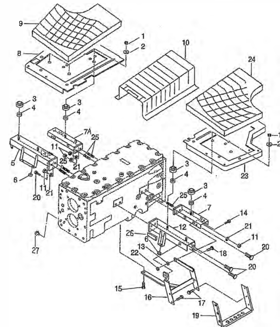
FIG.219 ステップ/STEP
