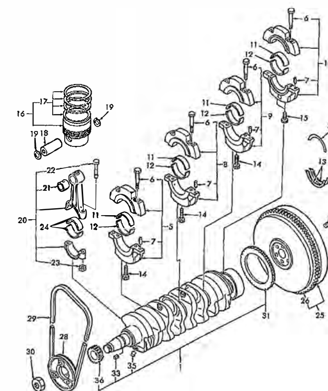
FIG.104 クランクシャフト &amp; ピストン／CRANKSHAFT &amp; PISTON
