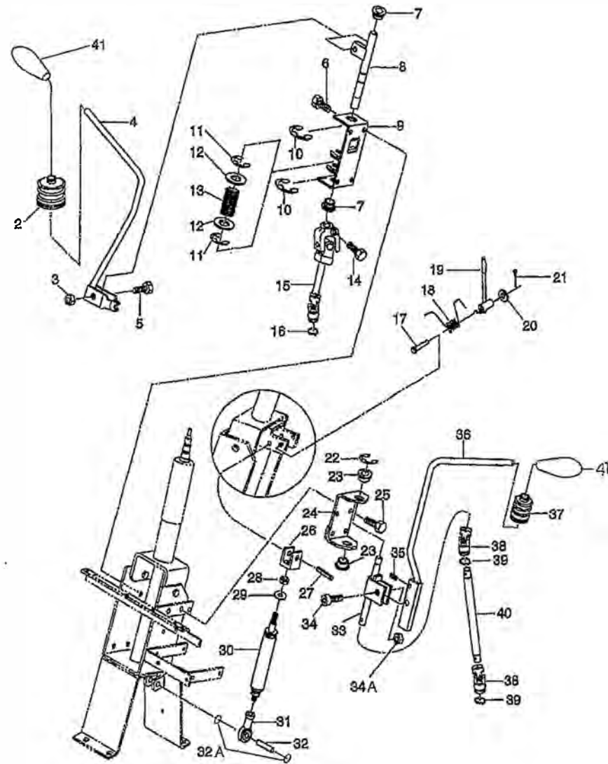
FIG.215 コラムシフト、チルト/テレスコ/COLUM SHIFT & TILT/TELE SCORPING
