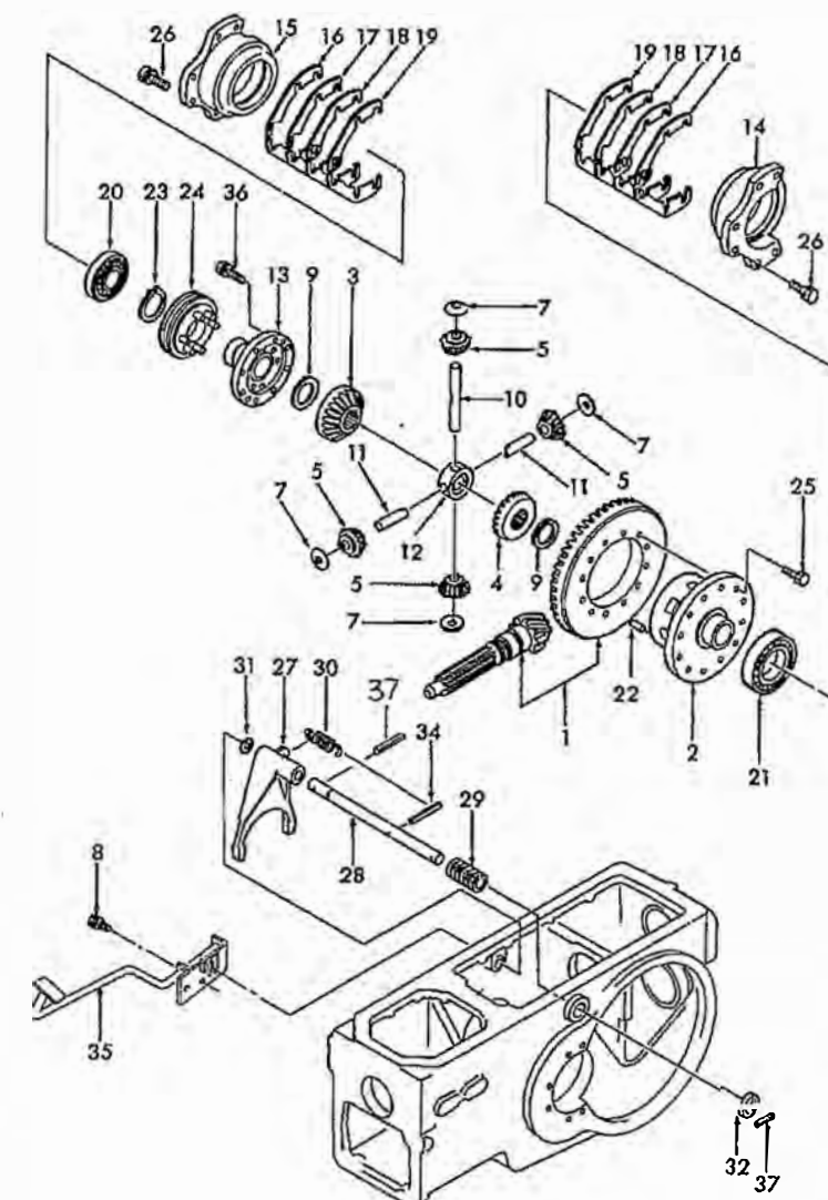
FIG.213 リヤトランスミッション；デフ／REAR TRANS MISSION；DIFF
