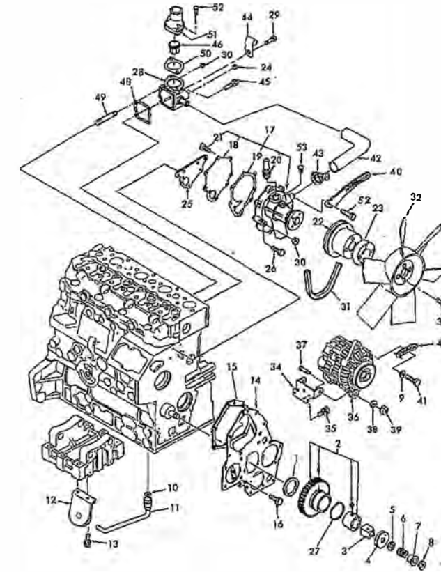
FIG.107 オイルポンプ、ウォーターポンプ、ファン/OILPUMP, WATER PUMP, FAN
