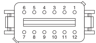
MCU J5 (Brown)
