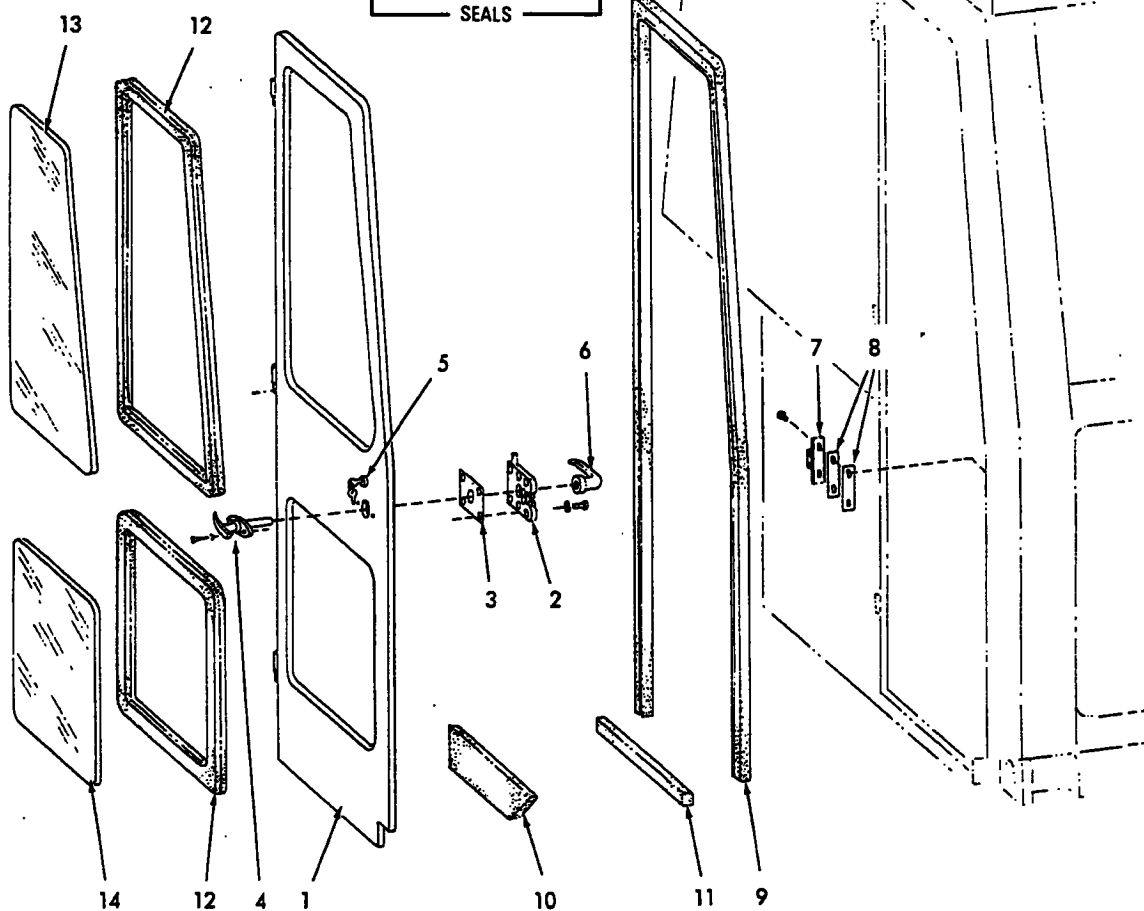
CAB DOOR
