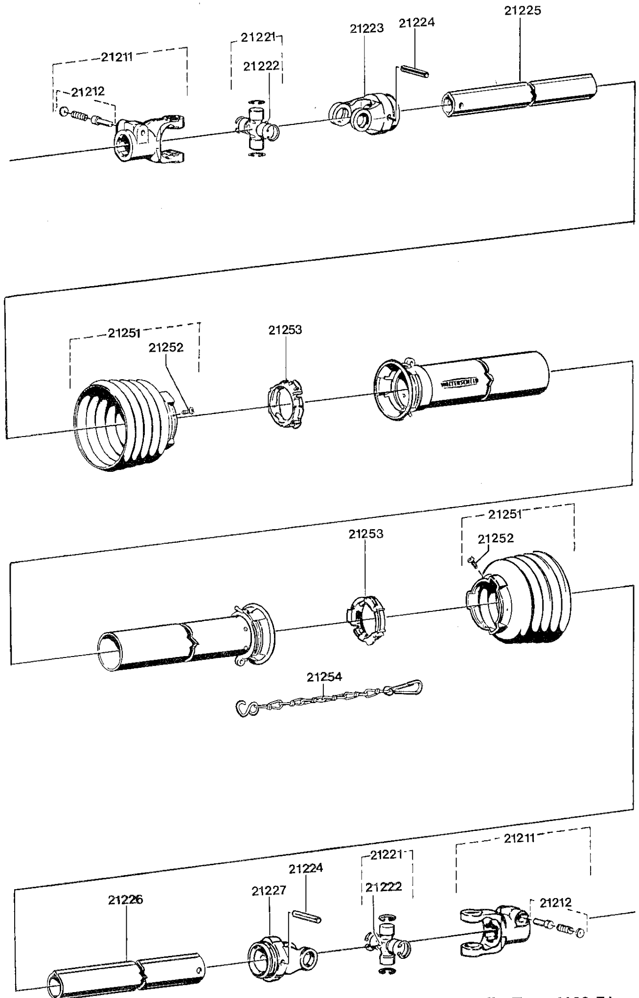
Gelenkwelle Type 4169-71 für C 500 Bildtafel - table - No. 232
