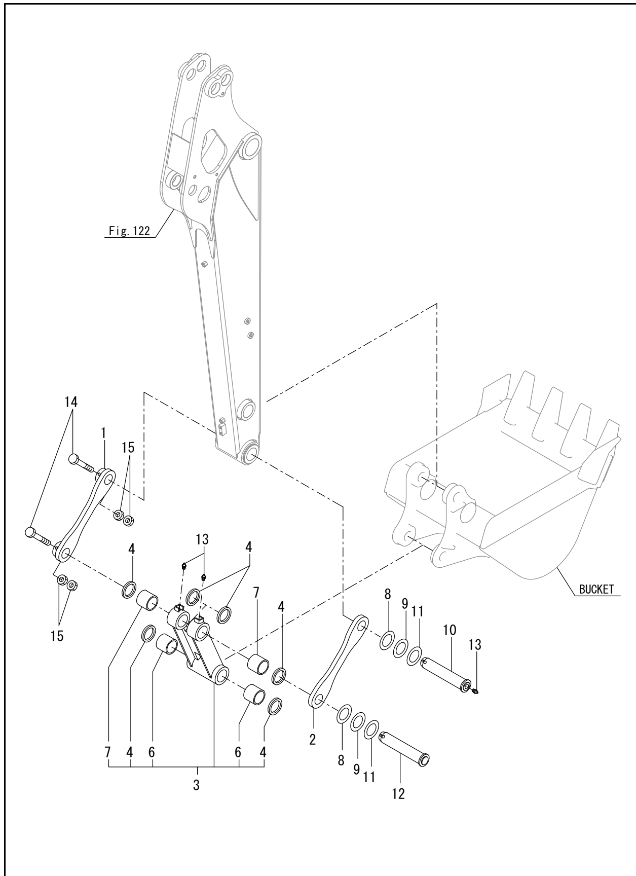
FIG. 124 - BUCKET ARM & LINK
