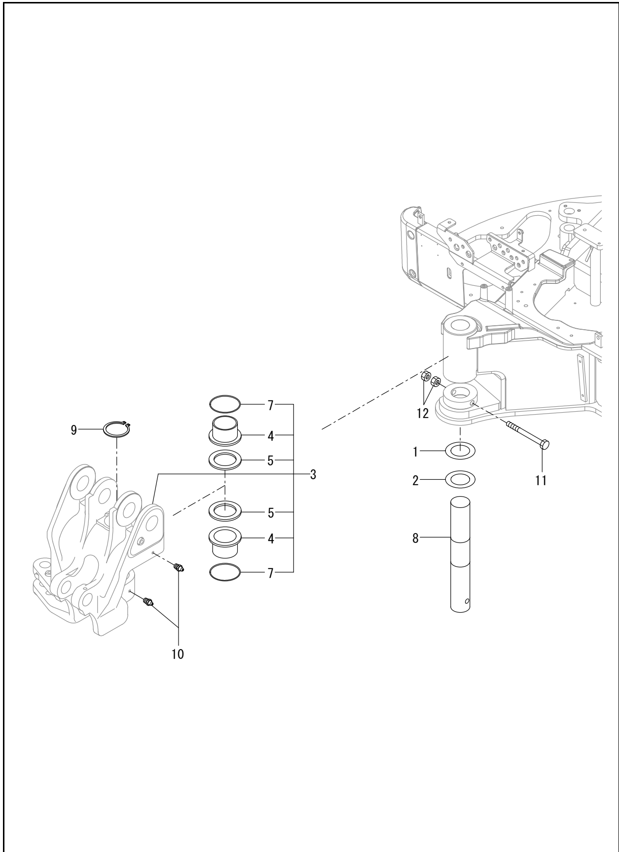
FIG. 118 - BOOM BRACKET
