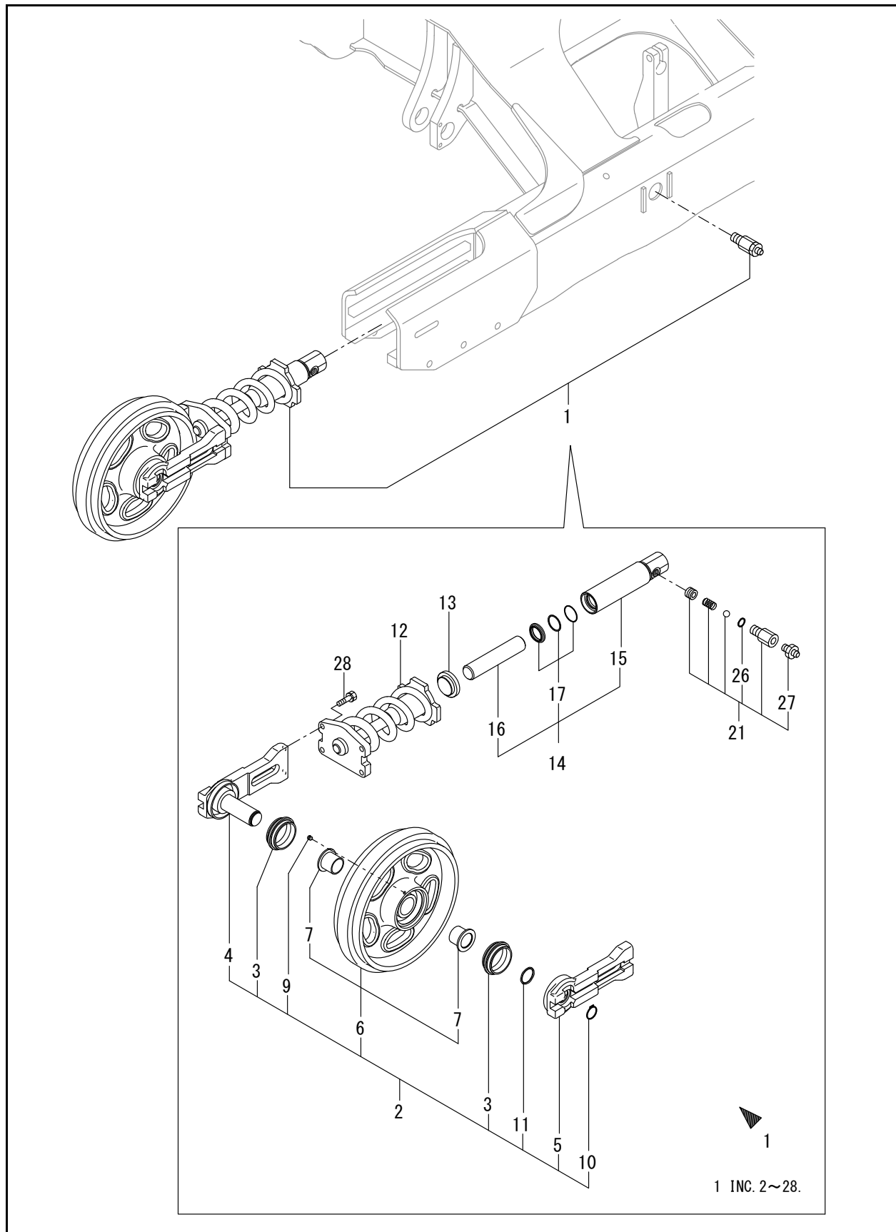
FIG. 31 - IDLER & ADJUST
