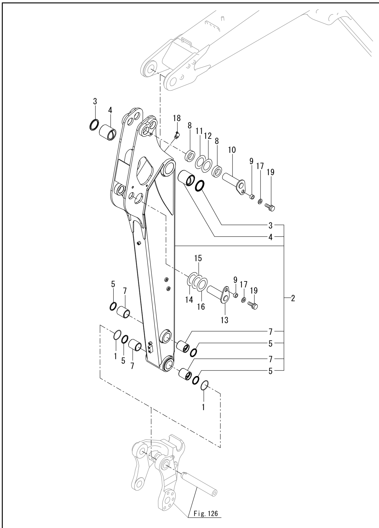
FIG. 122 - ARM
