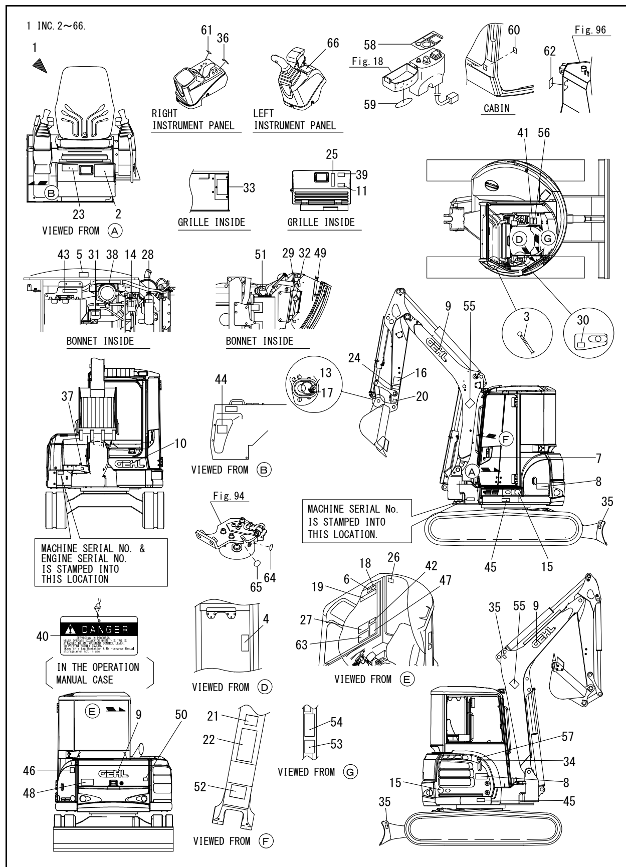
FIG. 2 - LABEL (CABIN)
