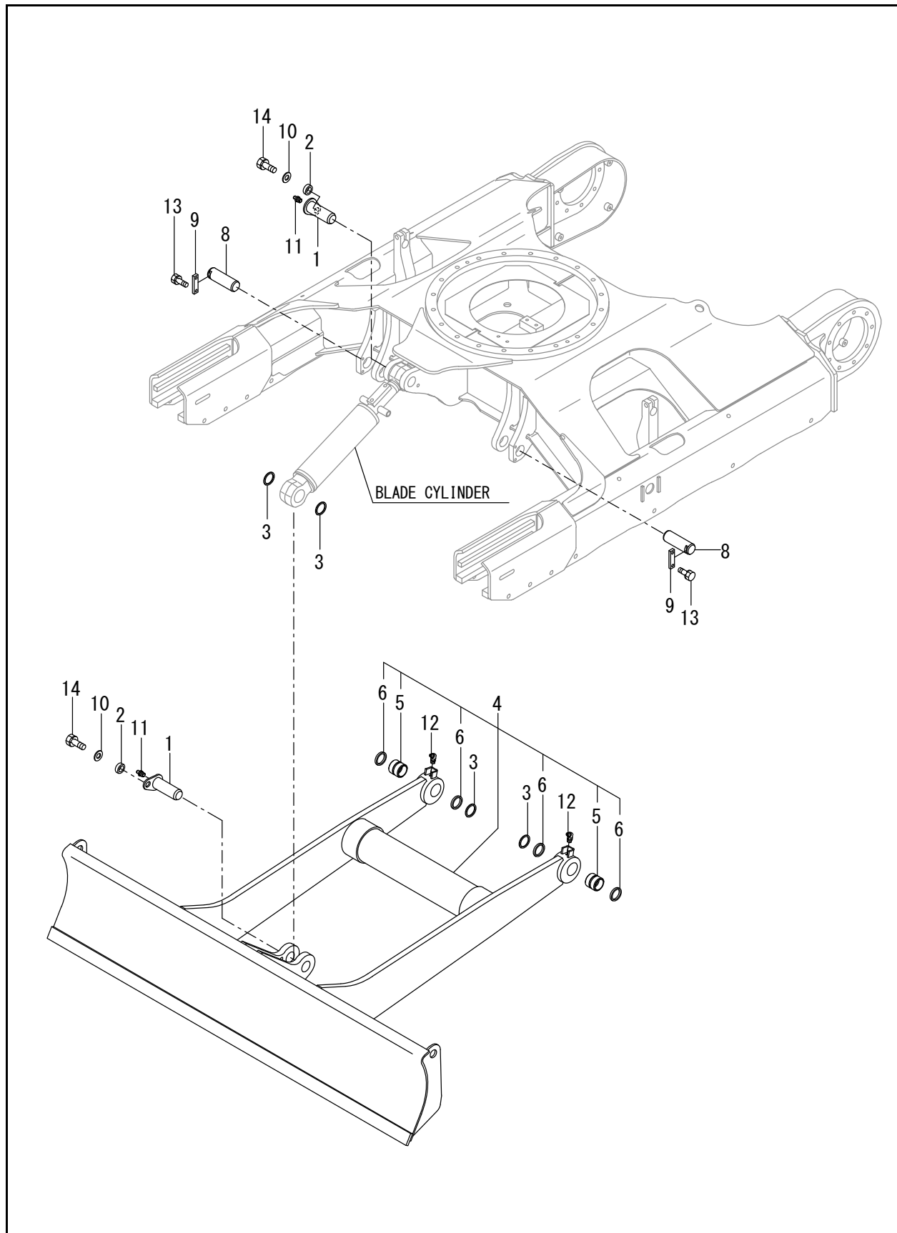
FIG. 128 - BLADE
