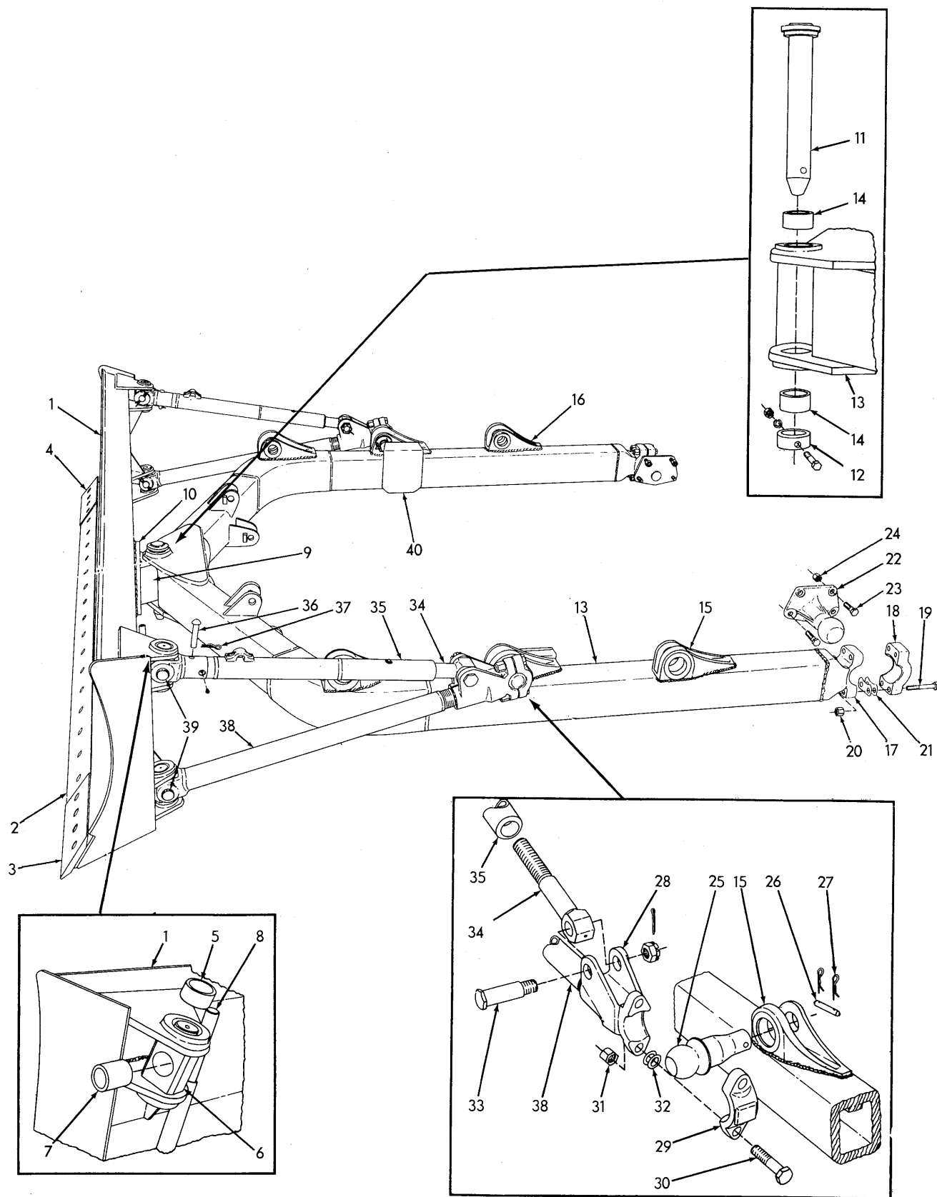
— ANGLING MOLDBOARD —
