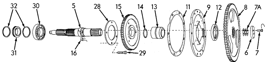
INPUT SHAFT
