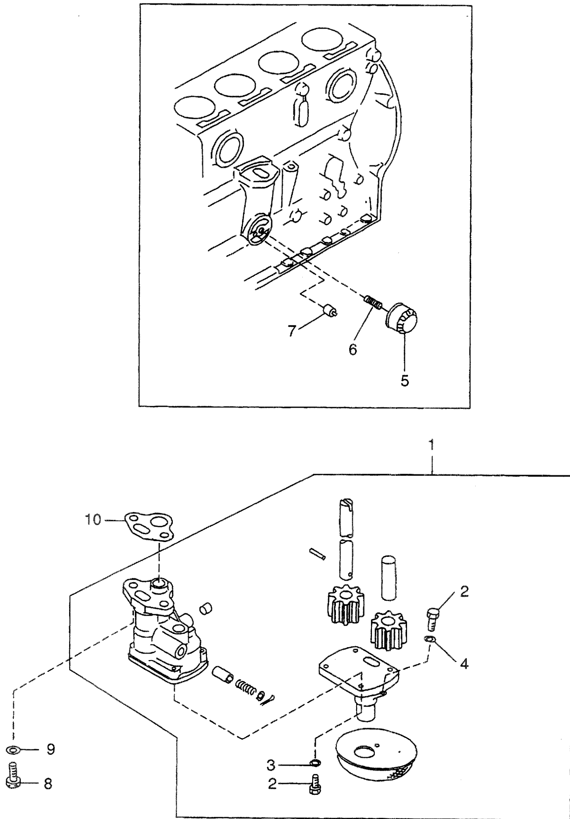
FIG. 23 OIL PUMP & OIL FILTER オイルポンプ およびオイルフィルタ
