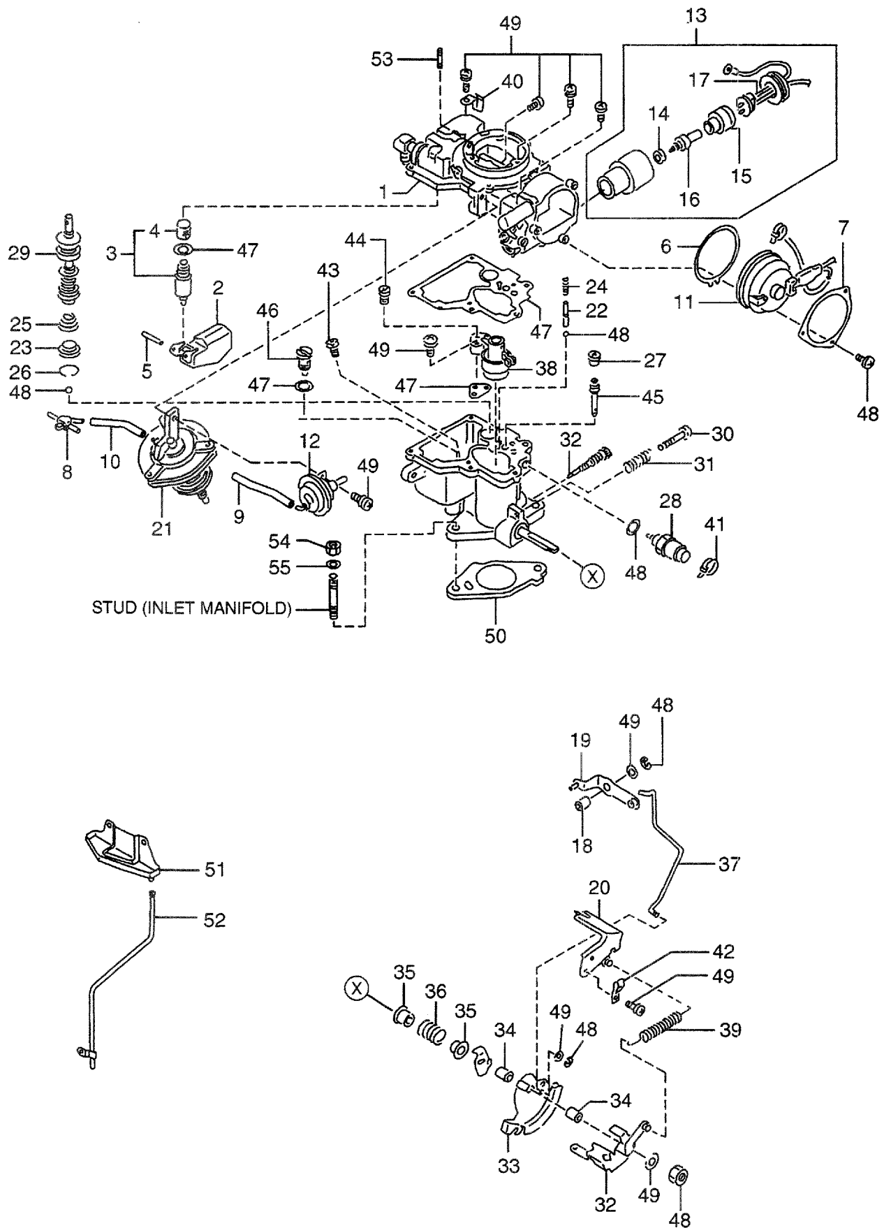
FIG. 30 CARBURETOR キャブレタ
