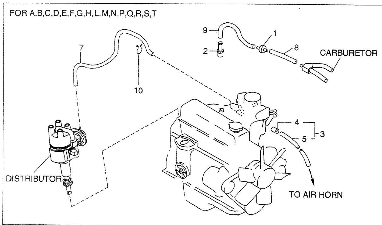
FIG. 49 VACUUM CONTROL SYSTEM バキュームコントロールシステム
