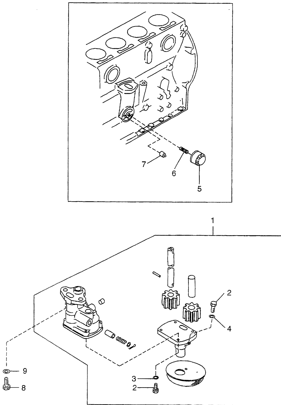
FIG. 22 OIL PUMP & OIL FILTER オイルポンプ およびオイルフィルタ
