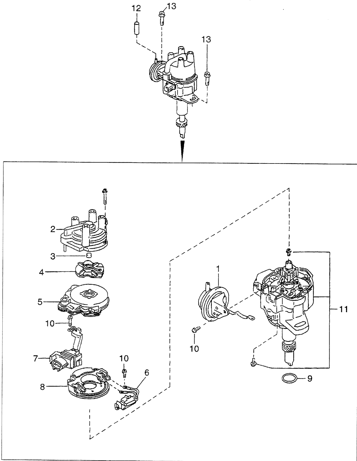
FIG. 48 DISTRIBUTOR ディストリビュータ
