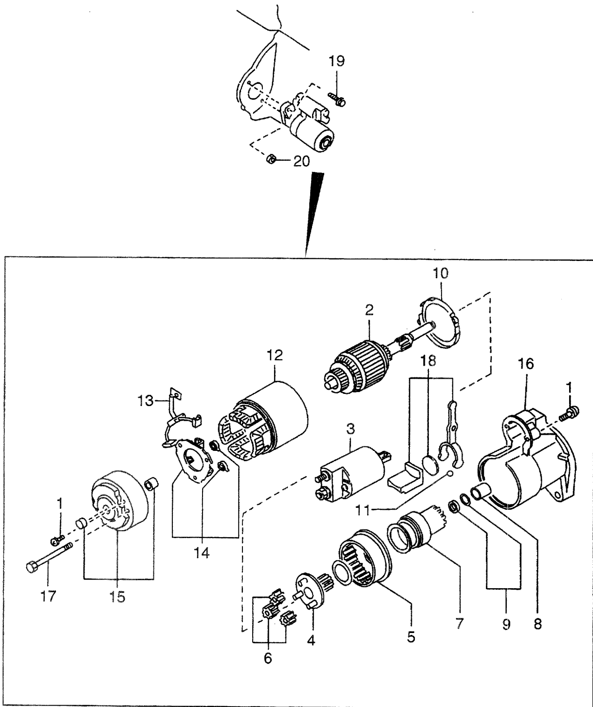
FIG. 65 STARTER スターター
