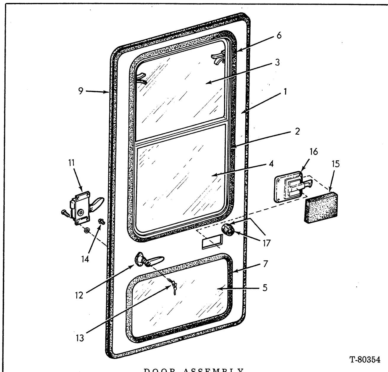
DOOR ASSEMBLY
