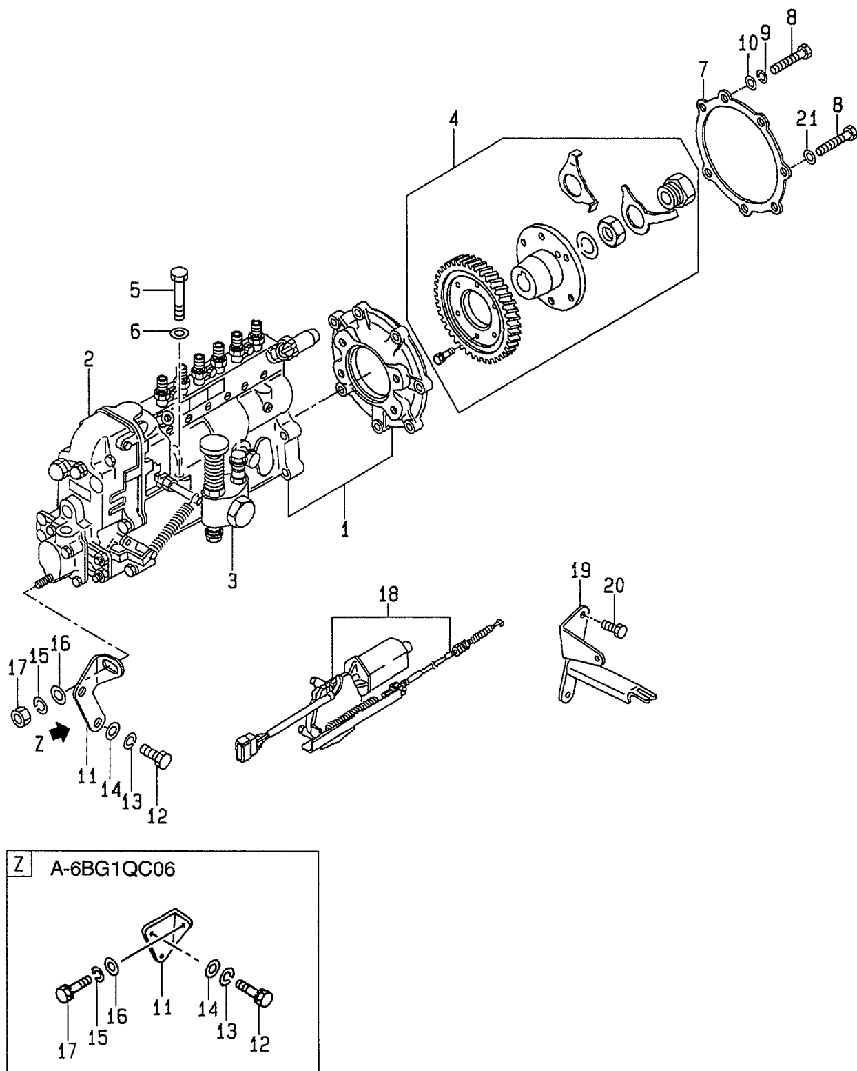
FIG. 30 INJECTION PUMP MOUNT (E,F,G,H,K) インジェクションポンプマウント
