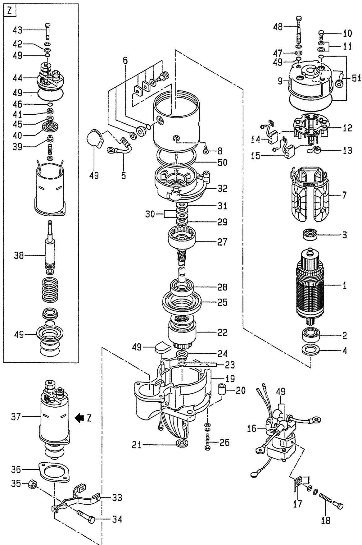
FIG. 36 STARTER (INNER PARTS) (NIKKO MAKE) (A,B) スタータ(インナパーツ)
