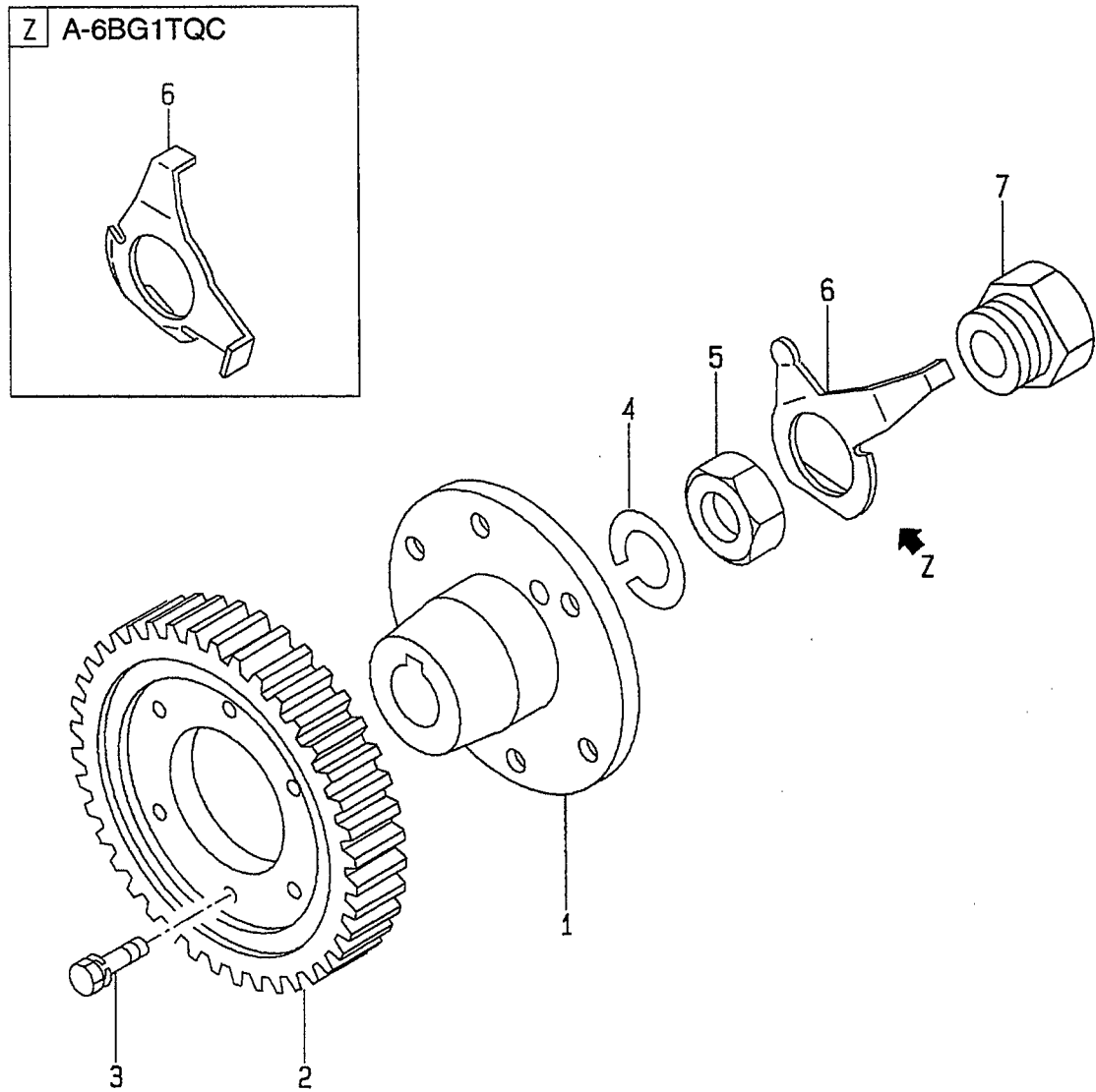
FIG. 34 COUPLING カップリング
