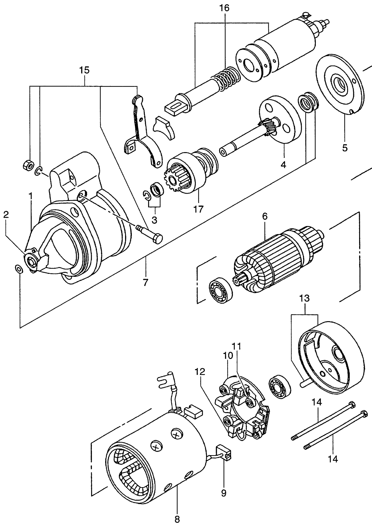
FIG. 37 STARTER (INNER PARTS) (HITACHI MAKE) (A,B) スタータ(インナパーツ)
