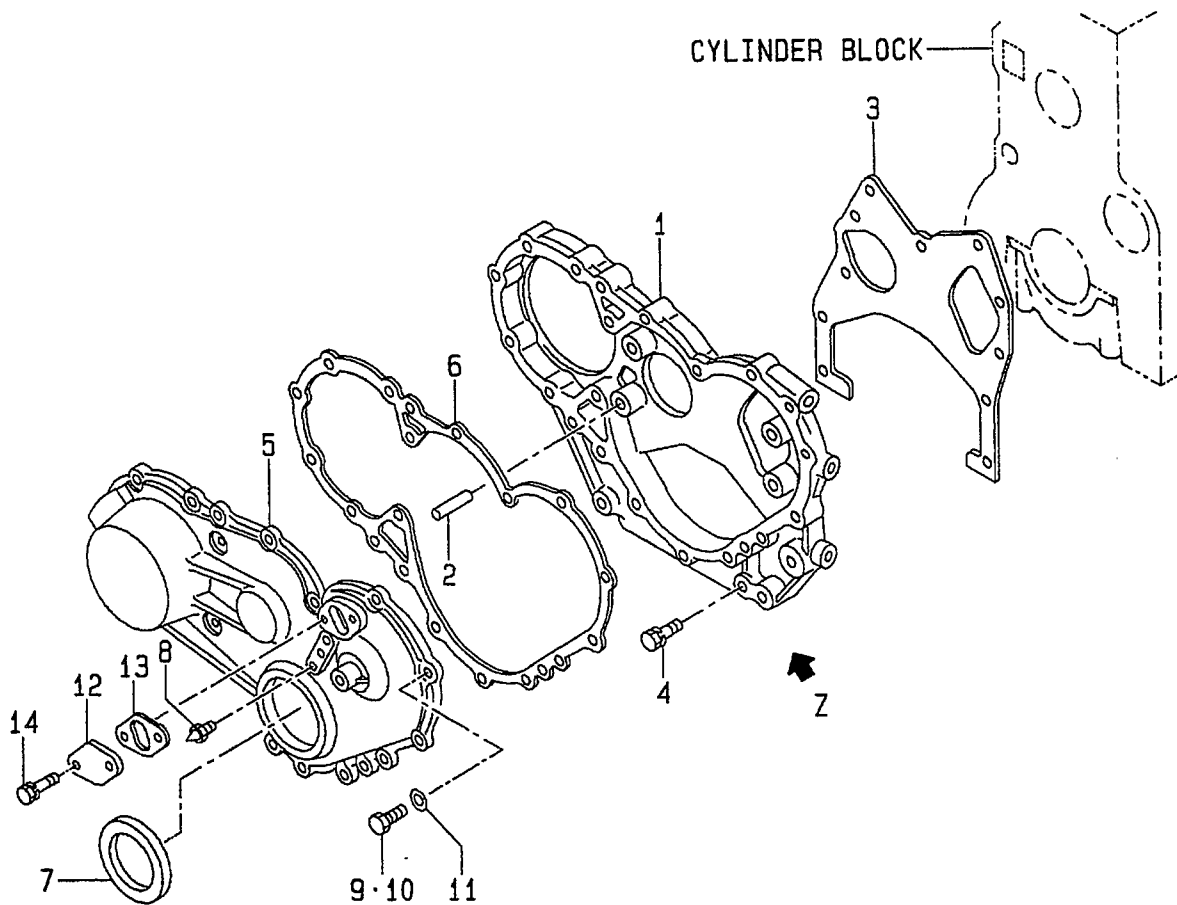
FIG. 4 GEAR CASE ギヤ-ケース
