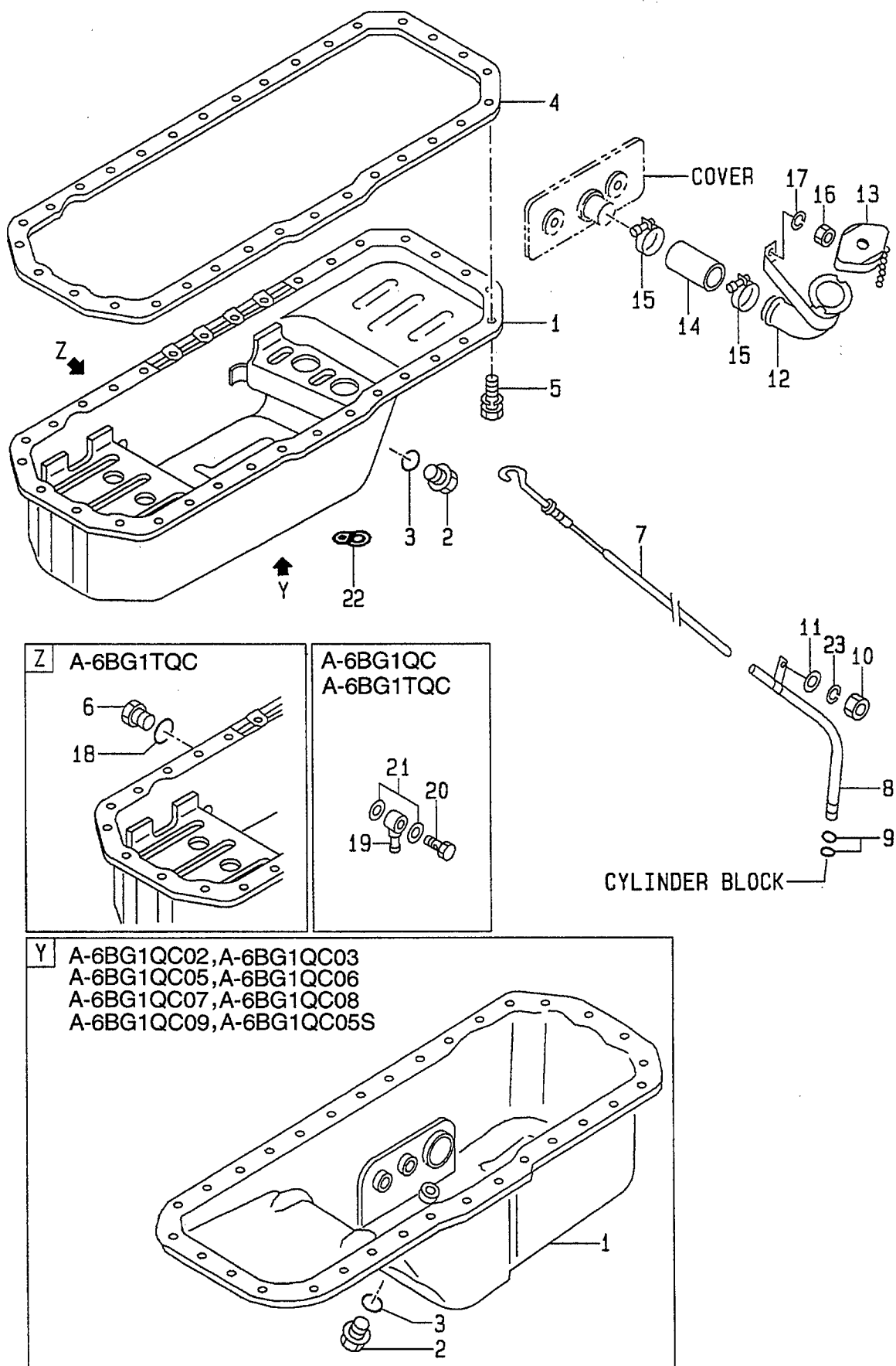
FIG. 6 OIL PAN オイルパン
