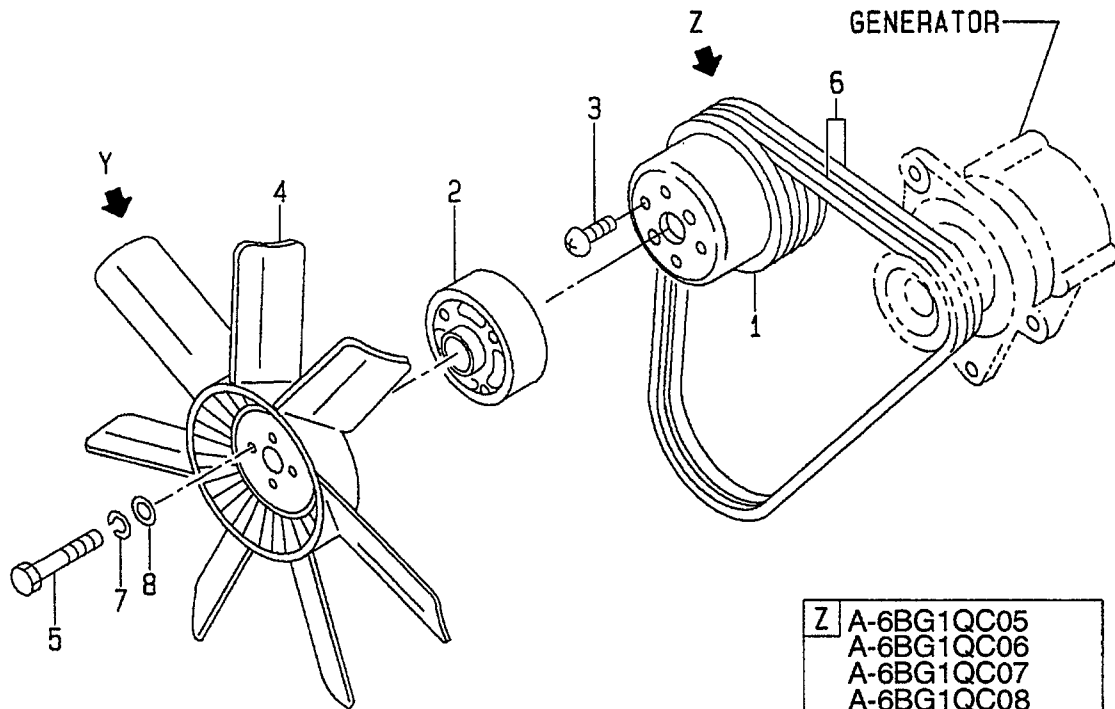
FIG. 20 FAN ファン
