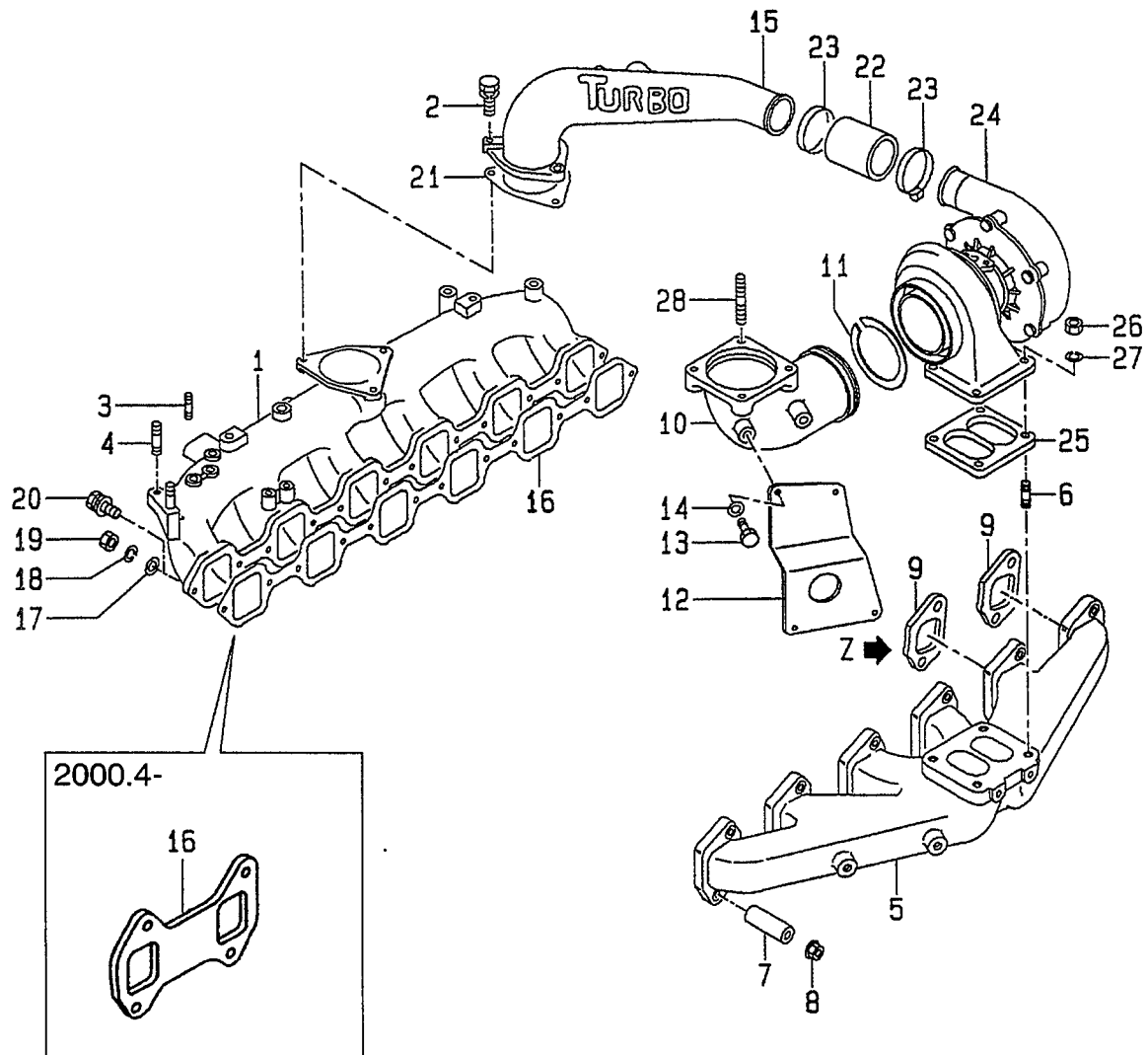
FIG. 10 AIR INTAKE & EXHAUST SYSTEM (B) エア・インターク&エキゾーストシステム
