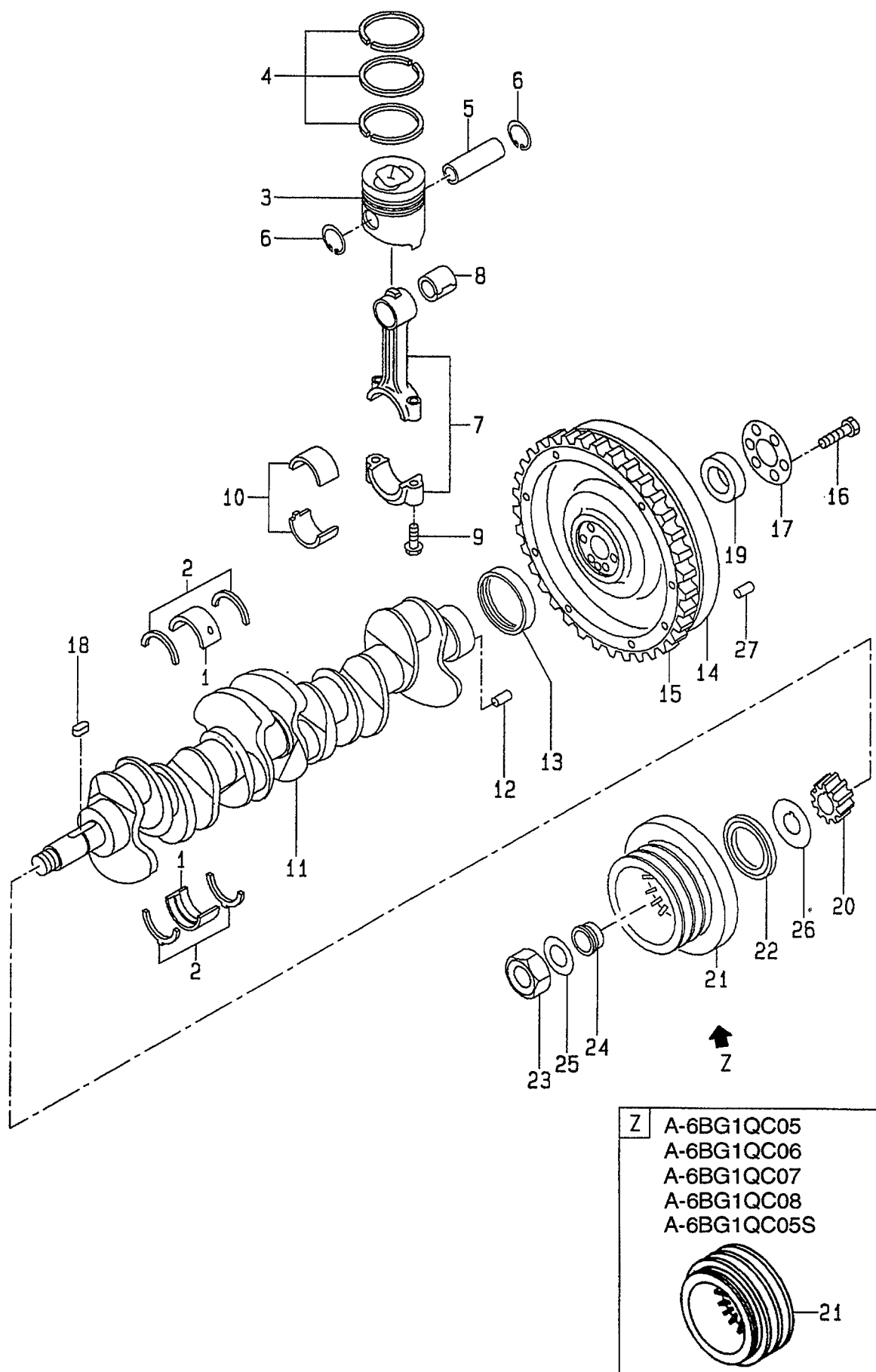
FIG. 3 CRANKSHAFT,PISTON & FLYWHEEL クランクシャフト,ピストン&フライホイール
