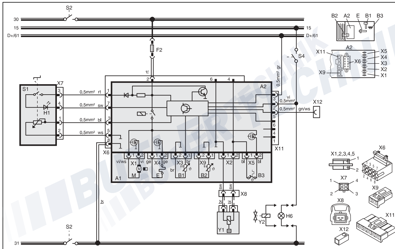
Bild 33: Automatischschaltplan Air Top 2000, 24V ADR-Betrieb mit Bedienelement, Legende siehe Seite 32 und 33
