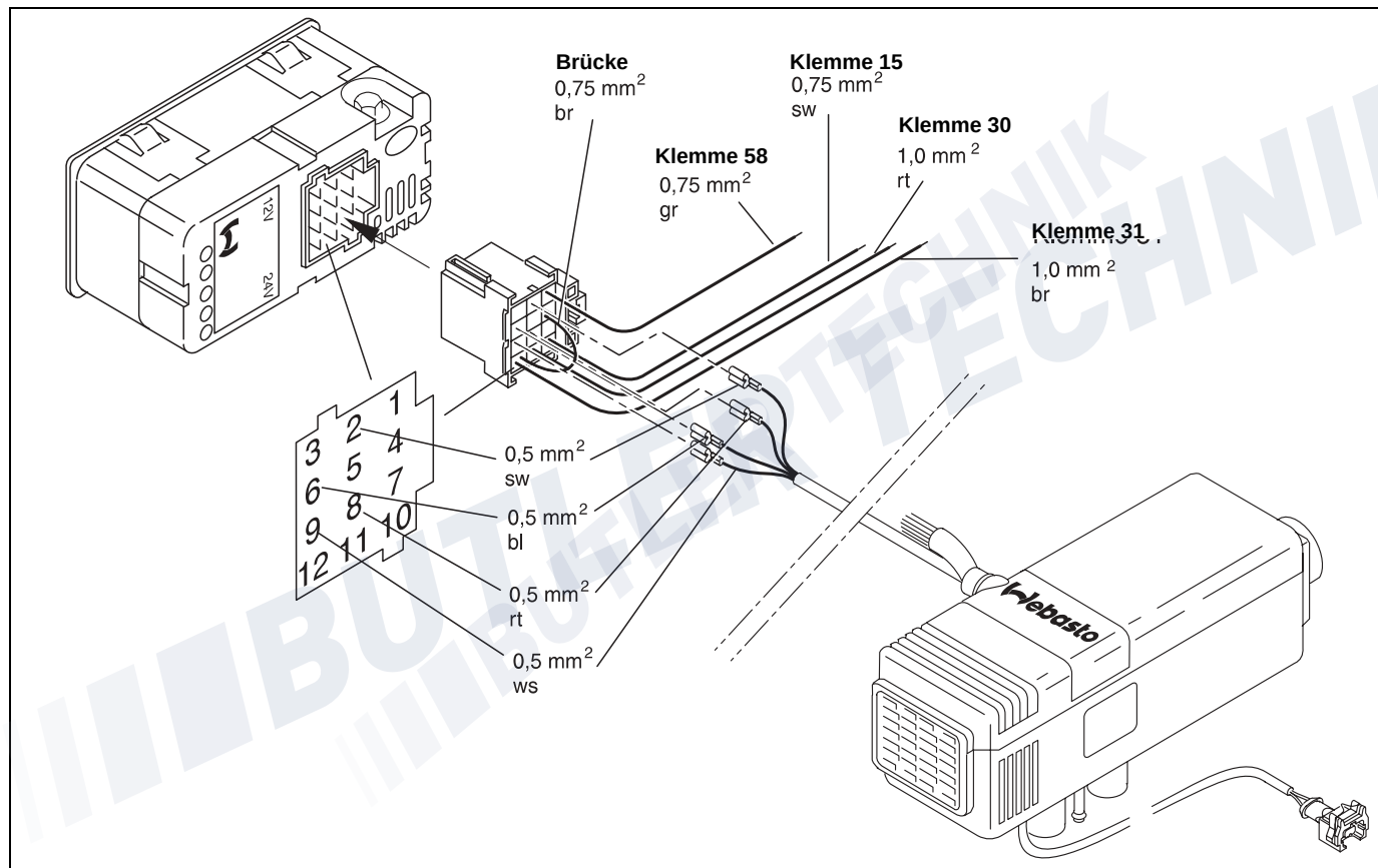
Bild 29: Anschlussschema Air Top 2000, Lieferumfang Komfort
