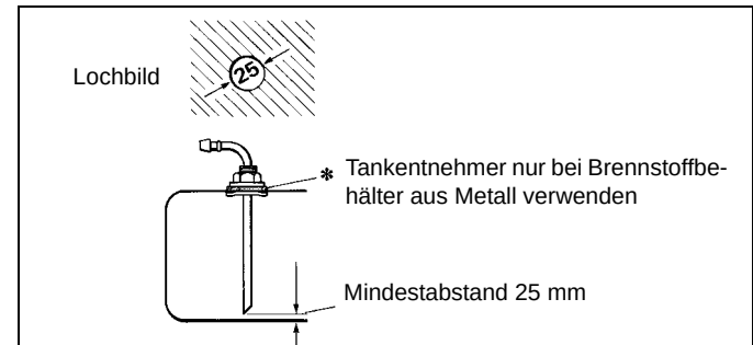
Bild 11: Webasto-Tankentnehmer
