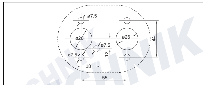
Fig. 3 Gabarit du trou
