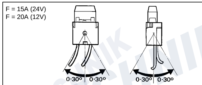
Bild 25: Sicherungshalter, Einbaulage
