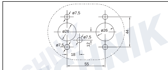
Bild 3: Lochbild
