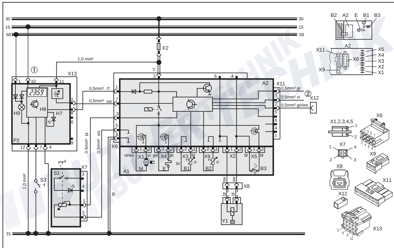
Bild 32: Automatischschaltplan Air Top 2000, 12V/24V mit Bedienelement und Kombiuhr, Legende siehe Seite 32 und 33
