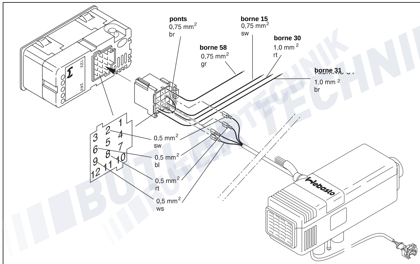
Fig. 29 Schéma de raccordement Air Top 2000, version confort
