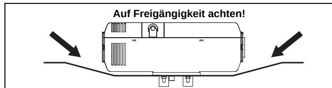
Bild 5: Einbau
