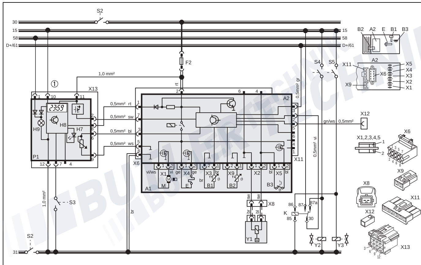
Bild 35: Automatikschaltplan Air Top 2000, 24V ADR-Betrieb mit Kombiuhr und 2 Nebenantrieben, Legende siehe Seite 32 und 33
