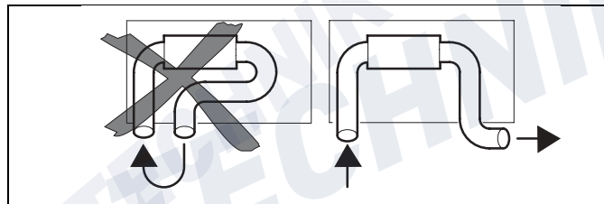
Bild 8: Heizlufteintritt und Heizluftaustritt
