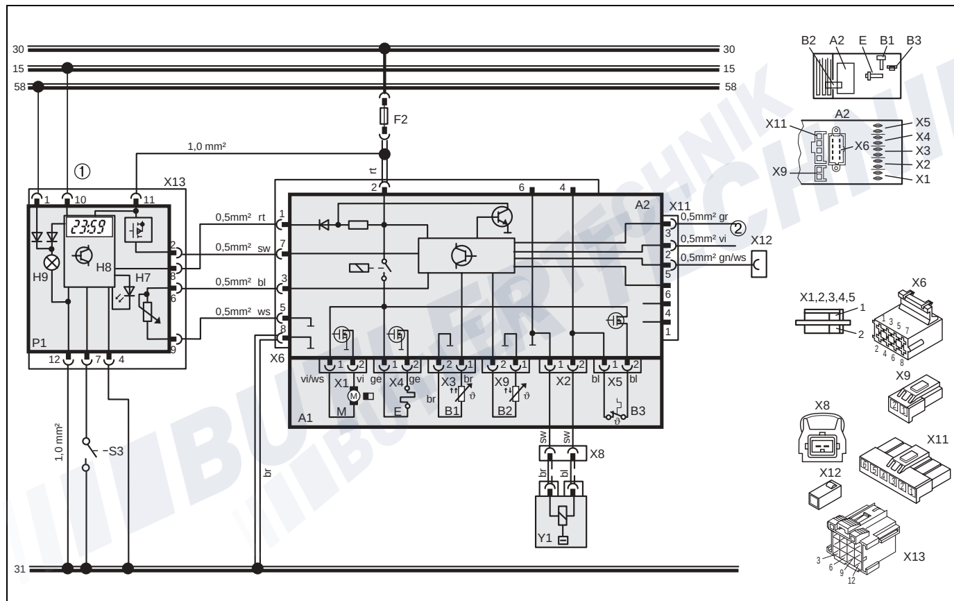
Bild 31: Automatikschaltplan Air Top 2000, 12V/24V mit Kombiuhr, Legende siehe Seite 32 und 33
