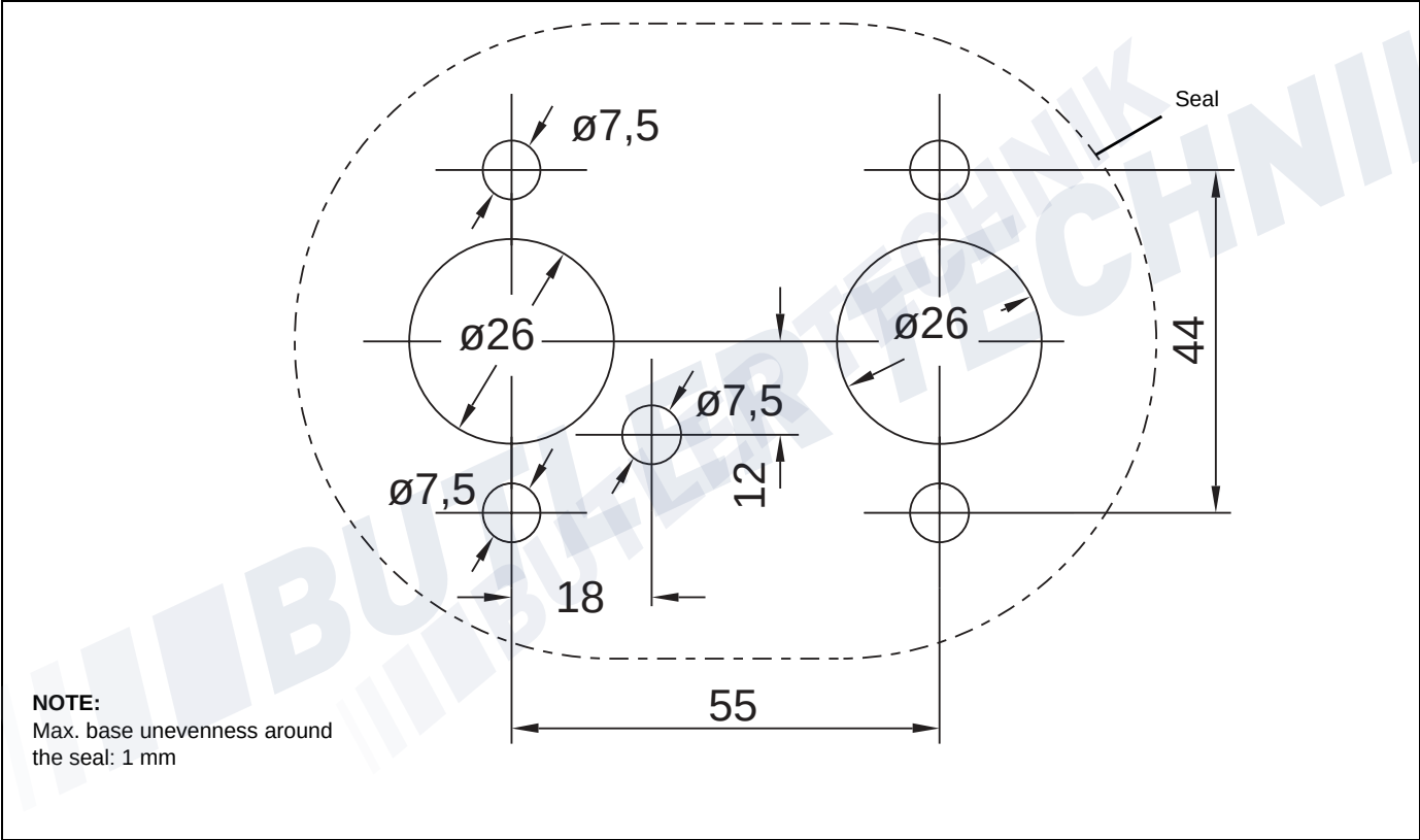
Fig. 37: Drilling template
