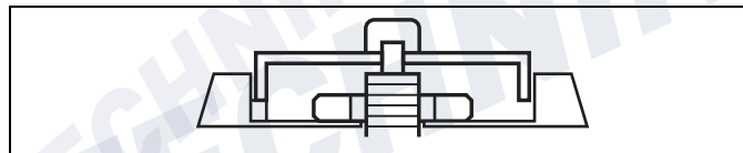
Fig. 28 Montage de l'organe de commande (incorrect)
