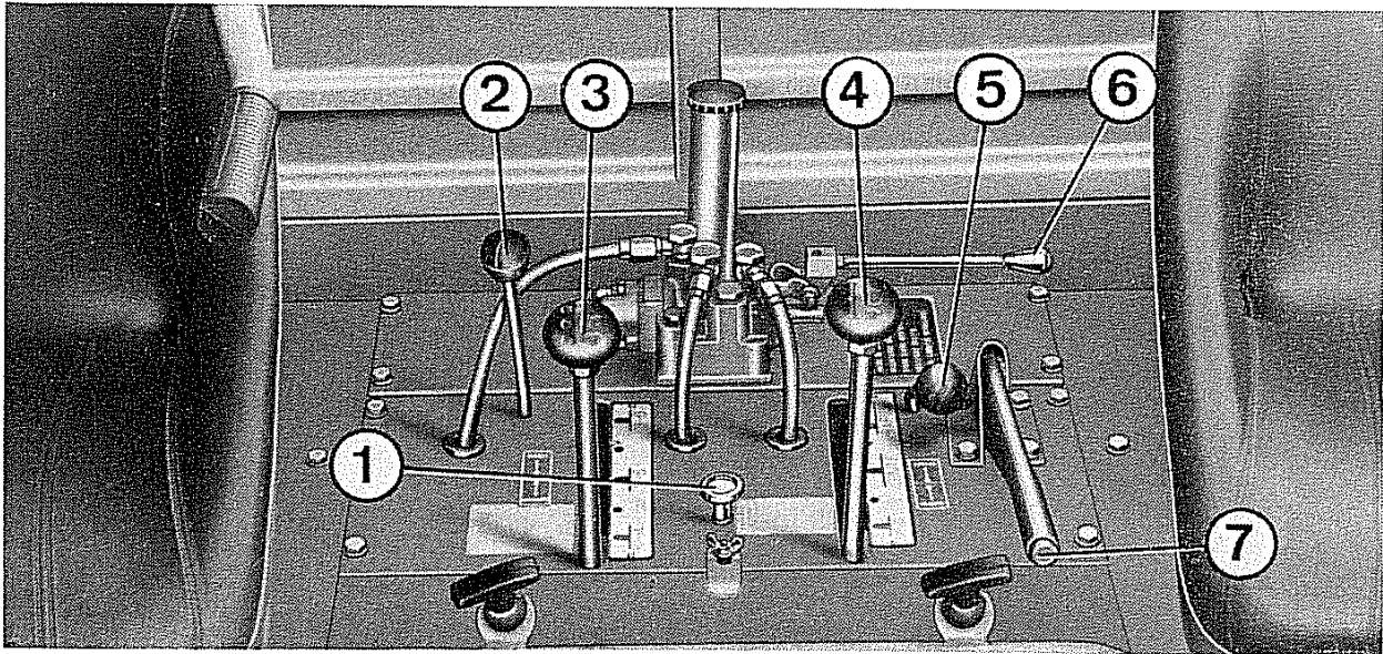
Fig. 1 - Comandi
