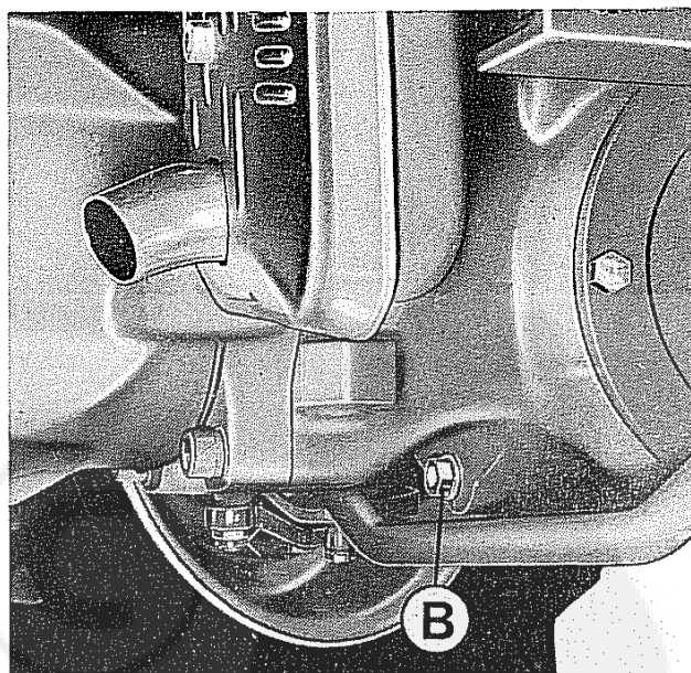
Fig. 18 - Scarico olio nel carter cambio
