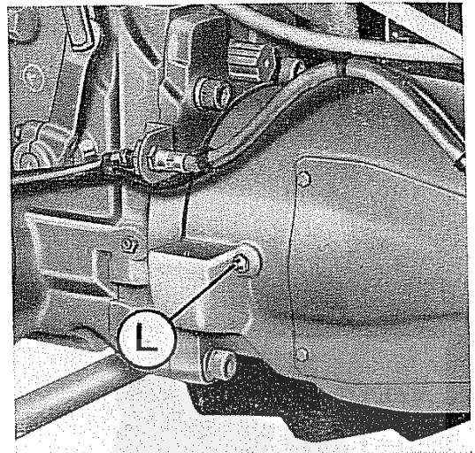
Fig. 15 - Punti d'ingrassaggio
