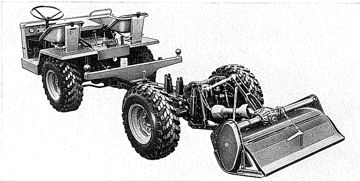
Fig. 39 - Applicazione fresa
