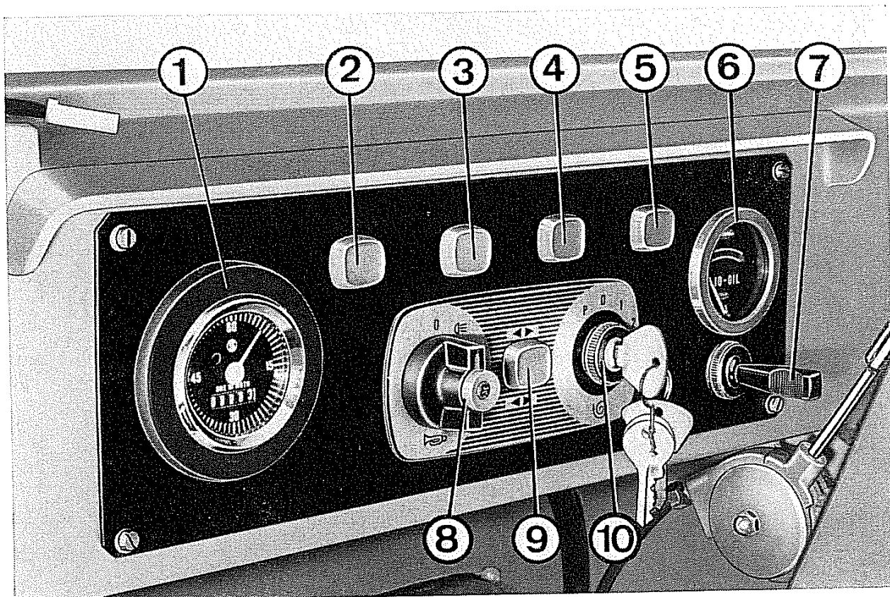
Fig. 31 - Cruscotto
