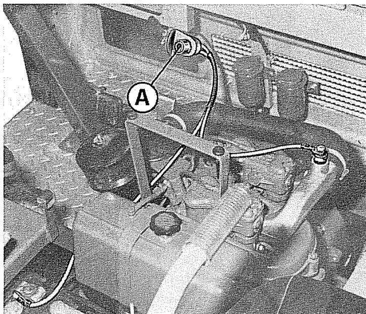
Fig. 33 - Termoavviatore
