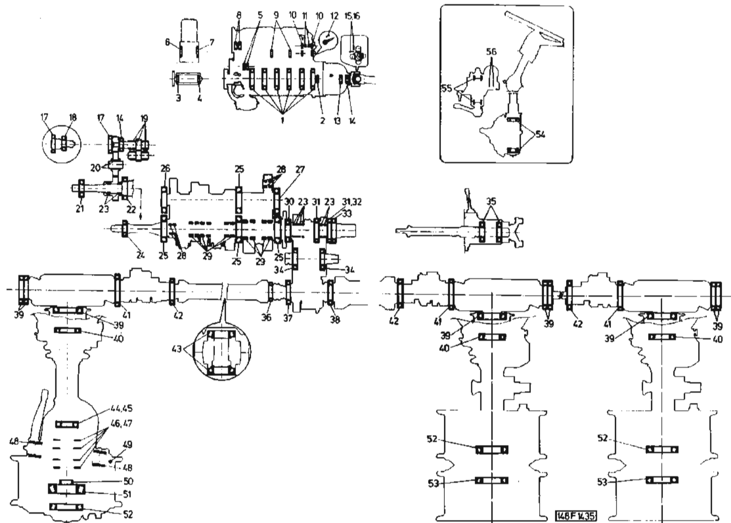
Seznam valivých ložisek motoru a podvozku – Verzeichnis der Wälzlager des Motors und Fahrgestells – TAB. 3 List of antifriction bearings of engine and chassis – Liste des roulements du moteur et du châssis
