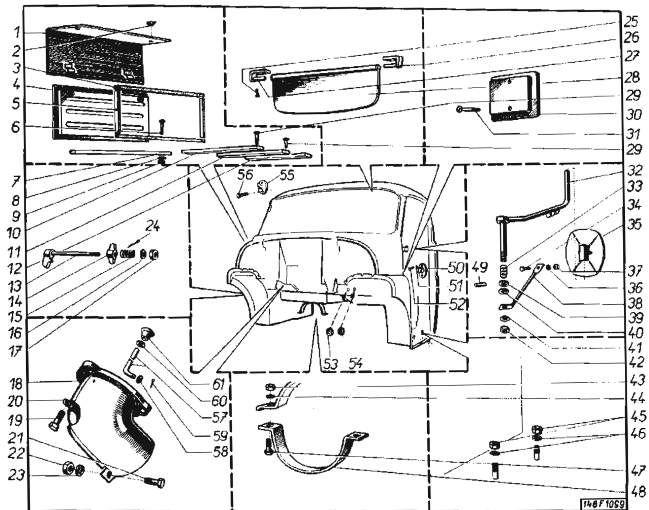
Součásti budky řidiče — Bestandteile des Fahrerhauses — Driver's cab elements — Pièces de la cabine du conducteur TAB. 119
