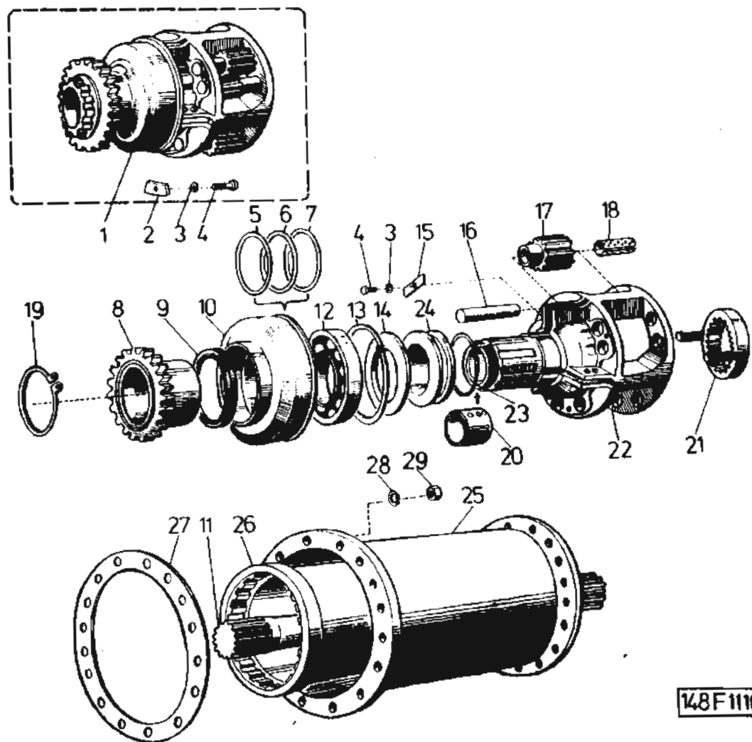
Vyrovnávací soukolí (diferenciál) střední nápravy — Ausgleichgetriebe (Differential) der mittleren Achse — TAB. 87 Middle-axle differential gearing — Différentiel du premier pont arrière
