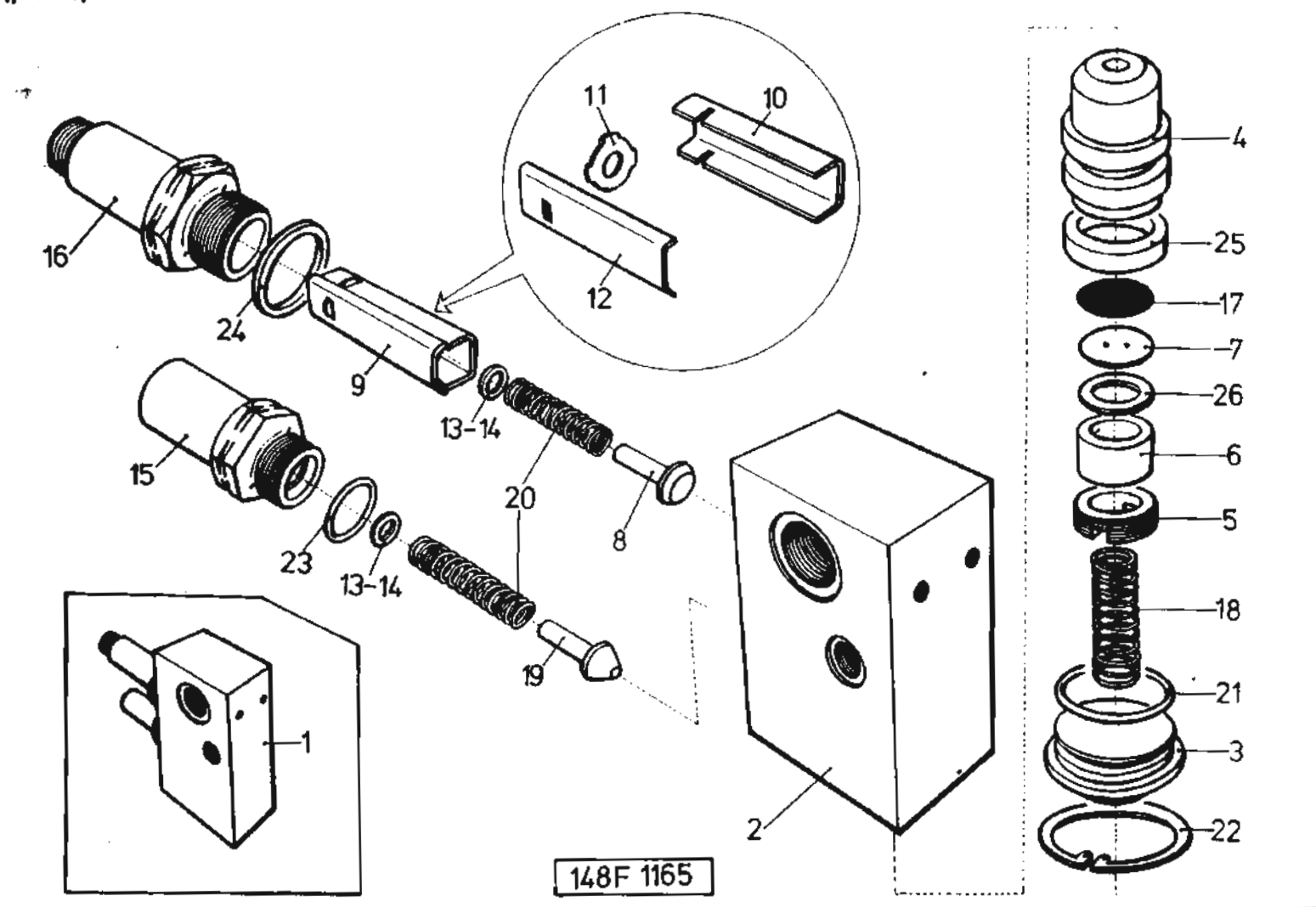
Přepouštěcí ventil (součásti) – Überlaufventil (Bestandteile) – Over-flow valve (parts) – Distributeur (pièces)
