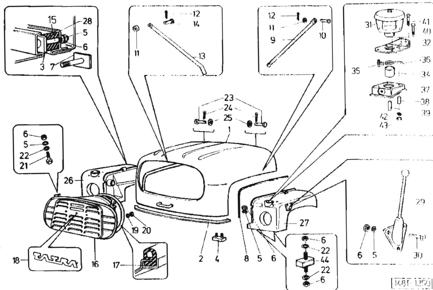
Kapota s maskou, přední blatníky – Motorhaube mit Maske, vordere Kotflügel – Bonnet c/w grill, front mudguards – Capot moteur avec calandre, ailes avant TAB. 117
