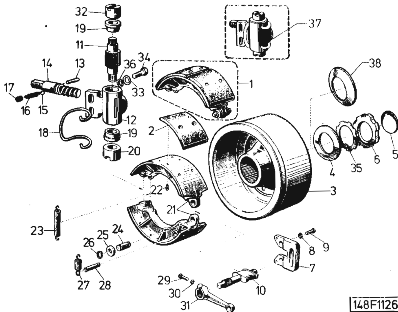
Brzdový buben a čelisti ruční brzdy – Bremstrommel und Bremsbacken der Handbremse – Brake drum and handbrake shoes – Tambour de frein et segments de frein à main TAB. 49
