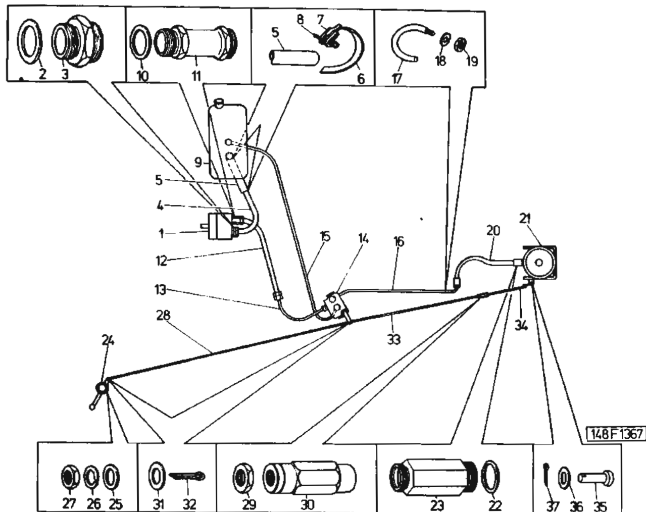
Součásti ovládání sklápěcího zařízení (S1) – Bestandteile für die Betätigung der Kippeinrichtung (S1) – TAB. 105 Parts of tilting mechanism control (S1) – Pièces de commande de basculement (S1) – (od 75 501. V.)
