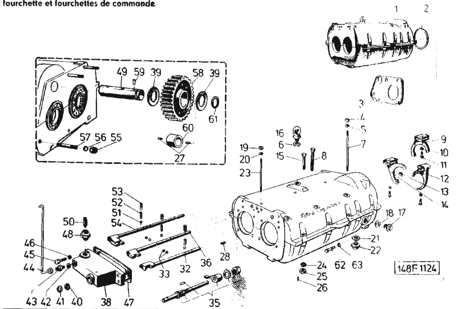
Skříň převodovky, vložené kolo zpětného chodu, zasouvací tyče a vidlice – Wechselgetriebe-Gehäuse, Rückwärtsgang-Zwischenrad, Schaltstangen und Schaltgabeln – Gearbox housing, intermediate reverse gear, gearshift rods and forks – Carter de la boîte de vitesses, pignon intercalé de marche AR, axes de fourchette et fourchettes de commande TAB. 41
