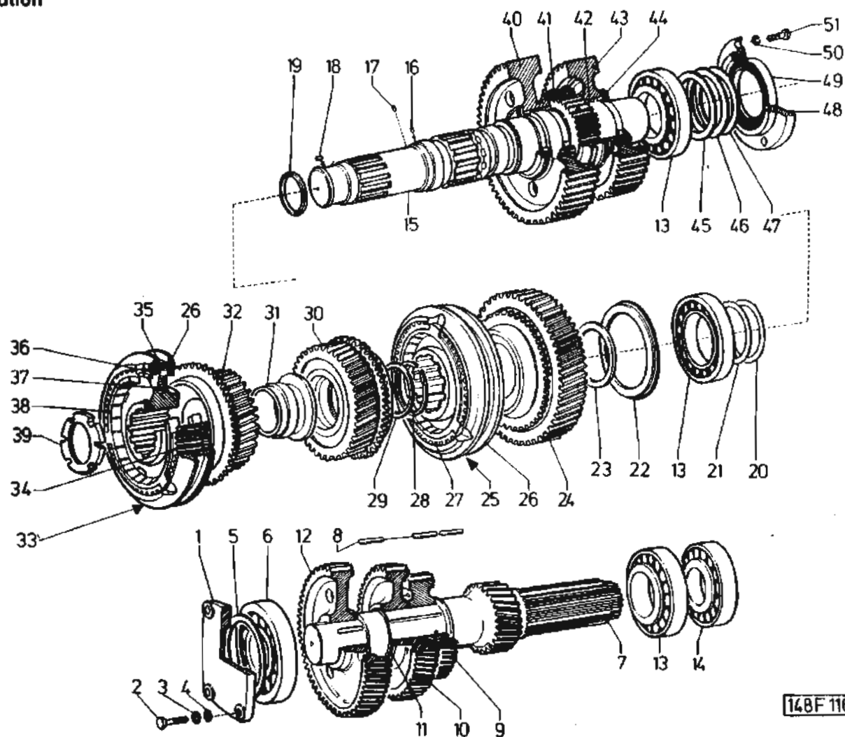
Hnaný hřídel s převodovými koly a synchrony – Getriebene Welle mit Zahnradern und Gleichlauf- TAB. 43 tung – Driven shaft with gears and synchromesh mechanisms – Arbre mené avec roues de transmission et synchronisation
