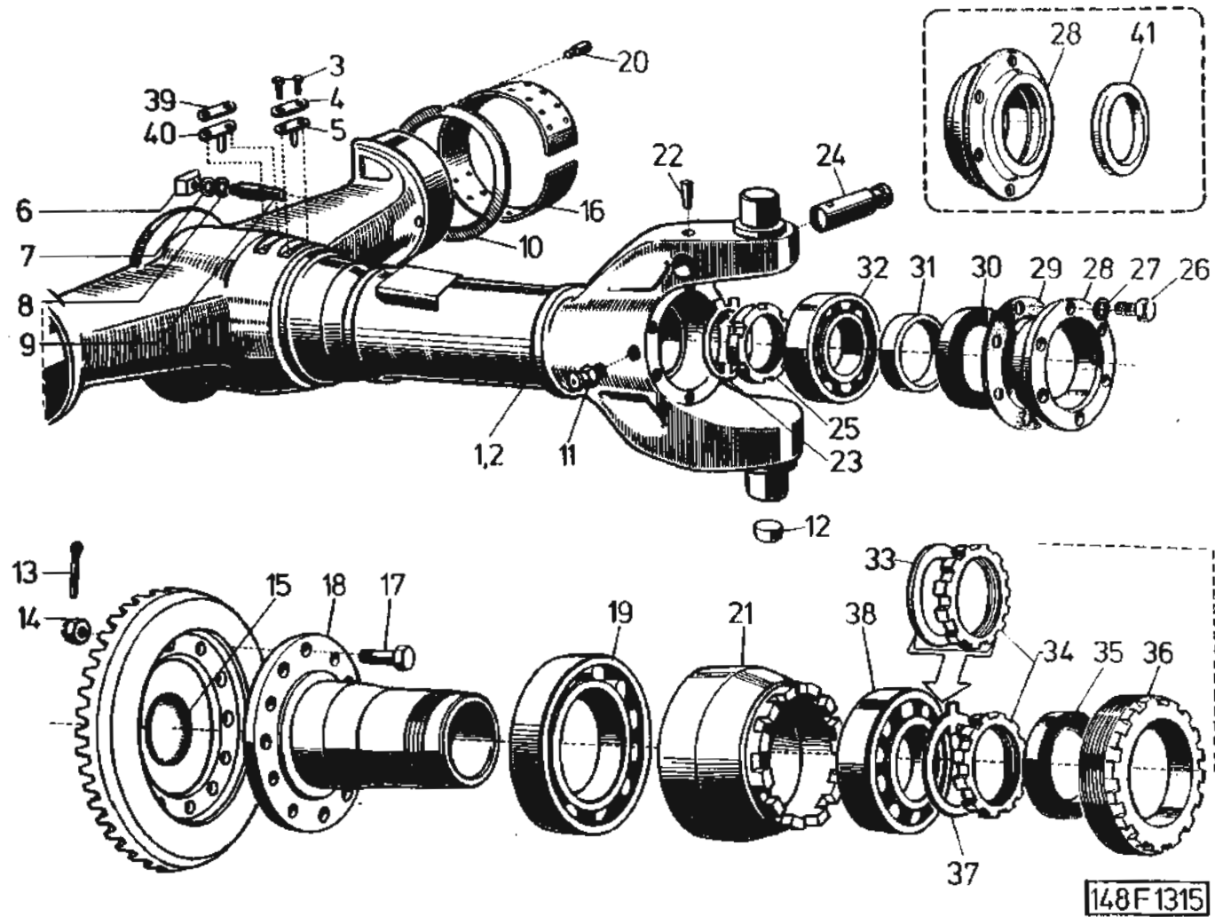
Přední kyvadlové polonápravy — Vordere Schwinghalbachsen — Front swing half-axes — Demi-arbres oscillants avant
