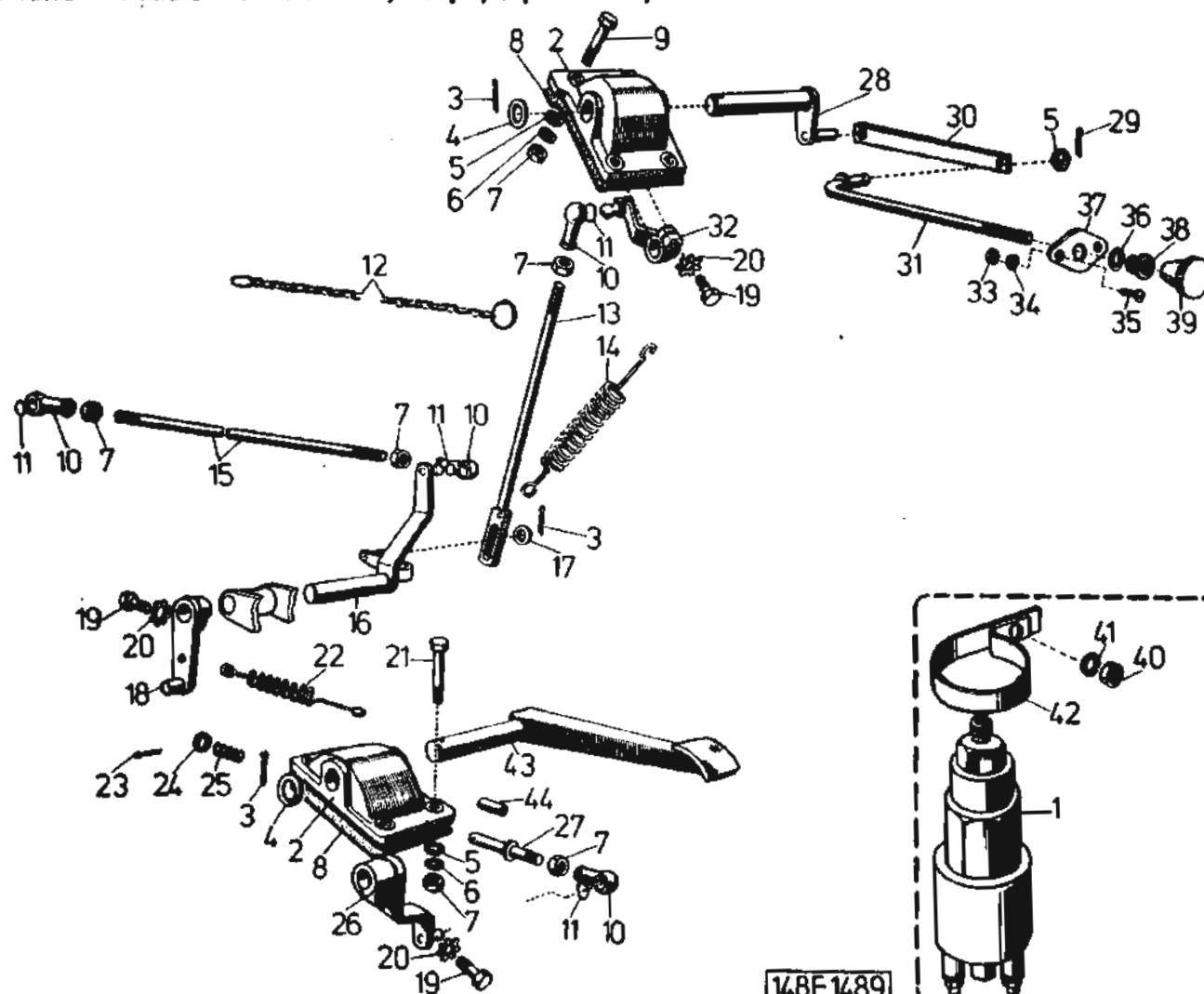
Pedál akcelátoru, pneumatický ventil – Fahr­fusshebel, pneumatisches Ventil – Accelerator pedal, pneumatic valve – Pédale d'accélérateur, soupape pneumatique
