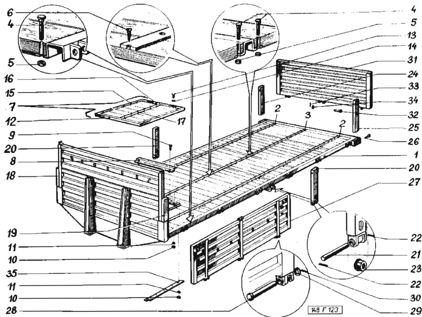
Plošina volniku (čela a bočnice) — Pritschenplattform (Stirn- und Seitenwände) — Platform lorry body TAB. 139 (face and side walls) — Plate-forme du camion (faces frontales et paroi latérale)
