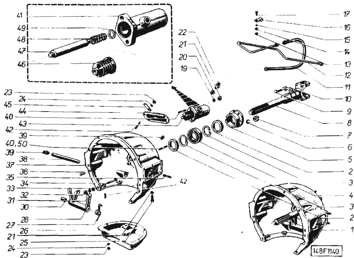
Skříň spojky, spojkový hřídel — Kupplungsgehäuse, Kupplungswelle — Clutch housing, clutch shaft — Boîtier d'embrayage, arbre d'embrayage
