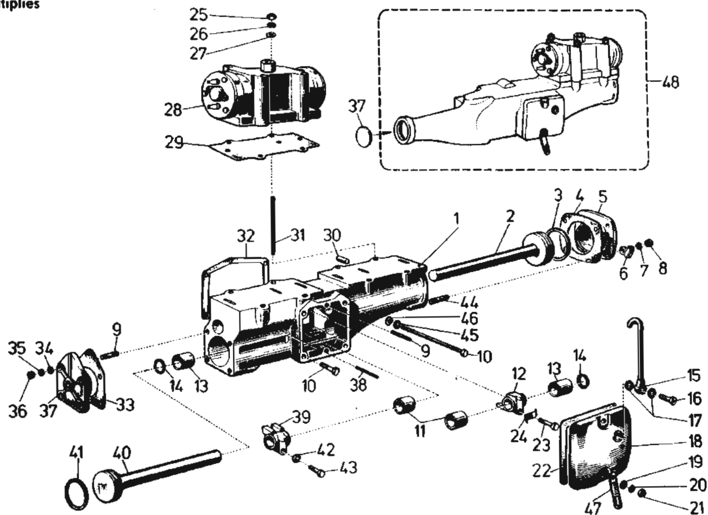
Skříň tlakovzdušného řazení redukčního převodu – Druckluft-Schaltgehäuse des Zusatzgetriebes – Pneumatic gear-shift housing of auxiliary gearbox – Boîtier de commande pneumatique des rapports démultipliés
