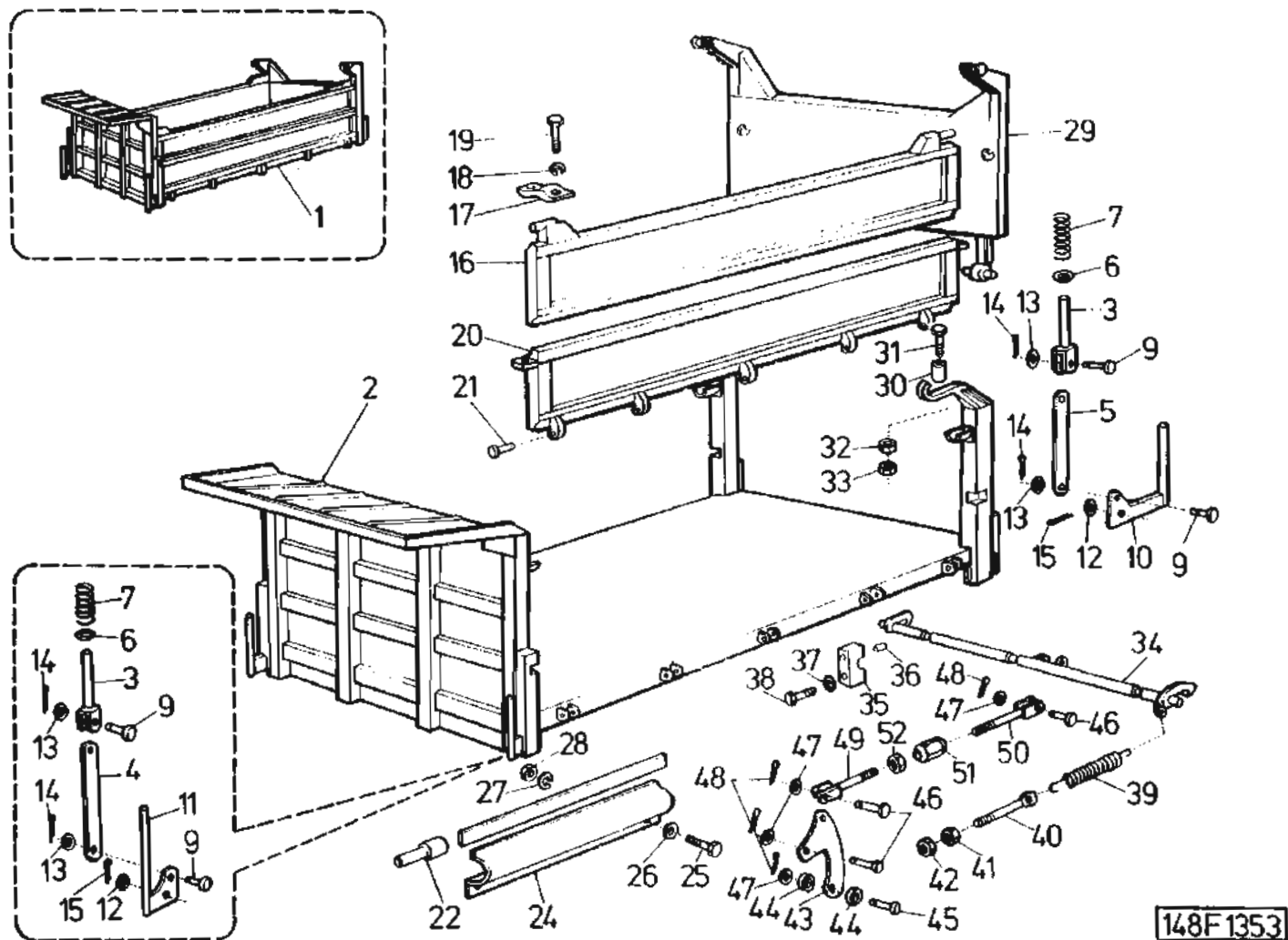
Korba sklápěčky S3 — Kipperaufbau S3 — Body of dumper S3 — Benne basculante S3 — {od 75 501. V.} TAB. 135
