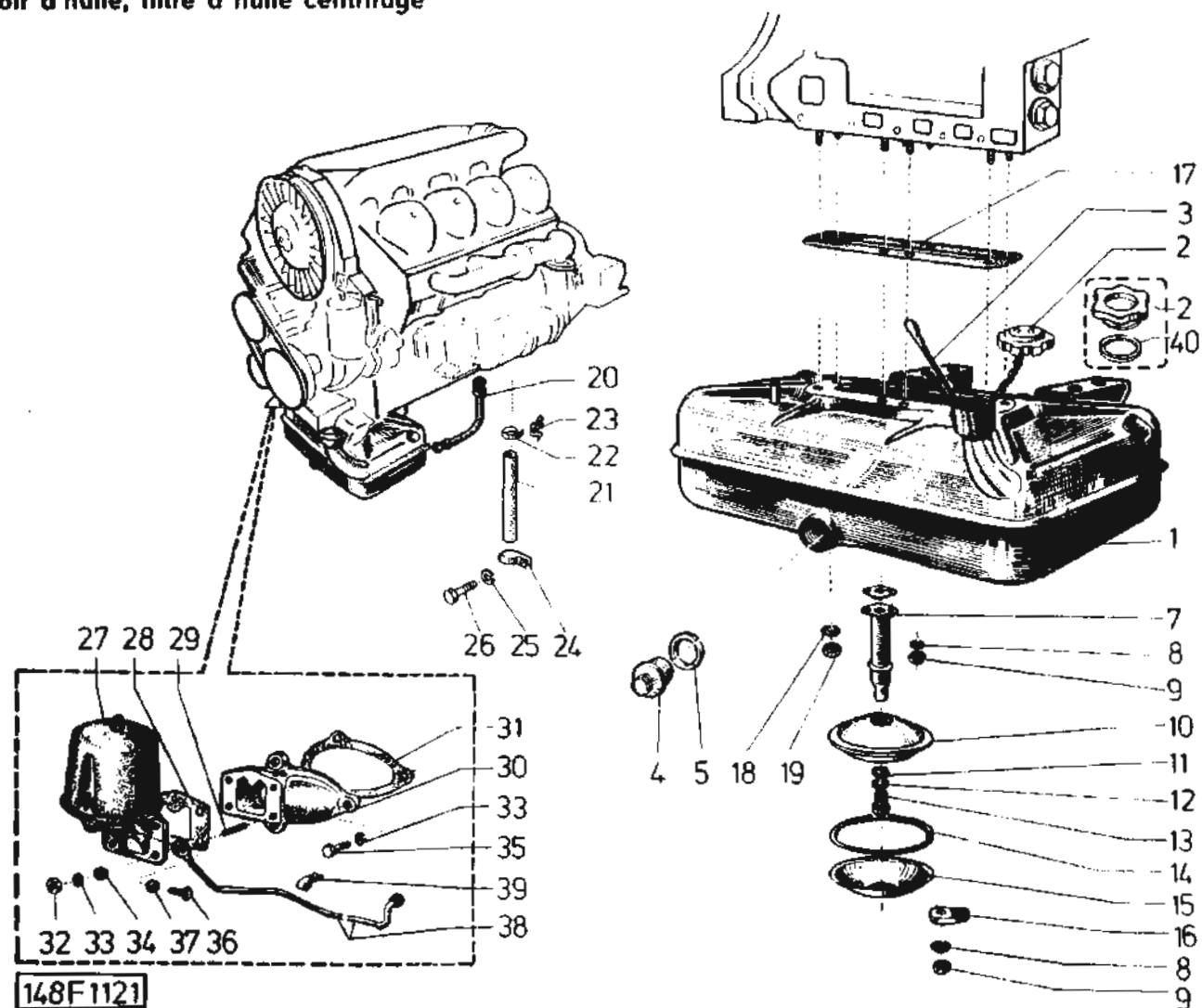
Olejová nádrž, odstředivý čistič oleje – Ölbehälter, Fliehkraft-Ölfilter – Oil tank, centrifugal oil filter – TAB. 25 Réservoir d'huile, filtre à huile centrifuge
