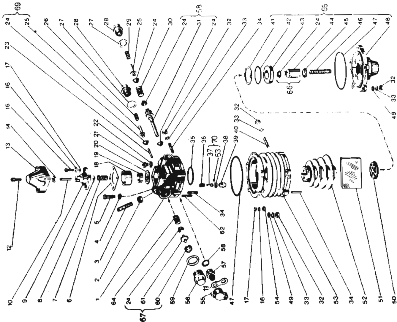
Sdružený regulátor tlaku vzduchu (součásti) – Kombiniertes Luftdruckregler (Bestandteile) – Air-pressure governor (parts) – Régulateur de pression d'air combiné (pièces) TAB. 97
