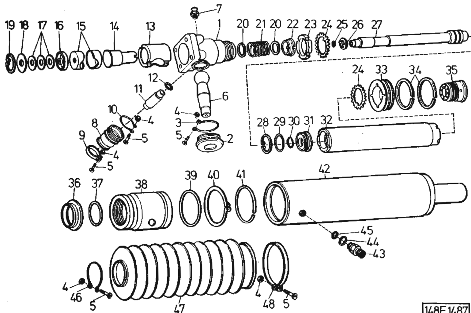
Válec servořízení (součásti) — Servolenkung-Zylinder (Bestandteile) — Servosteering cylinder, (parts) — TAB. 75 Cylindre de servo-direction (pièces)
