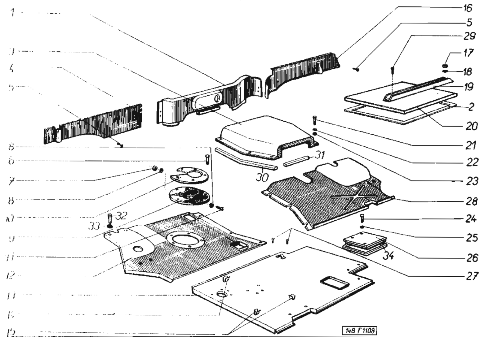
1A8. 120 Odnímatelné díly podlahy budky řidiče – Abnehmbare Fahrerhaus-Fussbodenteile – Dismountable parts of driver's cab floor – Pièces démontables du placher de la cabine
