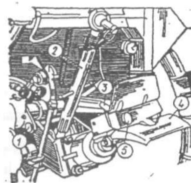
48. ábra Pótkocsi felső vonófej
