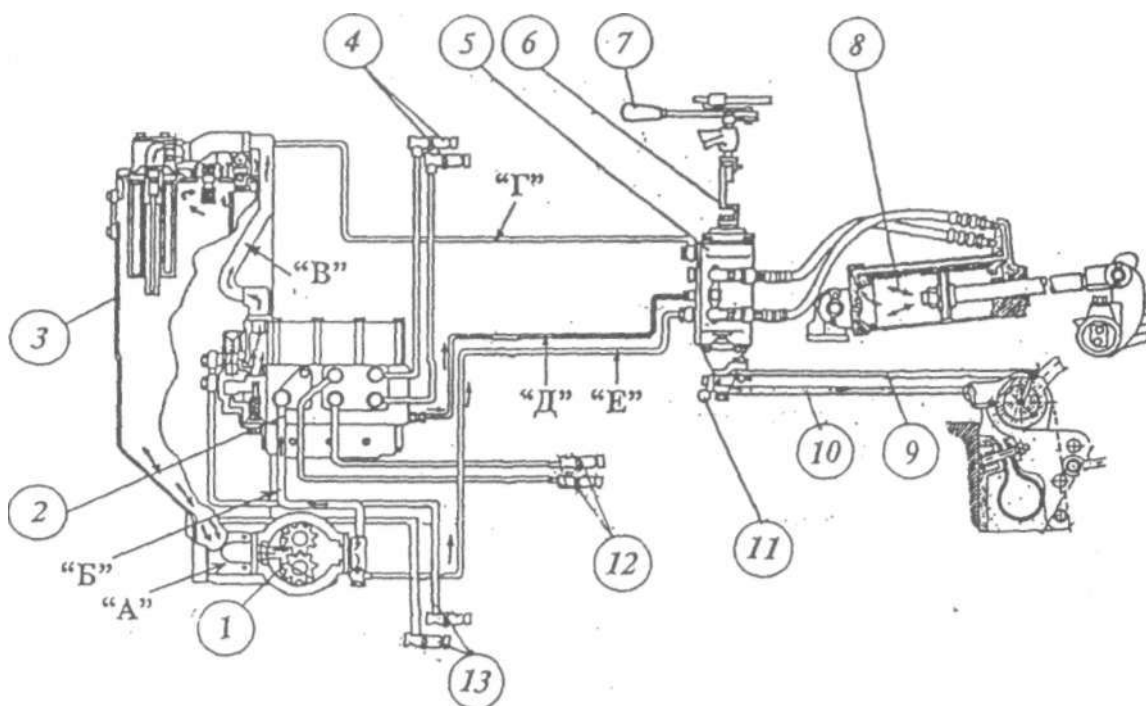
27. ábra A hidraulika rendszer vázlata
