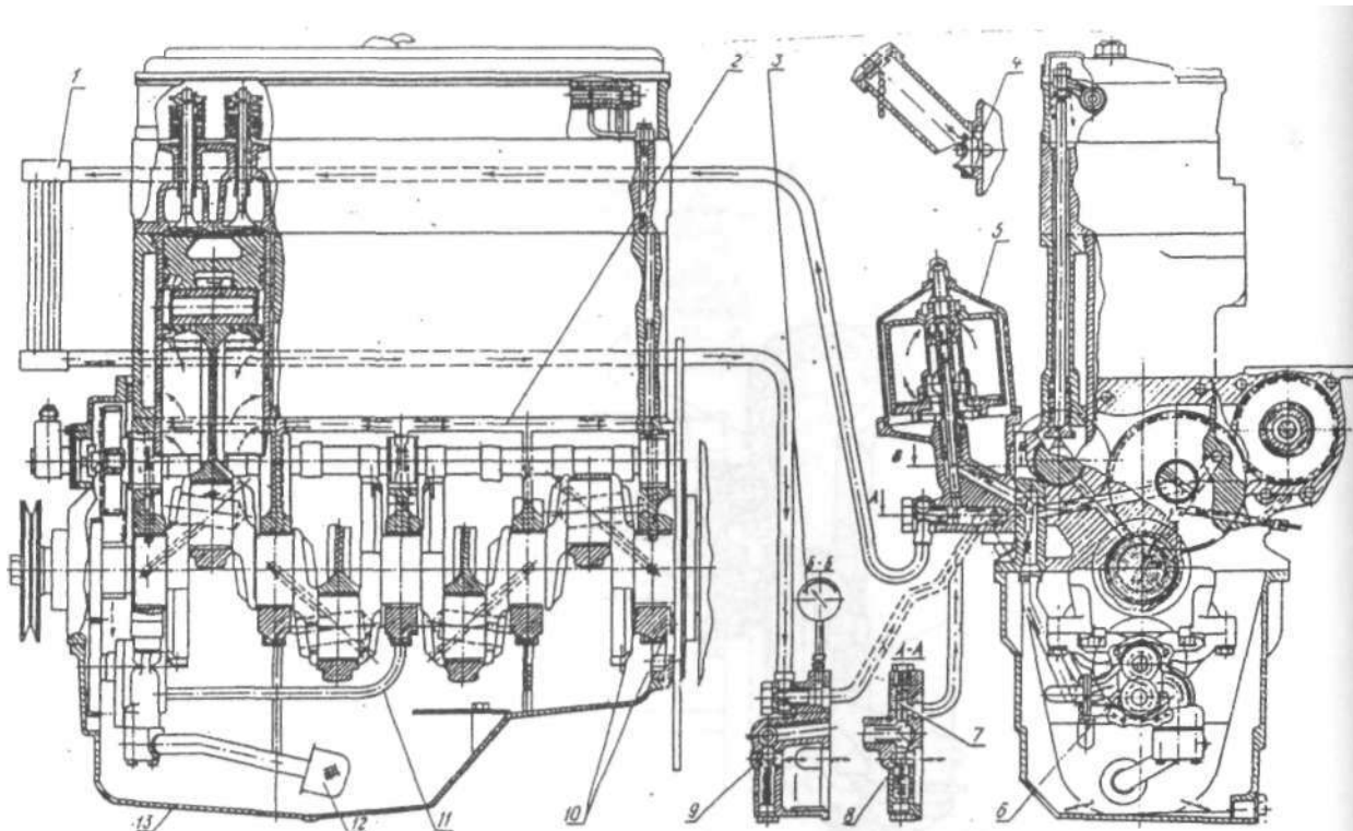
24. ábra A motor kenési rendszere
