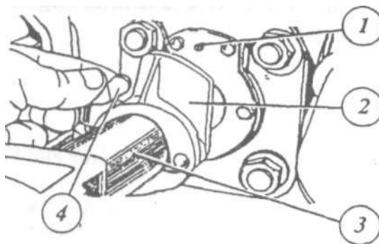
50. ábra A függesztőmű munkahenger lökethatároló
