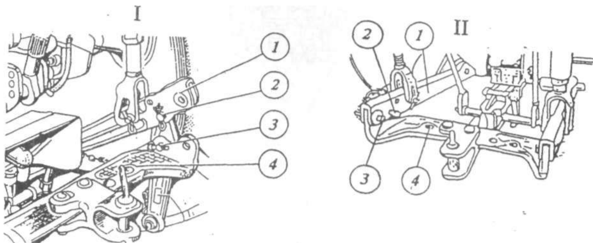
44. ábra A traktor vonóberendezése
