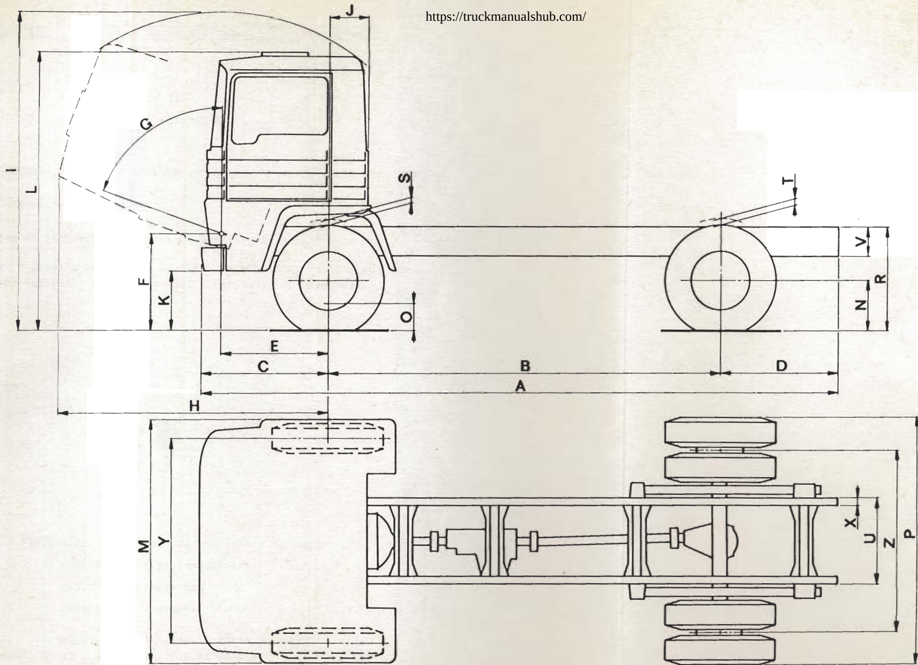
Fig.1.1 Dimensiones generales
