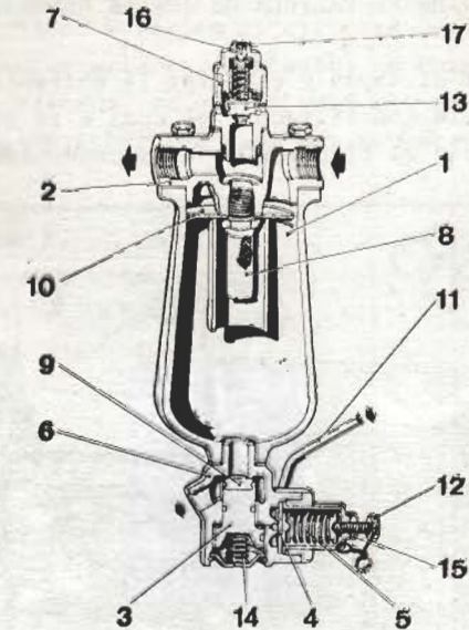
Fig.12.2 Depurador-regulador de aire.
