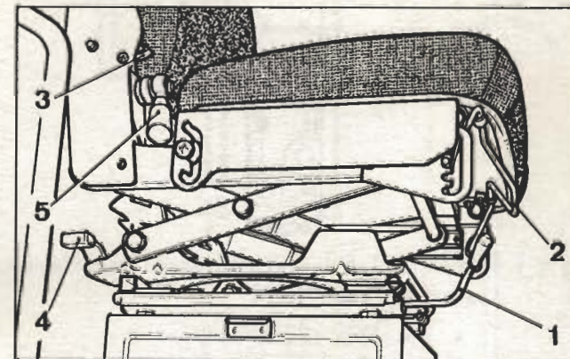
Fig.2.7 Mandos del asiento.
