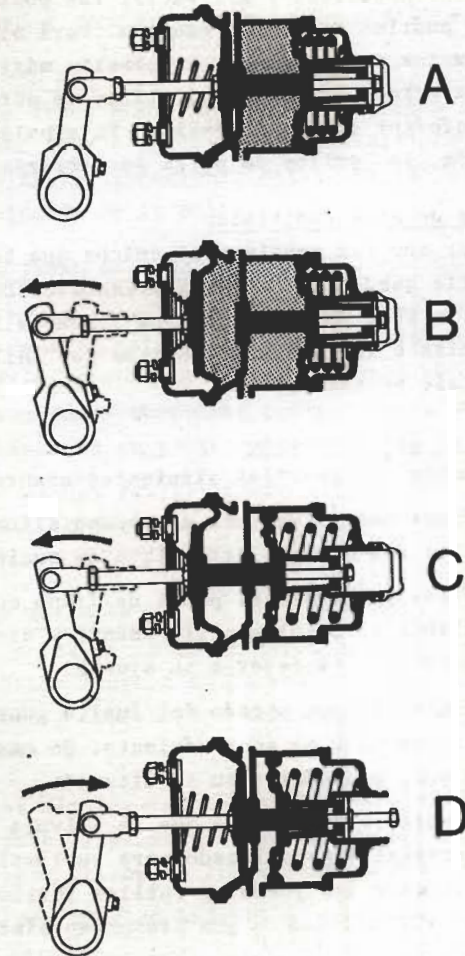
Fig.12.5 Funcionamiento de las Cámaras M.G.M.
