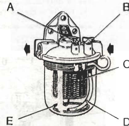
Fig. 4.2 Filtro primario de combustible.
