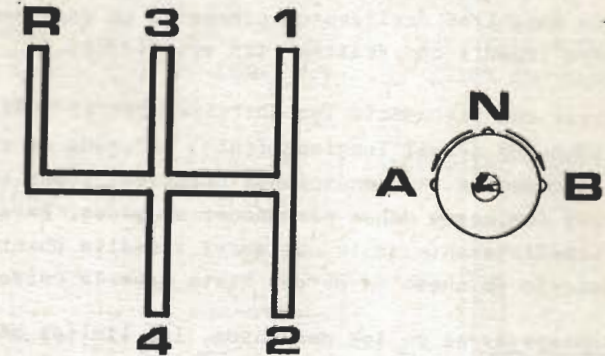
Fig.2.9 Posiciones de las velocidades y accionamiento del multiplicador.
