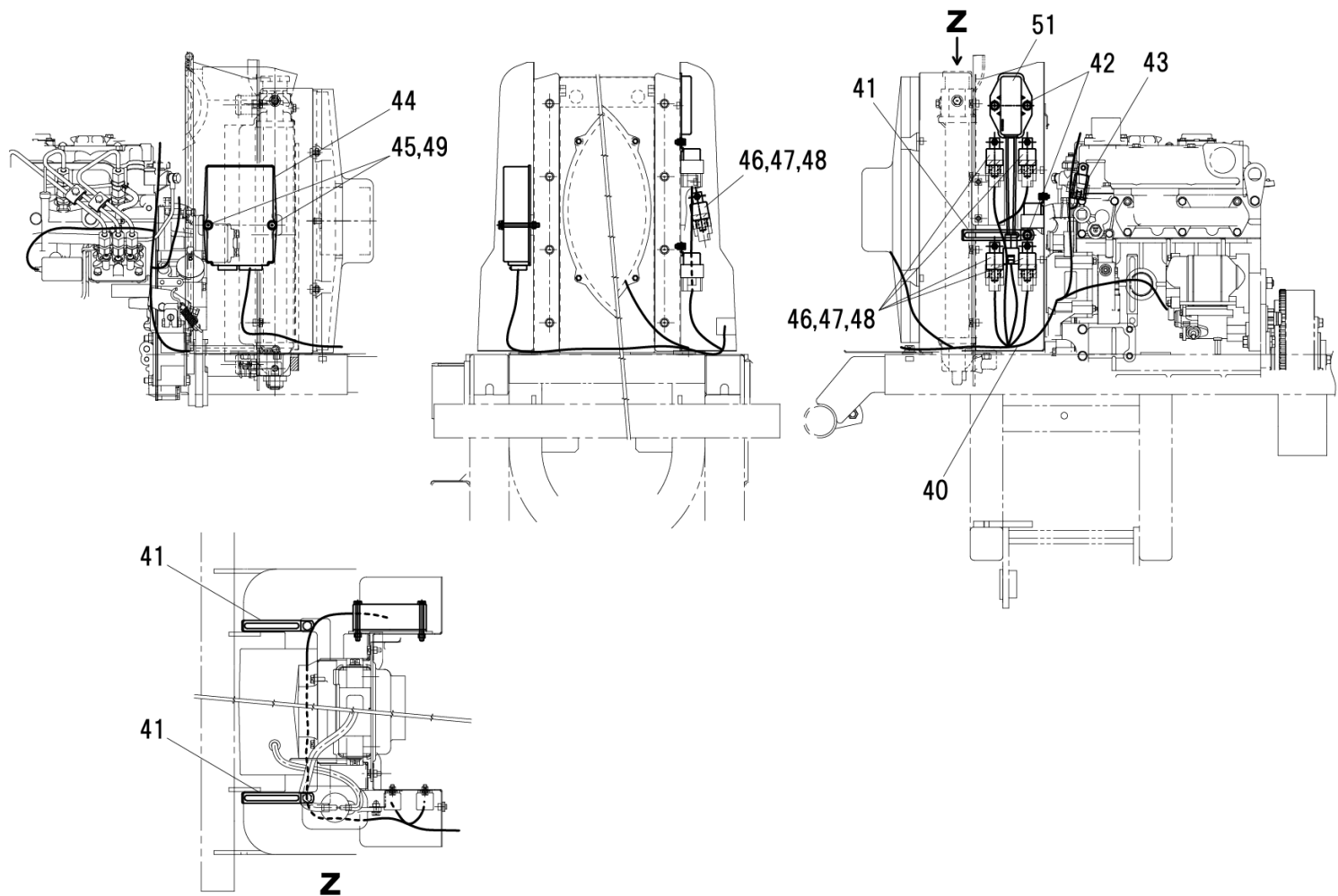
FIG.228 (2) ワイヤハーネス ; デンドウ ファン WIRE HARNESS ; FAN MOTOR
