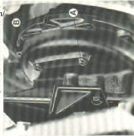
FIG. 25 - A-B: Tappi di introduzione e livello olio nei riduttori laterali posteriori.
