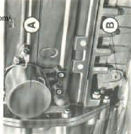
FIG. 16. A: Filtro olio motore B: Tappo scarico olio
