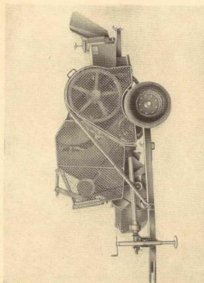
Vysokatalový zberací lis K 442/1 so sklzyým plácom pre baly
