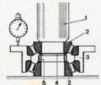
Règlage des roulements du pignon d'attaque (pont « 1500 »).
