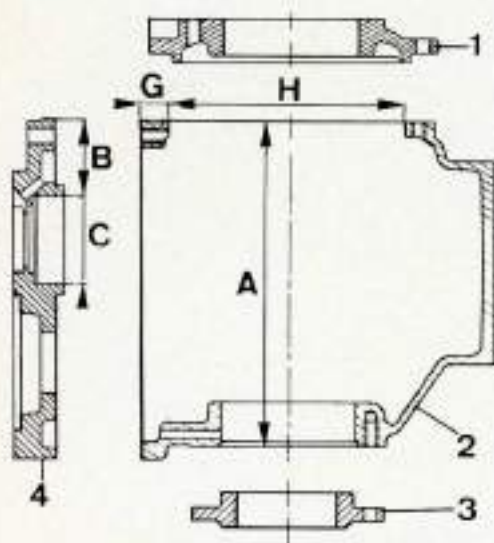
Mesures du carter de l'inverseur et de la plaque intermédiaire.
