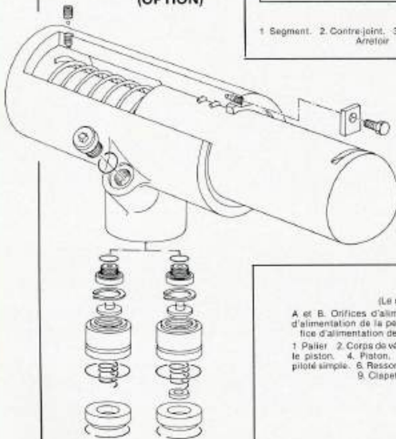
Creux d'un vérin.
