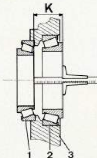
Relevé de la cote « K » pour déterminer l'épaisseur de l'entretoise des roulements à rouleaux coniques de la plaque intermédiaire.
