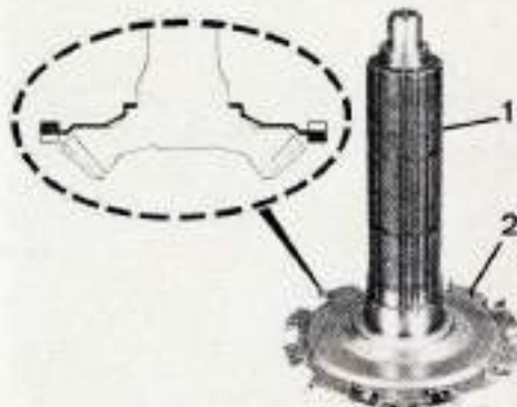
Sens de montage de la turbine sur le pignon conique de l'arbre secondaire.
