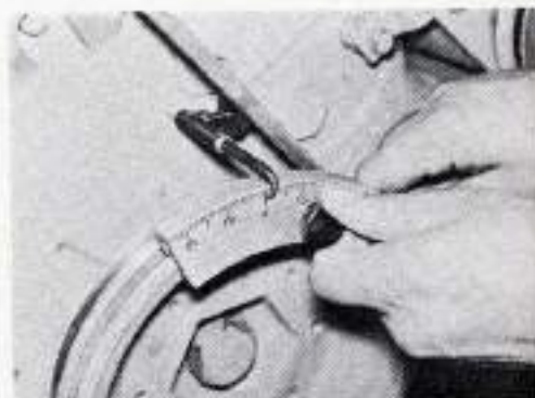
Réglage du secteur gradué.
