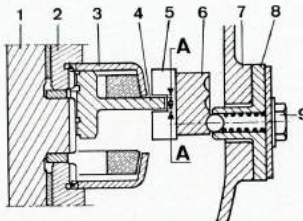
Coupe du synchroniseur de l'arbre vertical et du verrouillage de la fourchette.
