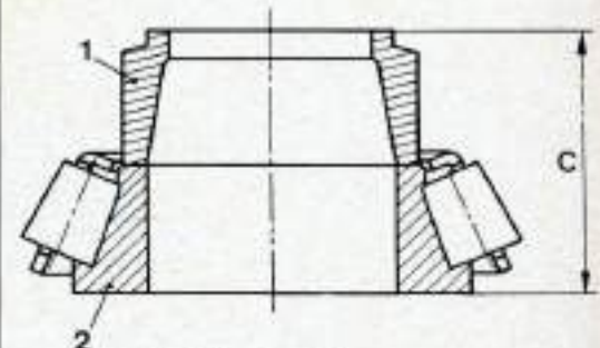
Calcul de la cote « C ».
