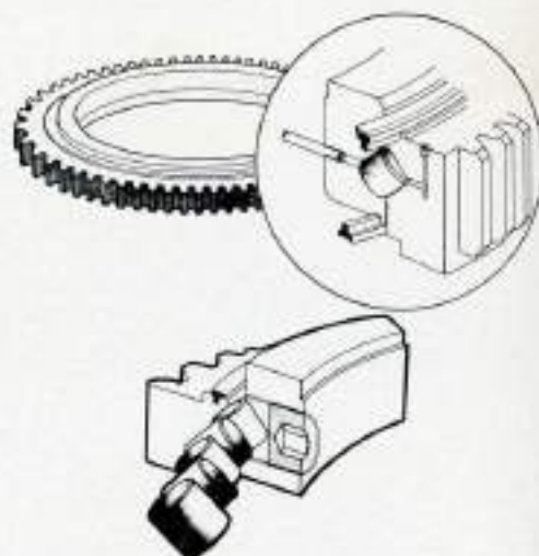
Couronne de bêche.
