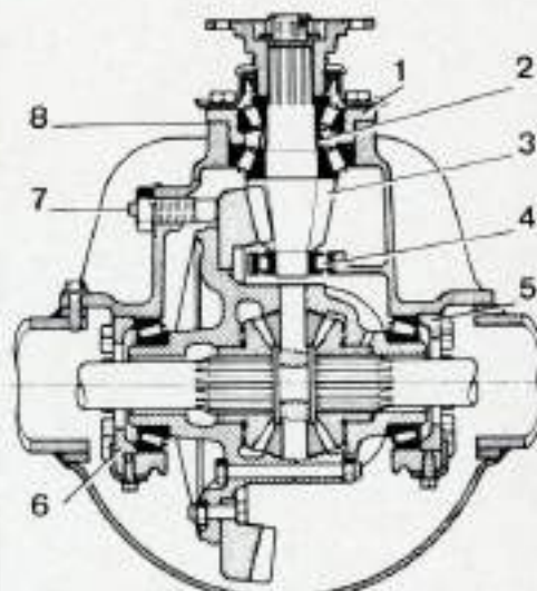
Coupe du pont « 1250 ».
