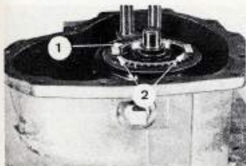
Réglage du synchroniseur de 3 e -4 e .
