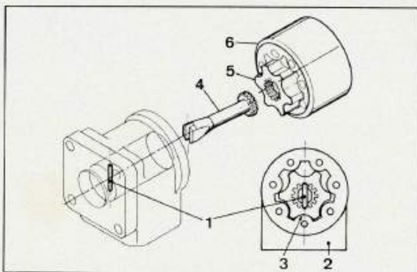
Calage du doseur.
