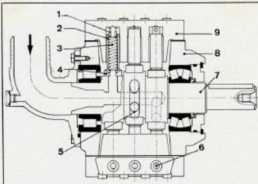
Coupe longitudinale de la pompe haute pression « PL ».
