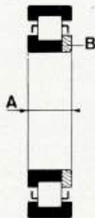
Relevé de l'épaisseur du roulement du pignon conique. A. Epaisseur du roulement. B. Rondelle d'appui.
