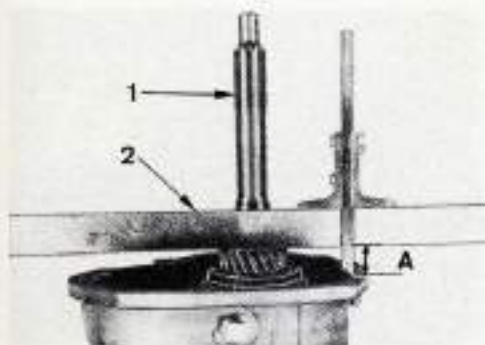
Relevé de la cote « A » pour le réglage du synchroniseur de 3 e -4 e .
