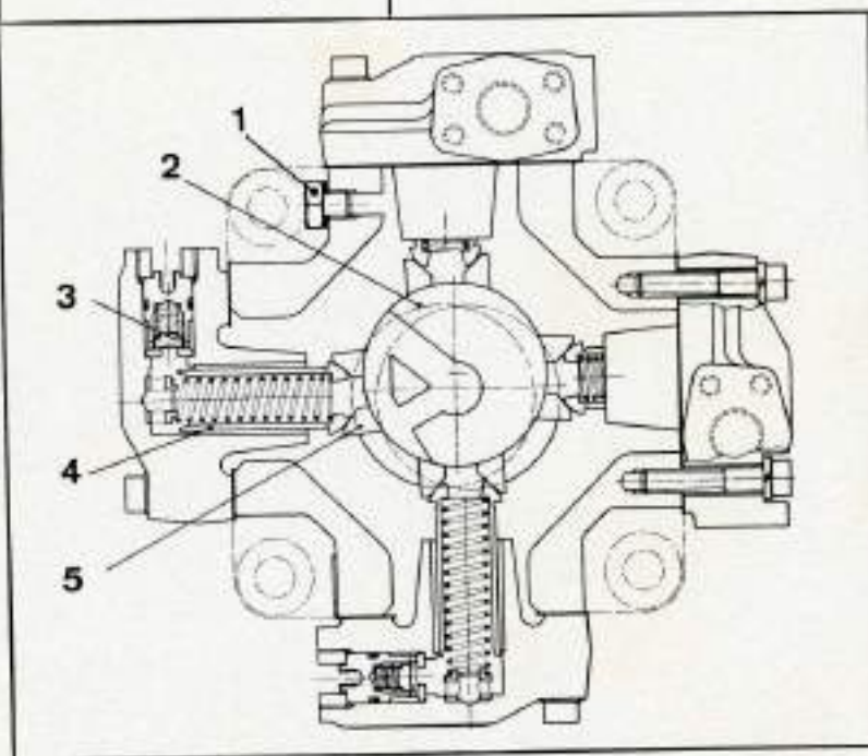
Coupe transversale de la pompe hydraulique « PL ».
