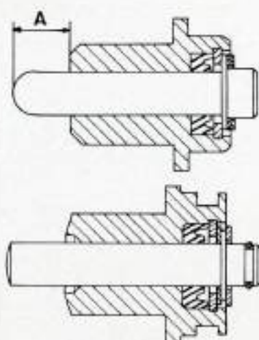
Identification des poussoirs.
