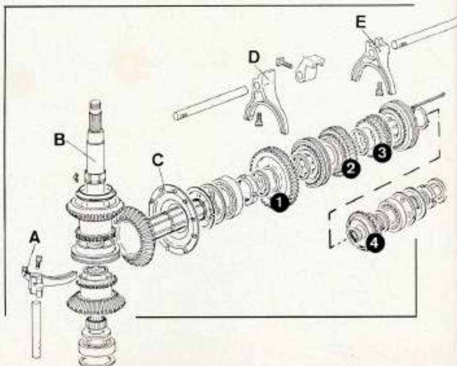
Arbres primaire, secondaire et vertical (Boîte M 27).
