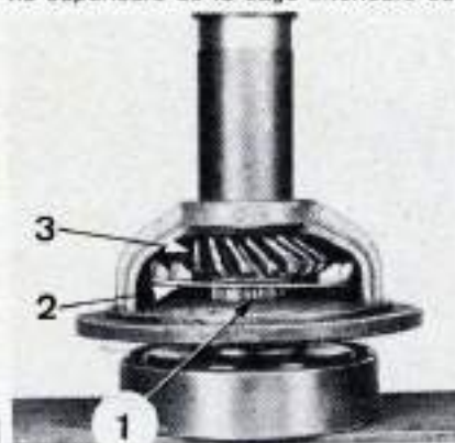
Montage du boîtier intermédiaire.
