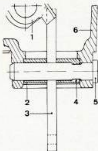
Coupe du mécanisme commandant la fourchette de l'inverseur (1 er montage).
