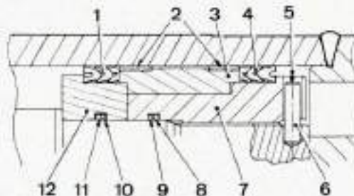
Demi-coupe d'un piston.
