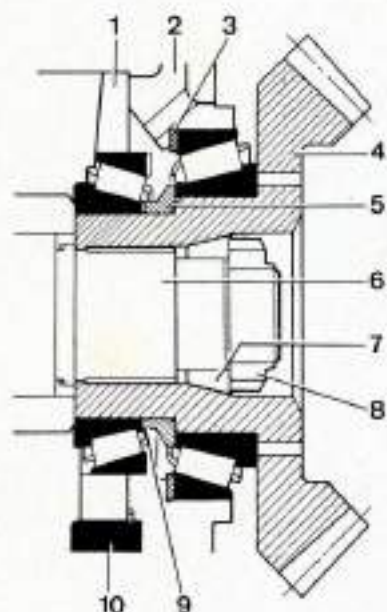
Coupe partielle de la plaque intermédiaire.
