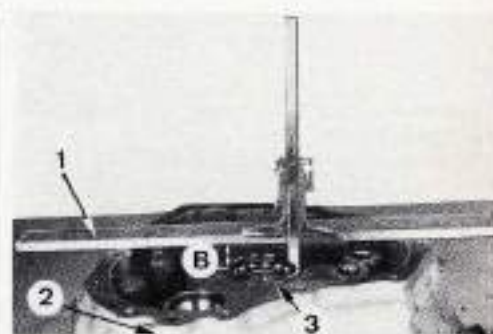
Relevé de la cote « B » pour le réglage du synchroniseur de 3 e -4 e .
