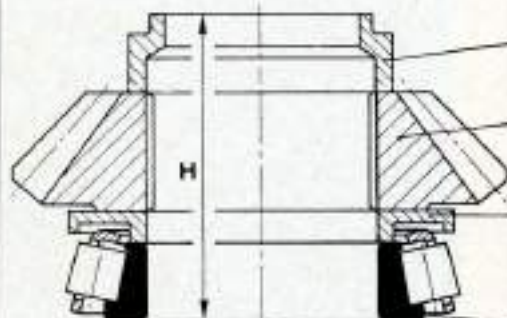
Calcul de la cote « H » (pelle 90 P).
