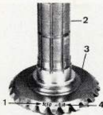
Emplacement de la valeur de la distance conique sur le pignon.
