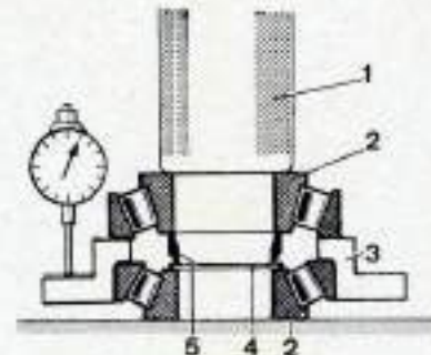
Règlage des roulements du pignon d'attaque (pont « 1250 »).
