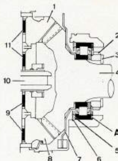
Coupe partielle de l'inverseur.
