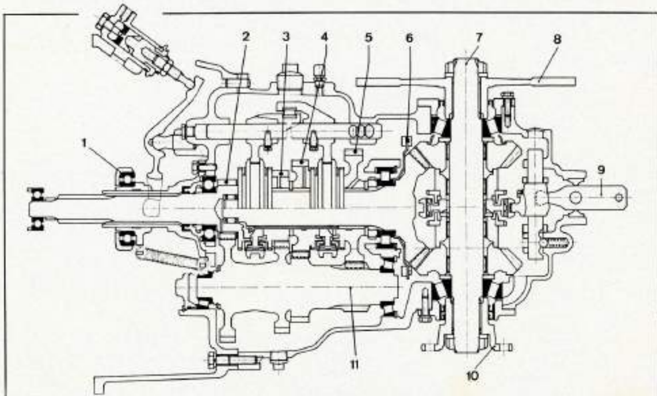
Coupe de la boîte de vitesses-inverseur type M 27 (Pelle « 75 P »).
