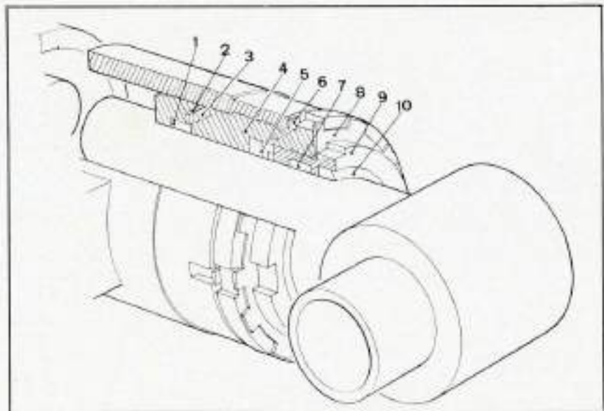
Creux d'un vérin.
