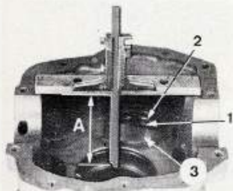
Relevé de la distance entre le fond du logement de roulement et le plan de joint du carter de boîte (côté inverseur).
