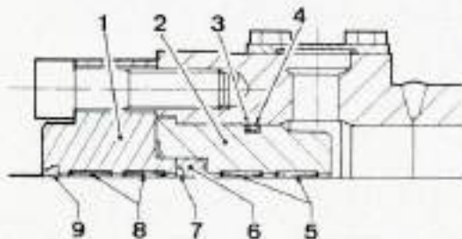
Demi-coupe d'un palier.
