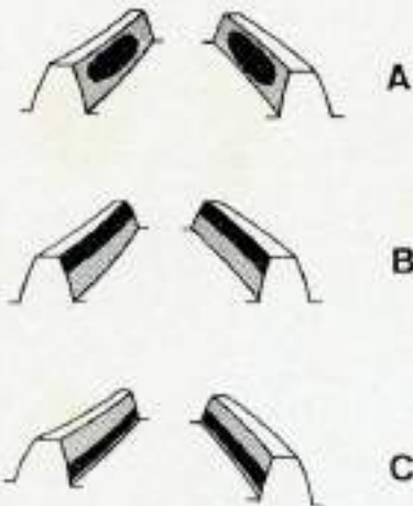
Portée de la denture de la couronne en charge.
