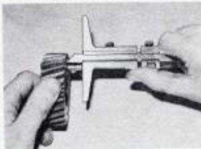
La goupille tubulaire doit dépasser de 17 mm le pignon de vilebrequin.
