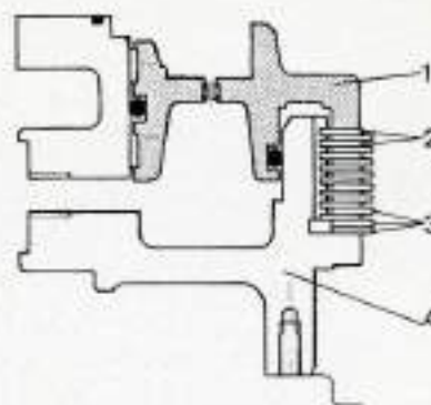
Disposition des disques dans le carter (ancien montage).
