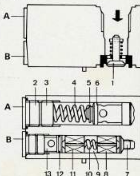
Calage du doseur.
