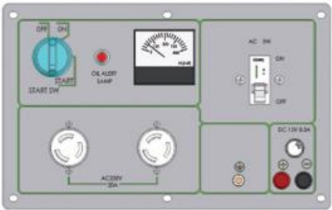
A:type-Export standard
