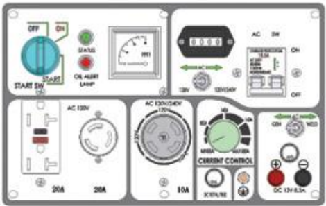
B:type-U.S.A standard
