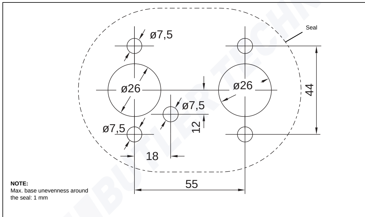
Fig. 37: Drilling template
