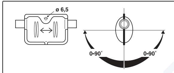
Fig. 18 Silencieux d'échappement Sens du flux (au choix)
