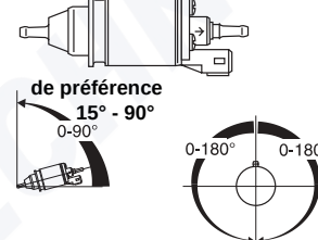
Fig. 15 Pompe de dosage DP 2 Emplacement de montage et fixation
