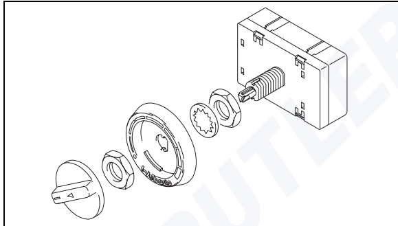
Bild 26: Bedienelement
