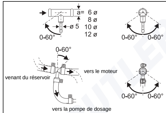
Fig. 10 Préleveur de carburant Webasto
