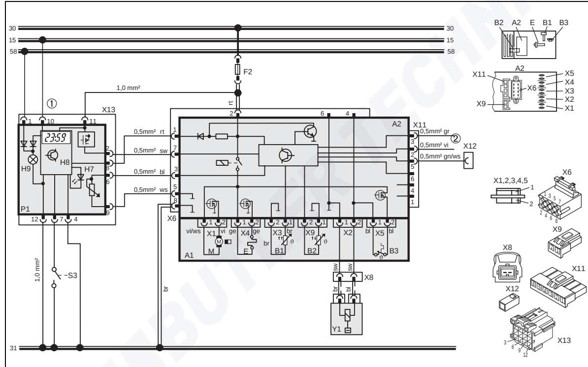
Bild 31: Automatischeschaltplan Air Top 2000, 12V/24V mit Kombiuhr, Legende siehe Seite 32 und 33
