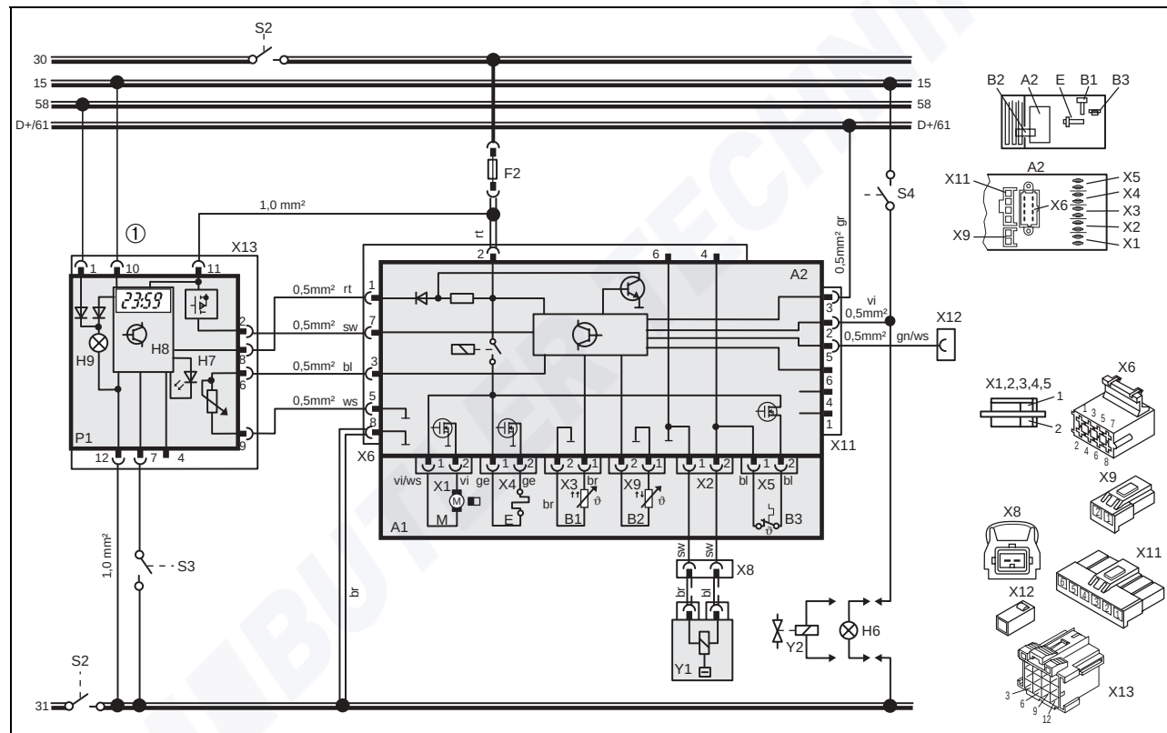
Fig. 34 Schéma électrique d'ensemble Air Top 2000, 24 V en mode ADR avec horloge polyvalente ; légende : voir pages 108 et 109
