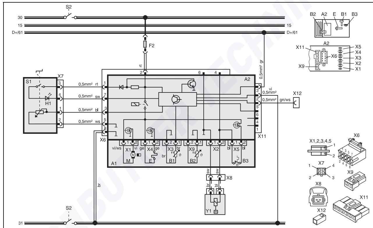
Fig. 36 Schéma électrique d'ensemble Air Top 2000 Diagnostic, 24 V en mode ADR avec organe de commande sur les véhicules ne disposant pas de commande auxiliaire ; légende : voir pages 108 et 109
