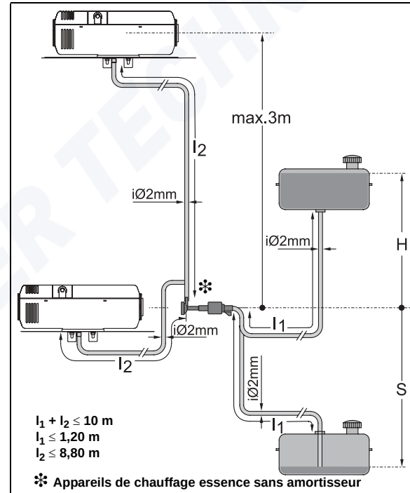
Fig. 9 Alimentation en carburant
