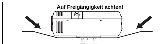
Bild 5: Einbau
