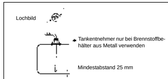
Bild 11: Webasto-Tankentnehmer
