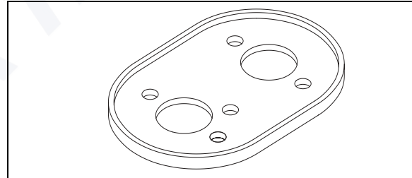
Bild 4: Dichtung
