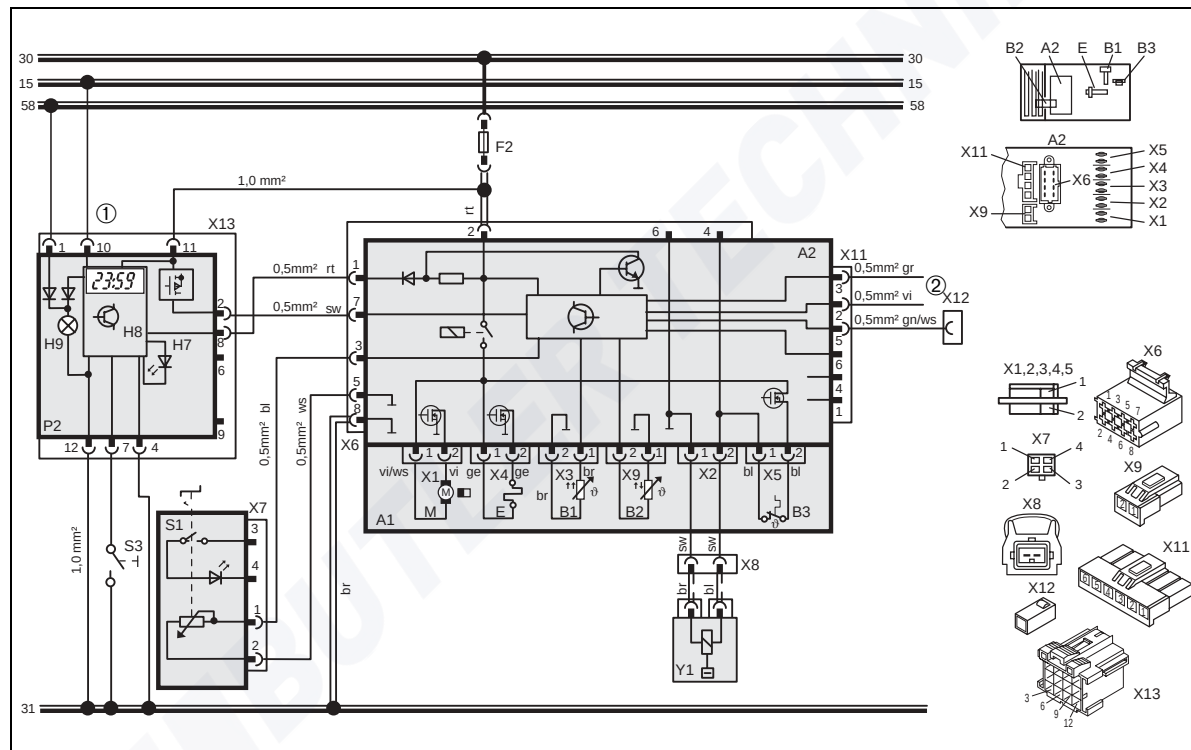
Bild 32: Automatschaltplan Air Top 2000, 12V/24V mit Bedienelement und Kombiuhr, Legende siehe Seite 32 und 33
