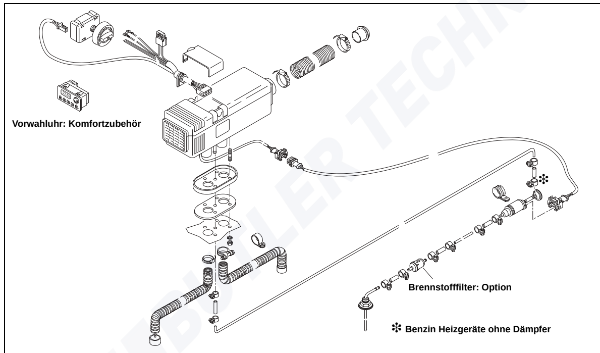
Bild 6: Einbauschema für Luftheizgerät
