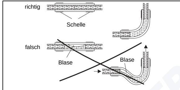
Bild 14: Rohr/Schlauchverbindung
