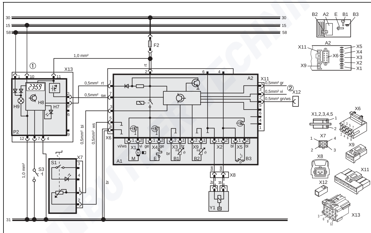
Fig. 32 Schéma électrique d'ensemble Air Top 2000, 12 V/24 V avec organe de commande et horloge polyvalente ; légende : voir pages 108 et 109
