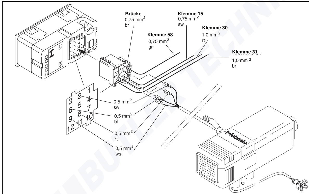
Bild 29: Anschlussschema Air Top 2000, Lieferumfang Komfort
