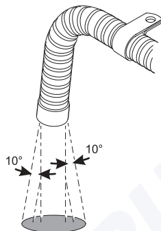
Fig. 22 Embouchure du pot d'échappement Emplacement de montage
