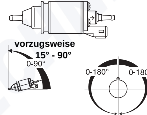
Bild 15: Dosierpumpe DP 2
