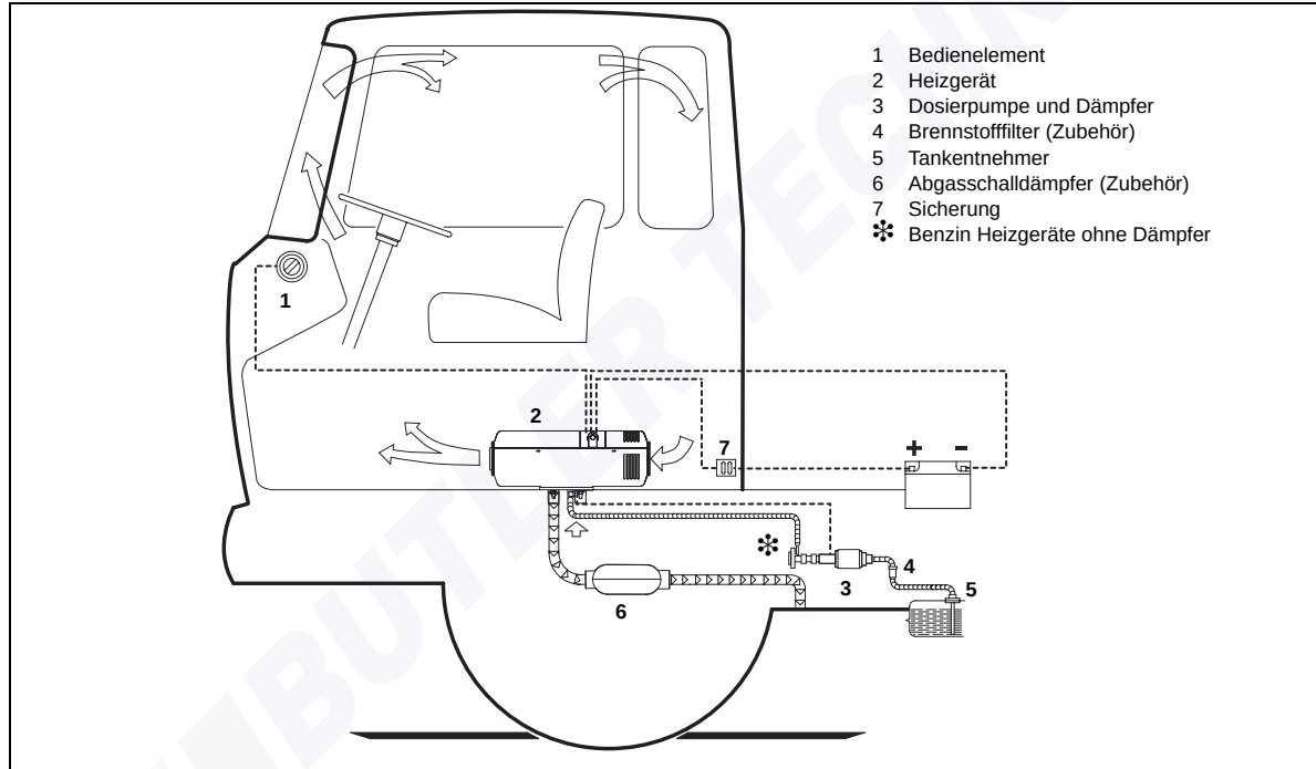
Bild 7: Einbaubeispiel für Luftheizgerät
