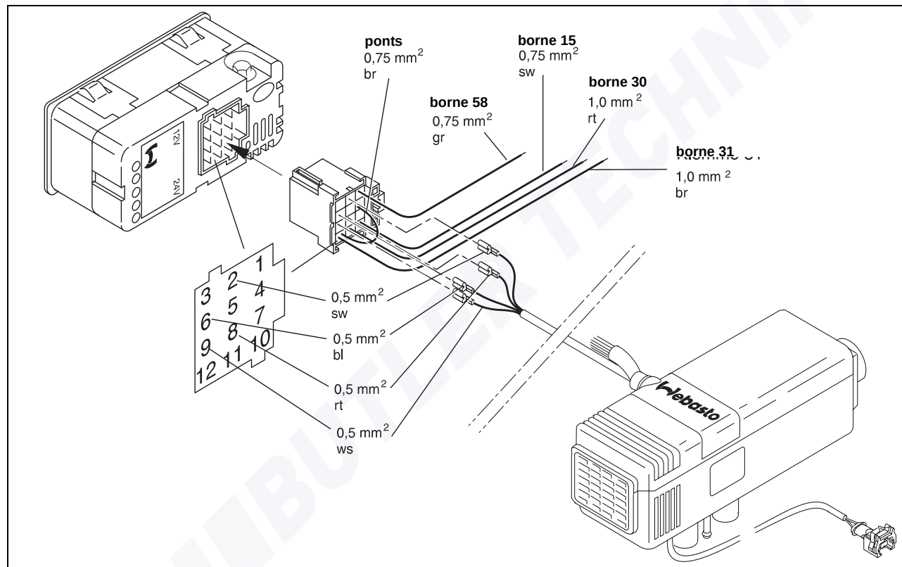
Fig. 29 Schéma de raccordement Air Top 2000, version confort
