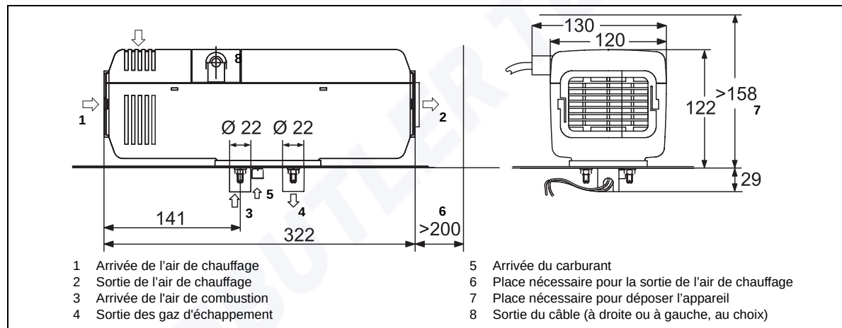
Fig. 1 Dimensions de l'appareil de chauffage
