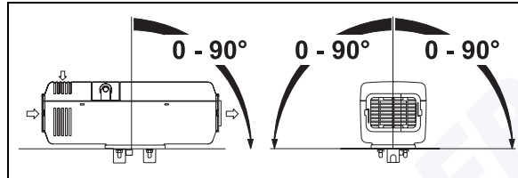
Bild 2: Empfohlene Einbaulagen Diesel Heizgeräte
