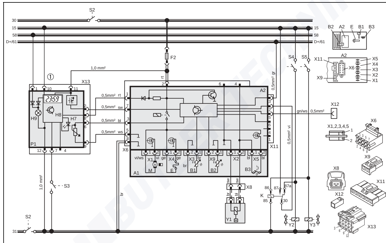
Fig. 35 Schéma électrique d'ensemble Air Top 2000, 24 V en mode ADR avec horloge polyvalente et double commande auxiliaire ; légende : voir pages 108 et 109
