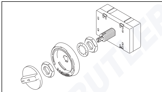
Fig. 26 Organe de commande
