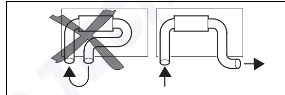
Fig. 8 Arrivée et sortie de l'air de chauffage
