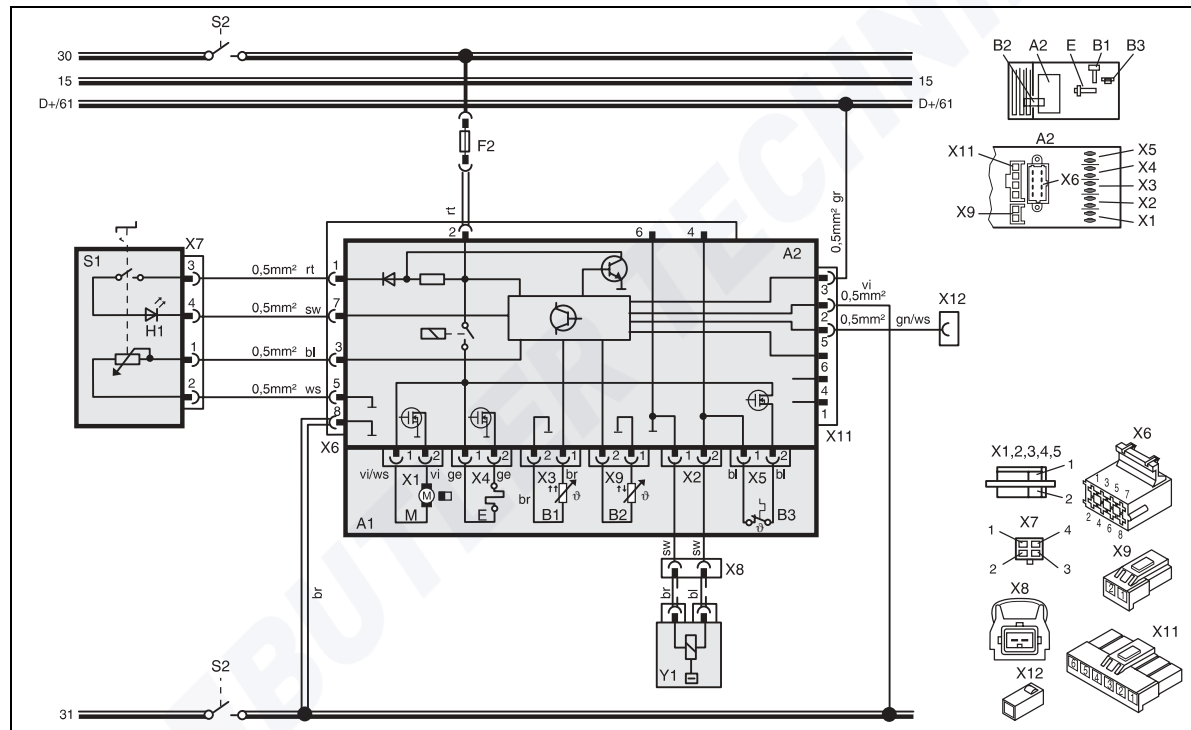
Bild 36: Automatikschaltplan Air Top 2000 Diagnose, 24V ADR-Betrieb mit Bedienelement bei Fahrzeugen ohne Nebenantrieb, Legende siehe Seite 32 und 33
