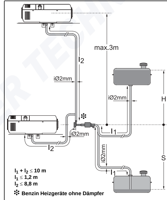
Bild 9: Brennstoffversorgung
