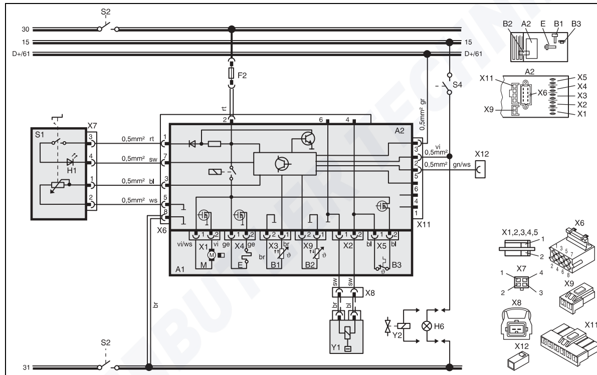
Bild 33: Automatikschaltplan Air Top 2000, 24V ADR-Betrieb mit Bedienelement, Legende siehe Seite 32 und 33
