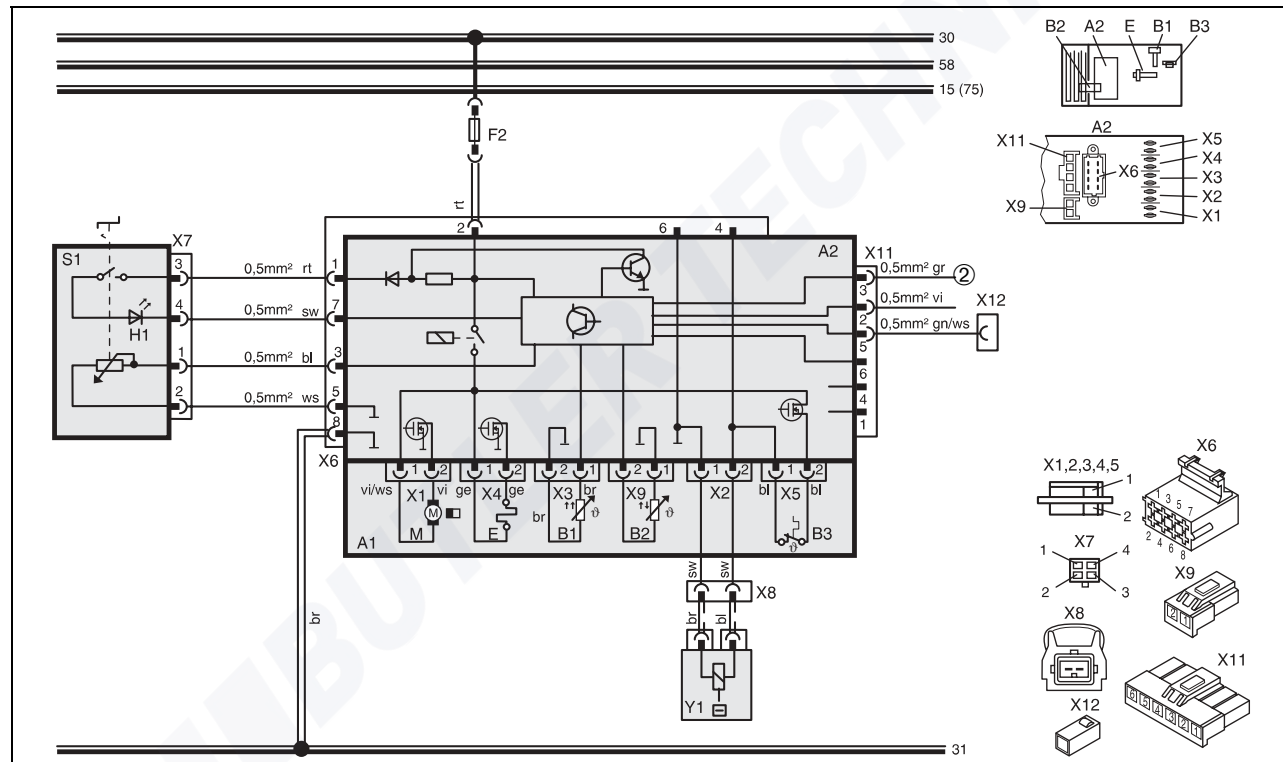
Fig. 30 Schéma électrique d'ensemble Air Top 2000, 12 V/24 V avec organe de commande ; légende : voir pages 108 et 109
