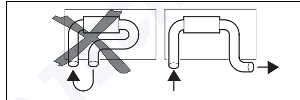
Bild 8: Heizlufteintritt und Heizluftaustritt
