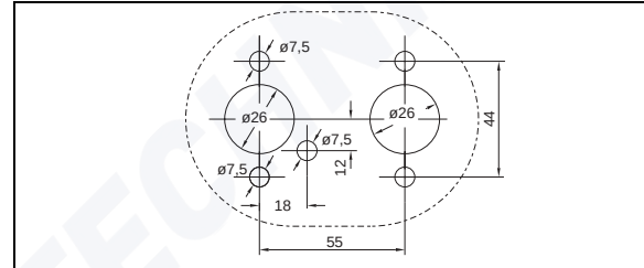
Bild 3: Lochbild
