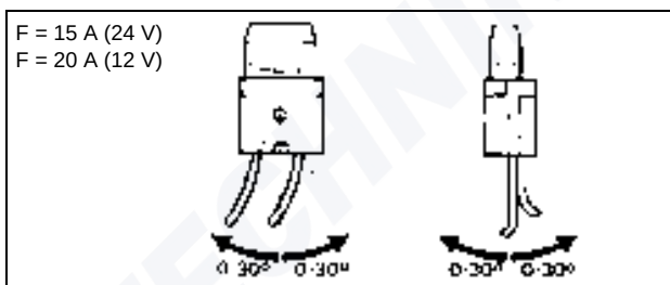
Fig. 25 Porte-fusibles, emplacement de montage
