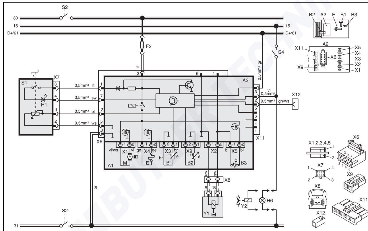
Fig. 33 Schéma électrique d'ensemble Air Top 2000, 24 V en mode ADR, avec organe de commande ; légende : voir pages 108 et 109
