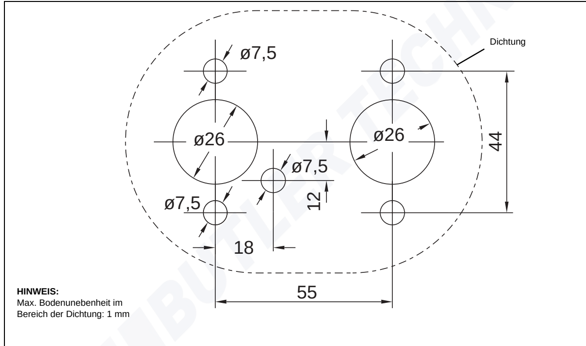
Bild 37: Bohrschablone
