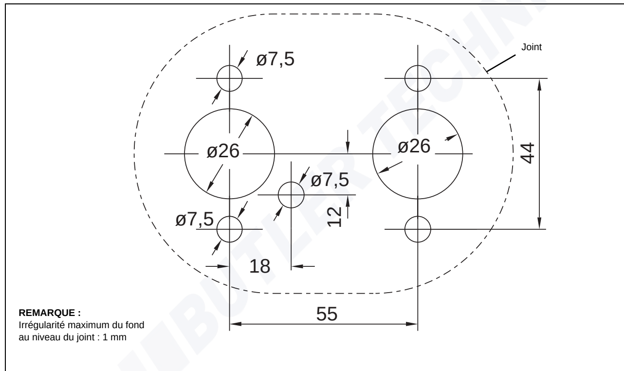
Fig. 37 Gabarit de perçage
