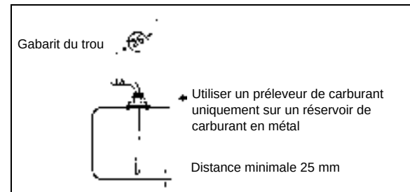
Fig. 11 Préleveur de carburant Webasto
