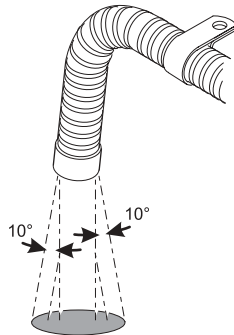
Bild 22: Abgasrohrmündung Einbaulage
