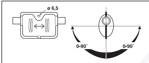
Bild 18: Abgasschalldämpfer Durchflußrichtung (beliebig)
