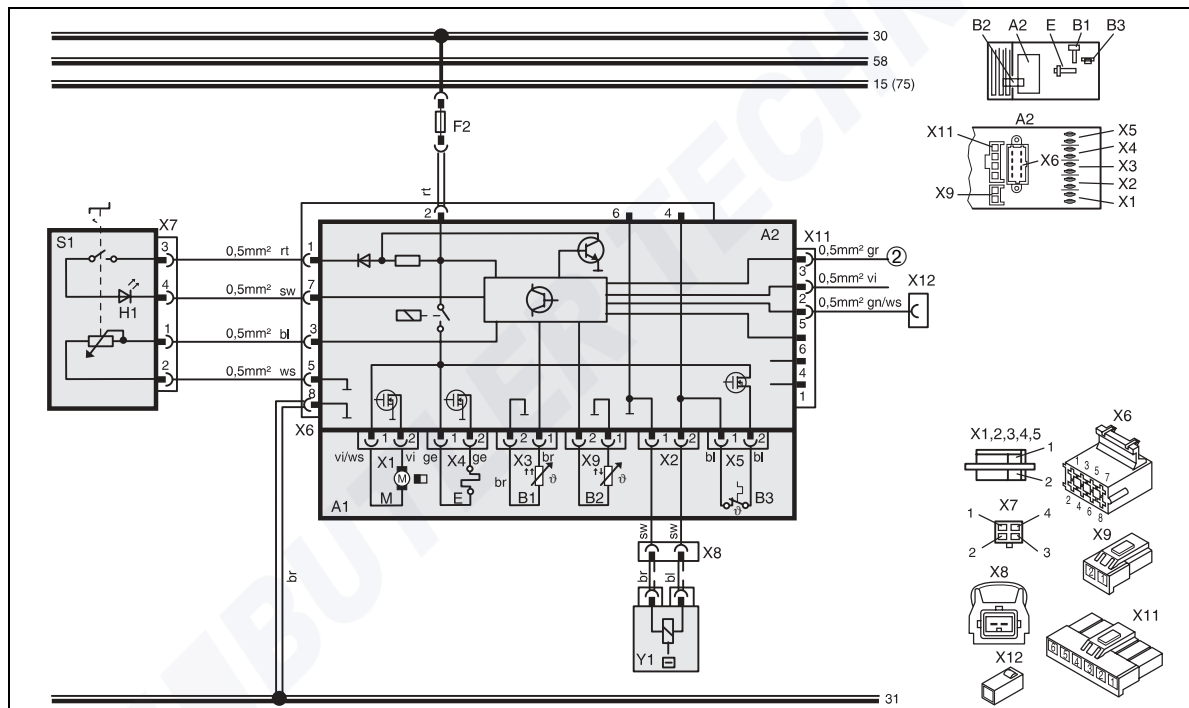
Bild 30: Automatikschaltplan Air Top 2000, 12V/24V mit Bedienelement, Legende siehe Seite 32 und 33
