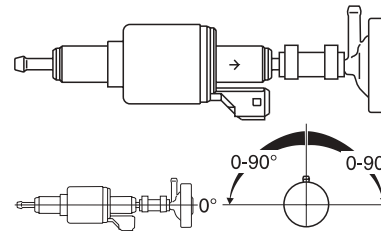
Fig. 16 Pompe de dosage DP 30 Emplacement de montage et fixation
