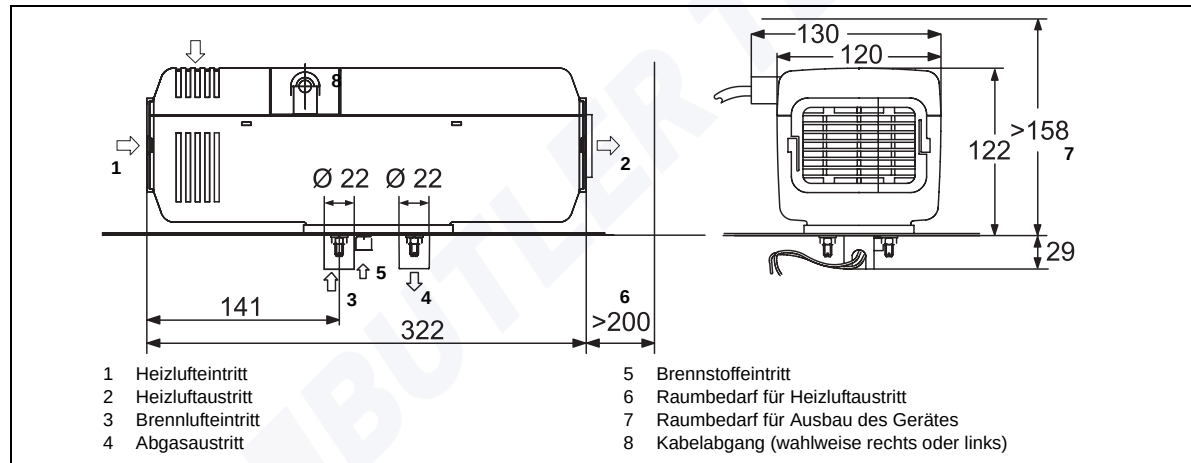
Bild 1: Abmessungen des Heizgerätes
