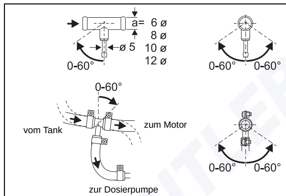
Bild 10: Webasto-Brennstoffentnehmer
