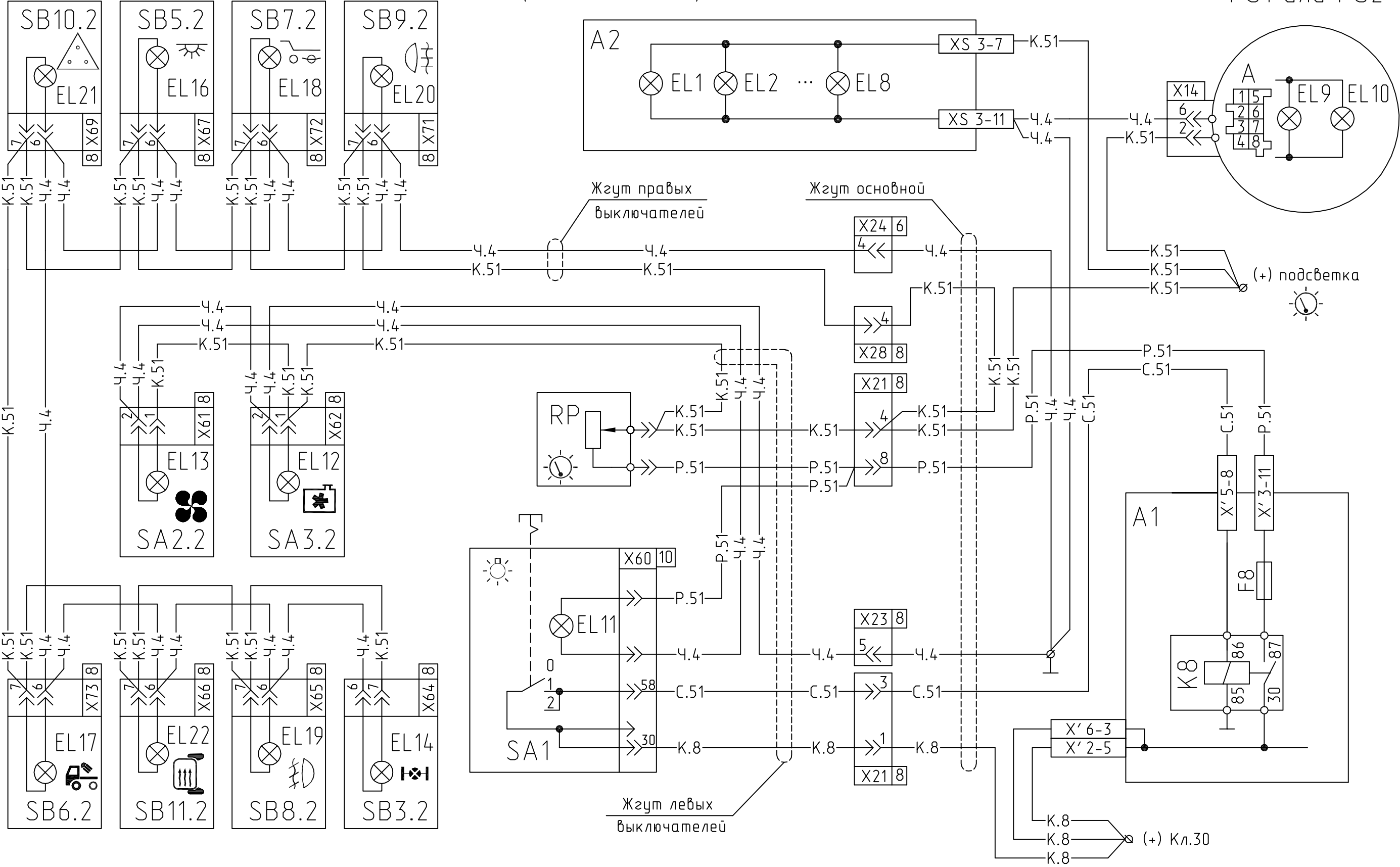
Схема включения ламп подсветки приборов и выключателей (2-х осные тягачи)
