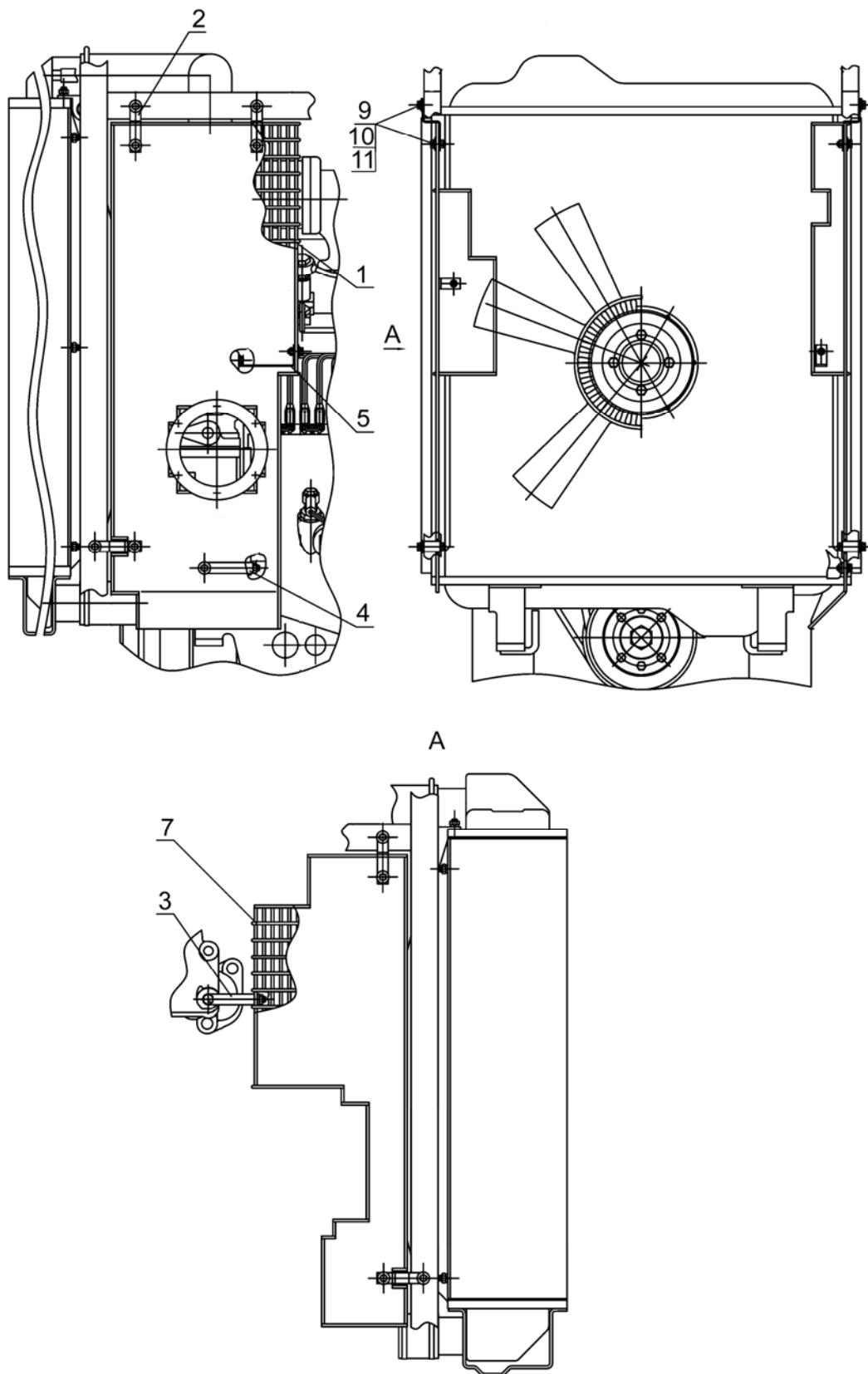
Fig. 13.2 Fan guard
