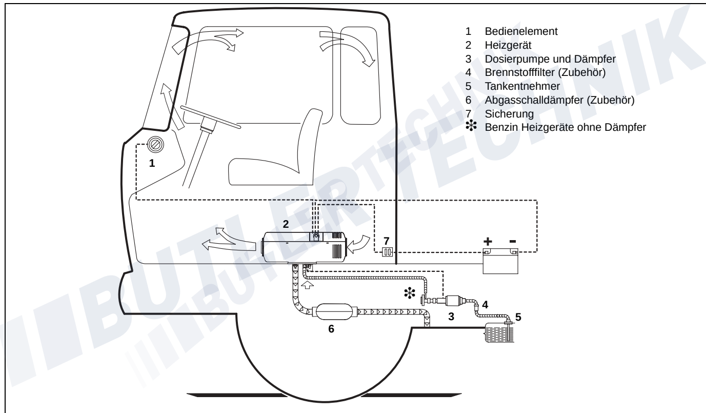
Bild 7: Einbaubeispiel für Luftheizgerät
