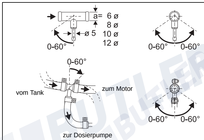
Bild 10: Webasto-Brennstoffentnehmer
