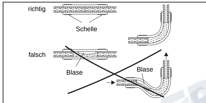
Bild 14: Rohr/Schlauchverbindung
