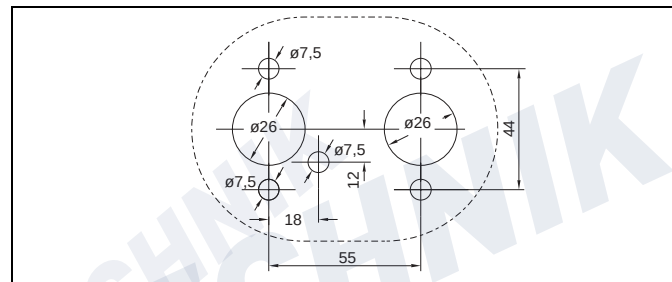
Bild 3: Lochbild
