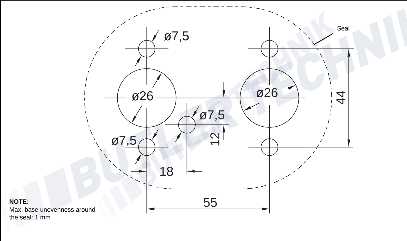
Fig. 37: Drilling template
