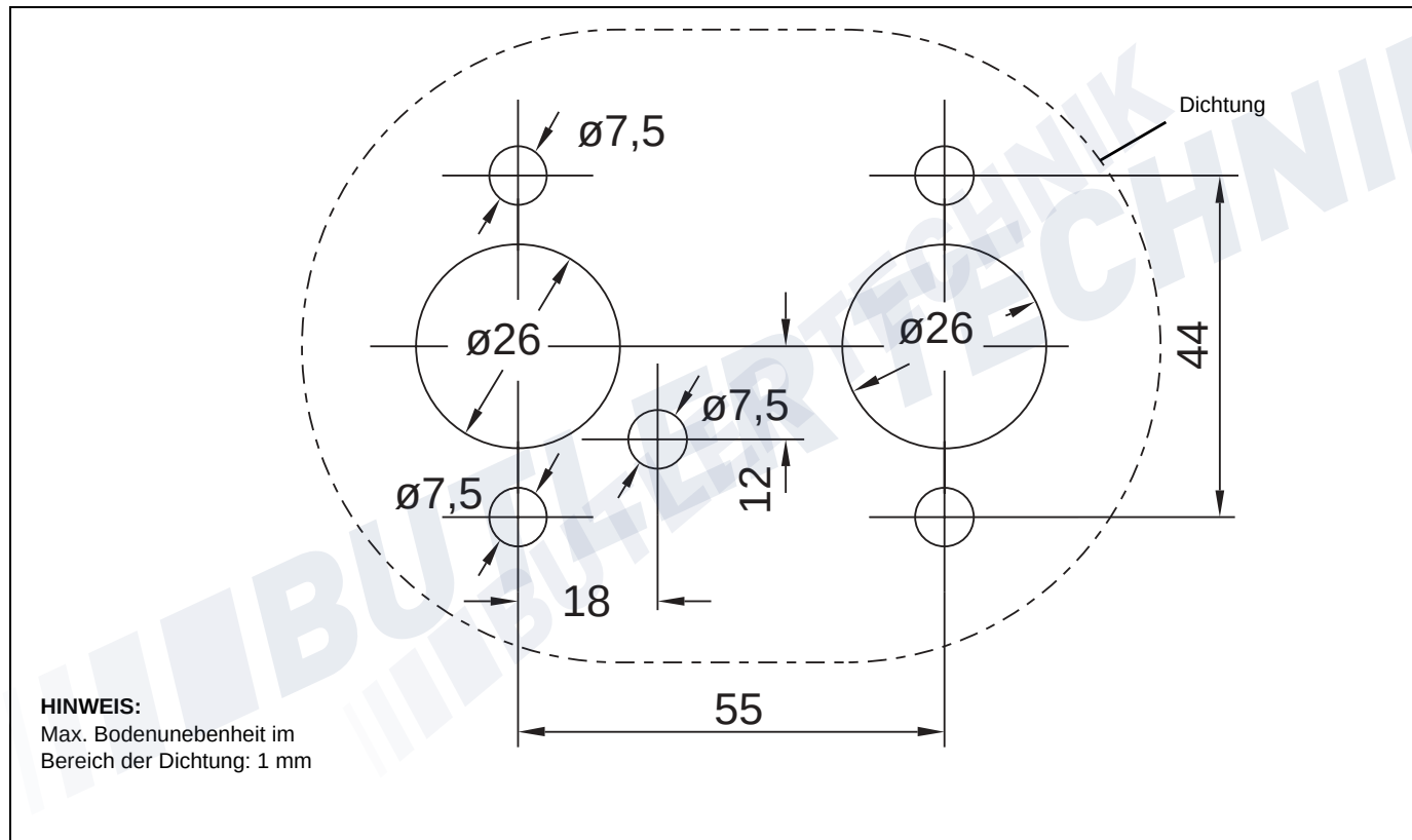
Bild 37: Bohrerschablone
