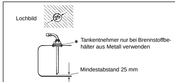
Bild 11: Webasto-Tankentnehmer
