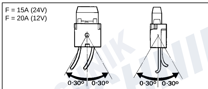
Bild 25: Sicherungshalter, Einbaulage
