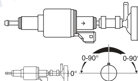
Bild 16: Dosierpumpe DP 30 Einbaulage und Befestigung
