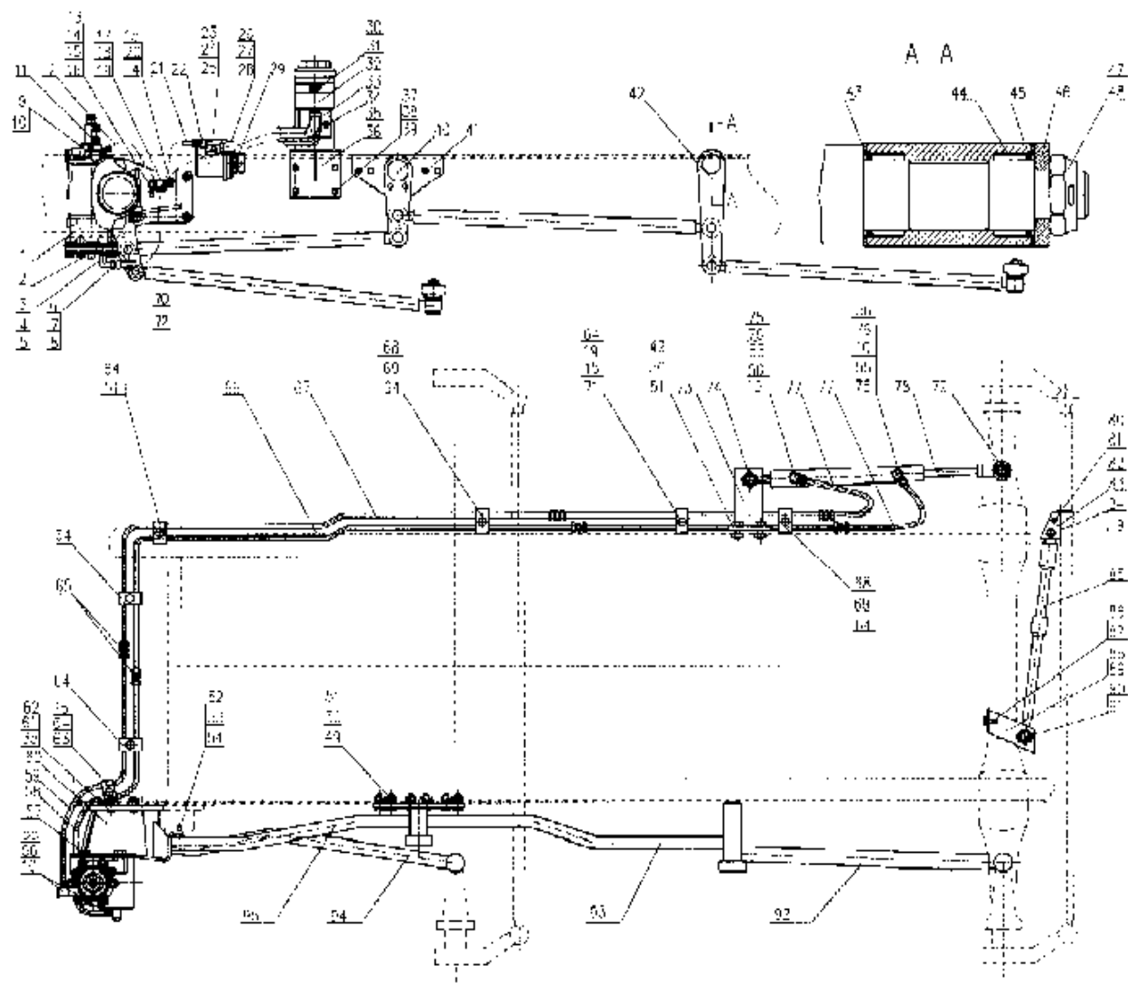
C9-4 8×4 HYDRAULIC STEERING SYSTEM/8×4液动力转向系统 Fig.C9-4
