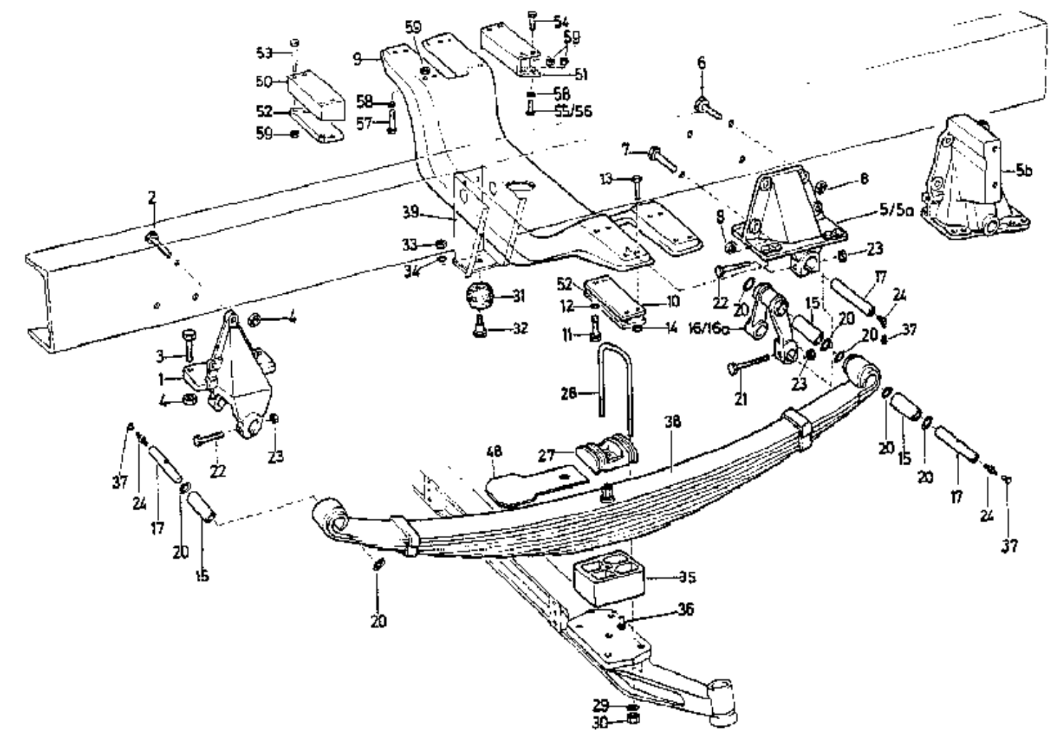
C8-1 4×2、6×2、6×4 FRONT SPRING/4×2、6×2、6×4前悬架
