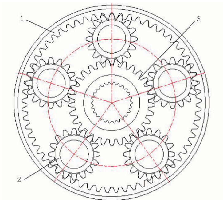
Рис. 1-7. Планетарный колесный редуктор 1 – Эпицикл; 2 – Сателлит; 3 – Солнечная шестерня
