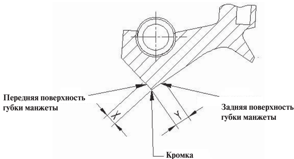
Рис. 2-5 Сечение уплотнительной манжеты
