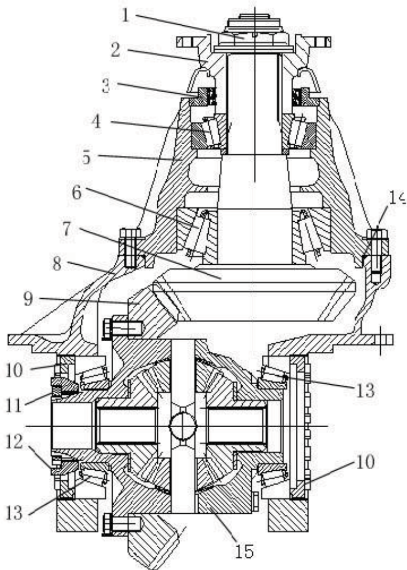
Рис. 1-4. Главная передача
