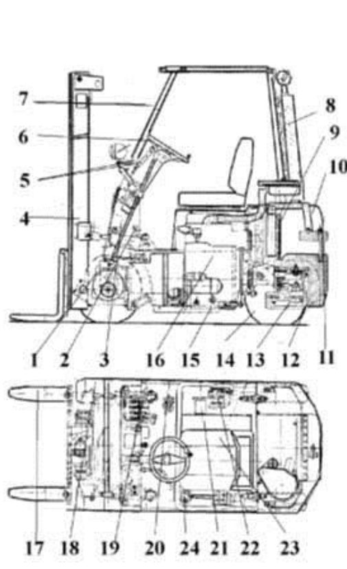
Рис. 1 Общий вид
