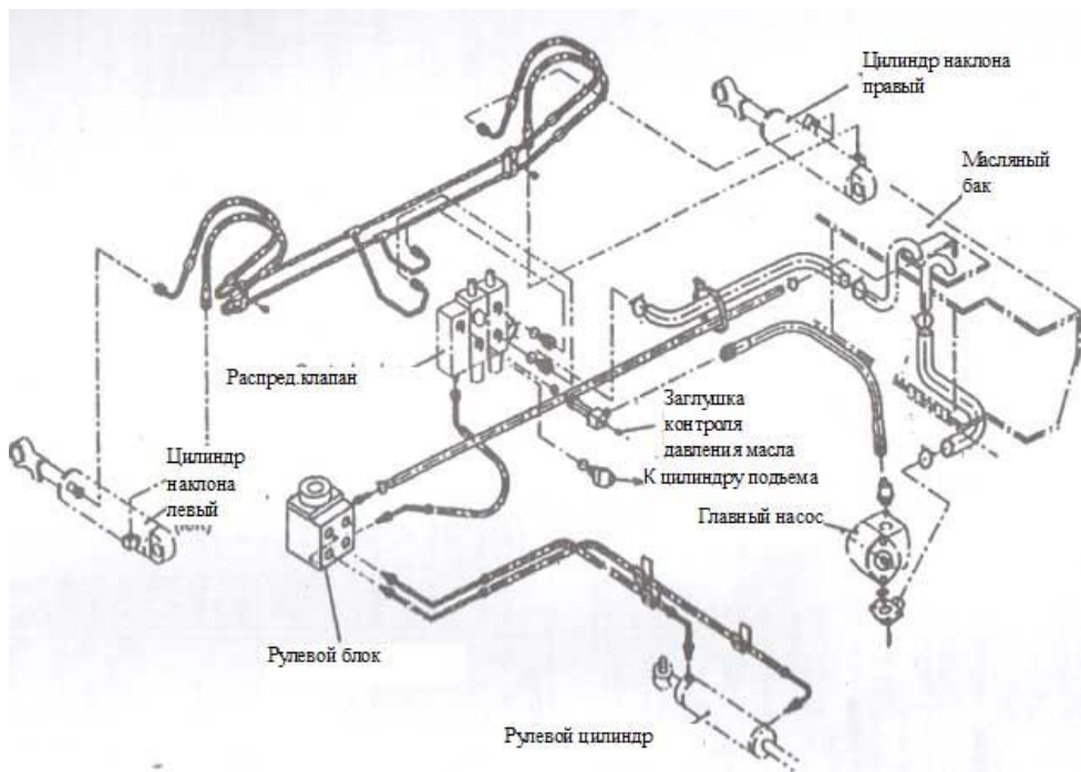
Рис. 32 Гидравлический трубопровод
